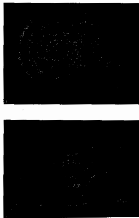
Рис. 2. Слияние изображений двух точек по мере их сближения: а — безусловное разрешение ( r = \lambda / A ); б — предельное разрешение ( r = 0,5 \lambda / A ).
