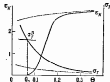
Рис. 2. Схематическое изображение зависимости от гомологической температуры \theta предельной деформации до разрушения \epsilon_k , предела текучести дислокационной пластичности \sigma_f и пластичности деформационного двойникования \sigma_d для кристаллов с ОЦК (сплошная линия) и ГЦК (штриховая линия) решётками.
