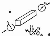
Рис. 1. Амплитудный модулятор света с поляризационной ищевой.
