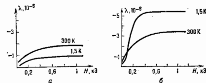
Рис. 2. Зависимость констант магнитоэлектричества Y_3Fe_5O_{12} от напряженности магнитного поля при разных температурах: а — \lambda_{100} , б — \lambda_{111} .
