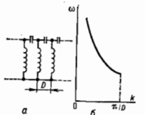
Рис. 3. Электрическая схема фильтра высоких частот (а) и дисперсионная характеристика распространяющейся в нём волны с отрицательной групповой скоростью v_g < 0 (б).
