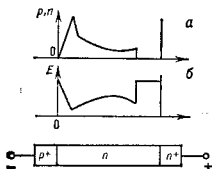
рис. 2. Распределение концентрации плазмы (а) и напряжения поля (б) при переключении диода на дрейфовой стадии накопления.
