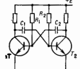
Рис. 3. Мультивибратор на биполярных транзисторах.
