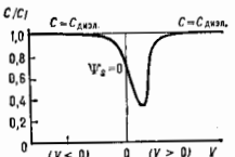
Рис. 5. Квазистатическая вольт-фарадная характеристика МДП-структуры.
