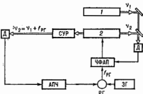
Рис. 1. Схема оптического стандарт частоты: ЧФАП — частотно-фазовый автоподстройщик; СУР — система получения сверхузкого резонанса; АПЧ — система автоматической подстройки частоты; ЗГ — звуковой генератор; РГ — радиогенератор; Д — фотодетектор.
