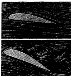
Рис. 2. Обтекание крыла: а — плановое; б — с образованием отрывного течения.
