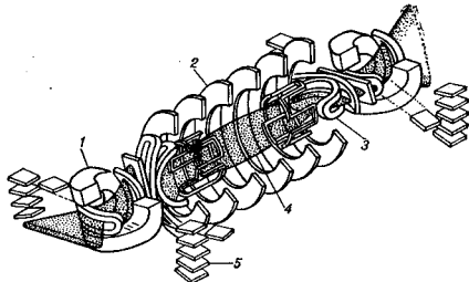
Рис. 2. Схема амбиполярной ловушки ТМХ: 1 — аксиально-несимметричные обмотки концевых пробкотронов, обеспечивающих минимум магнитного поля H на оси; 2 — обмотка центрального соленоида; 3 — переходные обмотки; 4 — плазма; 5 — инжекторы нейтральных атомов. Характерная «версная» форма плазмы вблизи концов установки обусловлена свойствами магнитного поля установки. В центральном соленоиде сечение плазмы круглое.
