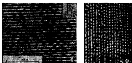
Рис. 15. Характерные периодические структуры, наблюдаемые лазерным излучением на поверхности твердых тел: а — одномерная решётка на поверхности Ge, наблюдаемая излучением неодимового лазера; б — двумерная решётка, возникающая на поверхности при увеличении интенсивности лазера.
