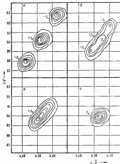
Рис. 6. Двумерные распределения интенсивности I в узле (002) кристалла — сегнетоэластика \text{K}_2\text{Fe}(\text{SO}_4)_2 при T = 52^\circ\text{C} (а); 1^\circ\text{C} (б); 4^\circ\text{C} (в); 10^\circ\text{C} (г); S_0 и S_c — компоненты узла, относящиеся к двумам двух возможных конфигураций; знаки \pm указывают на противоположную направленность спонтанной сдвиговой деформации, возникающей ниже точки фазового перехода 2-го рода.
