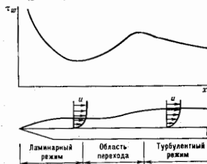
Рис. 4. Изменение режима течения в пограничном слое и поверхностного трения на плоской пластине.
