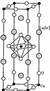
Рис. 2. Кристаллическая структура соединений \text{La}_{2-x}\text{Sr}_x\text{CuO}_4 .
