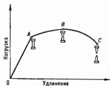
Рис. 8. Деформация при растяжении металлического цилиндра.
