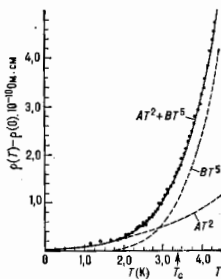
Рис. 6. Зависимость удельного сопротивления \rho от T . Точка — измеренные значения на вычитом остаточном сопротивлении 8,8 \cdot 10^{-10}\text{ Ом·см} ; сплошная линия — зависимость вида A72 + B75 , представляет сумму электрон-электронного и электрон-фононного вкладов.
