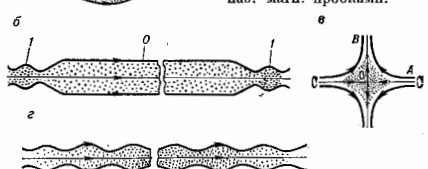
Рис. 1. Различные типы открытых магнитных ловушек (точками показана плазма): а — пробиротрон; б — амбиопланарная ловушка (О — длинный центральный пробиротрон, / — короткие концевые пробиротроны); в — антипробиротрон (О — нуль магнитного поля, А — осевая щель, В — кольцевая щель); г — многополюсная ловушка.
