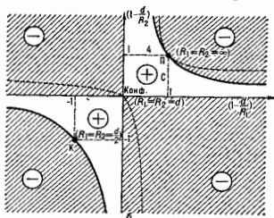
рис. 2. Образование каустики (а) и диаграмма устойчивости двухзеркальных резонаторов (б); а) аналог плюс отмечены области устойчивости; минус — области неустойчивости; сплошные линии — границы этих
