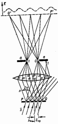
Рис. 3. Схема образования изображения несоосветящегося объекта по Аббе. Вверху — распределение освещённости в плоскости изображения; 0 , 1 — дифракционные максимумы; aa — апертура диафрагмы.
