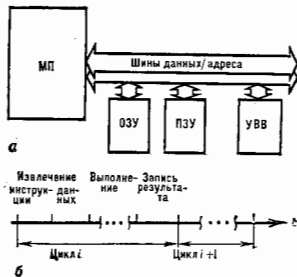
Рис. 1. Архитектура (а) и временная диаграмма шин инструкций (б) однокристального микропроцессора.
