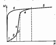
Кривая начального намагничивания (а) и безгистерезисная кривая намагничивания (б).
