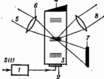
Рис. 9. Схема акустооптического модулятора света на бегущей волне: S(t) — модулирующий сигнал; 1 — генератор электрических колебаний; 2 — пьезопреобразователь; 3 — звукопровод; 4 — поглотитель; 5 — световой пучок; 6 — линза; 7 — экран; 8 — боковой дифракционный максимум.
