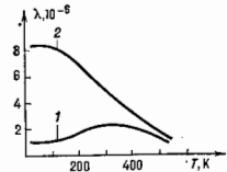
Рис. 1. Температурная зависимость констант магнитоэлектричества для Y_3Fe_5O_{12} : 1 — \lambda_{100} , 2 — \lambda_{111} .
