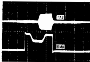
Рис. 3. Осциллограмма импульса поверхностной магнитоакустической волны, рассеянной на поверхностных акустических волнах. Амплитуда проходящего после рассеяния импульса поверхностной магнитоакустической волны (испытывающего брэгговское отражение) уменьшается (провал в середине осциллограммы импульса поверхностной магнитоакустической волны).
