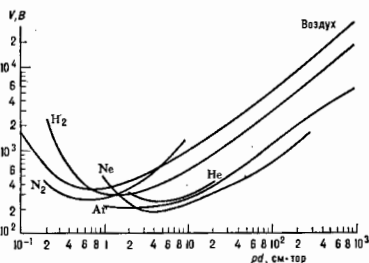
Рис. 1. Зависимости потенциалов зажигания от p \cdot d (кривые Пашена) для различных газов.
