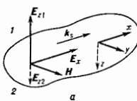
Рис. 1. Поверхностные оптические волны: а — ориентация электрических и магнитных векторов в поверхностной оптической волне, бегущей вдоль поверхности в направлении оси x ; б — распределение полей в поверхностной оптической волне в плоскости, перпендикулярной направлению распространения. 1 — для компонент E_z и H_x = H , изменяющихся при z < 0 непрерывно; 2 — для компоненты E_z , исчезающей при z > 0 скачком.
