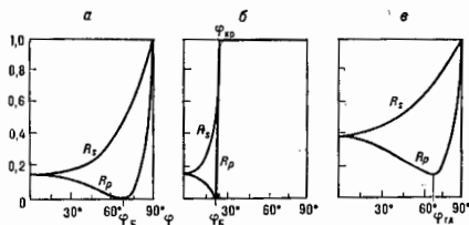
Рис. 2. Зависимость энергетических коэффициентов отражения R_s и R_p от угла падения \varphi для прозрачных диэлектриков: а) n_1 < n_2 (воздух — алмаз); б) n_1 > n_2 (алмаз — воздух); в) поглощающей среды (платина, n_2 = 2,00 , \kappa_2 = 2,03 ).
