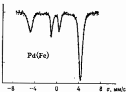
Рис. 10. Спектр испускания \gamma -квантов с E = 14,4 эВ ядер ^{57}\text{Fe} , образующихся при распаде ^{57}\text{Co} , внедрённого в Pd (концентрация \sim 10^{-4}\% ), при T = 0,025 К в поле H = 500 Э, параллельном направлению \gamma -квантов.
