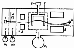
Рис. 4. Схема установки для исследования пучков в радиодиапазоне СВЧ: 1 — источник пучка; 2 — камера источника; 3 — буферная камера; 4 — прерыватель пучка; 5 — камера взаимодействия; 6 — генератор СВЧ; 7 — П-образный резонатор. Н 1 — форвакуумный насос, Н 2 и Н 3 — высоковакуумные насосы.
