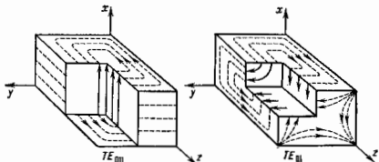
Рис. 2. Проеитные колебания (моды) TE -типа в прямоуг. объёмном резонаторе. Распределение электрических (сплошные линии) и магнитных (пунктир) полей.
