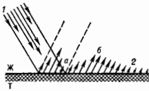
Рис. 9. Отражение звукового пучка конусного сечения, падающего из жидкости Ж на поверхность твердого тела Т под углом Разлеса: 1 — падающий пучок; 2 — отраженный пучок; а — область нулевой амплитуды; б — область хвоста пучка.
