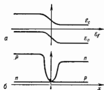
Рис. 2. Зонная диаграмма (а) и концентрация электронов и дырок (б) в области p - n -перехода; \mathcal{E}_F — дно зоны проводимости, \mathcal{E}_V — верхняя валентной зоны; \mathcal{E}_F — уровень Ферми.
