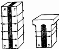
Рис. 2. Ферритовые преобразователи с установленными в монолитный сердечник постоянными магнитами (зачернены).
