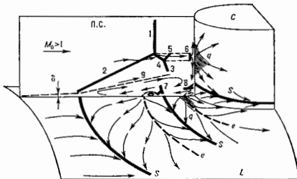
Рис. 4. Схема трёхмерного отрывного течения: L — поверхность летательного аппарата; C — цилиндрический выступ, П. с. — плоскость симметрии; \delta — толщина пограничного слоя; 1 — ударная волна; 2 — граница области отрывного течения; 3 — линии отрыва течения от поверхности летательного аппарата; 4 — линии растекания; 5 — зоны возмущённых тепловых потоков (заштрихованы).
