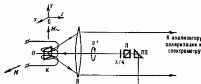
Рис. 2. Схема эксперимента по наблюдению оптической ориентации спинов методом поляризованной люминесценции; O — образец, K — линза, создающая переменное магнитное поле H_z для наблюдения резонансов, \lambda/4 — четверть-волновая фазовая пластинка, \Pi — поляризатор, \Pi\Pi — поворотная призма.
