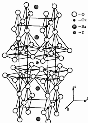
Рис. 3. Кристаллическая структура соединений \text{YBa}_2\text{Cu}_3\text{O}_x .
