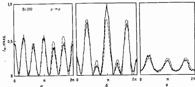
Рис. 8. Нелинейнооптическая диагностика поверхности монокристалла Si: а — интенсивность 2-й гармоники, отраженной от совершенного кристалла в зависимости от угла поворота \theta ; б, в — то же в имплантированном Si при разных дозах имплантации D = 1,2 \cdot 10^{16} \text{ см}^{-2} (б), 2,4 \cdot 10^{16} \text{ см}^{-2} (в).
