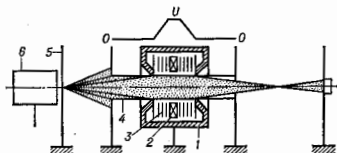
Рис. 3. Схема экспериментальной плазменной линзы для фокусирования ионного пучка: 1 — магнетрон; 2 — катушка магнитного поля; 3 — электрод-фиксатор; 4 — цилиндр — источник вторичных электронов; 5 — диафрагма; 6 — ионный источник.
