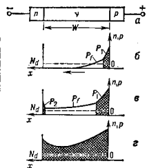
рис. 1. рун-диод: а — рун-структура; б — формирование плазменного слоя P_1 и концентрационной волны P_2 на начальной стадии включения; в — формирование слоя P_2 ; г — квазистационарное распределение плазмы после снятия диффузионных слоев.
