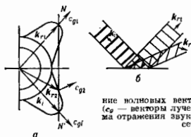
Рис. 4. Отражение акустической волны, падающей на свободную поверхность кристалла с образованием двух отраженных волн той же поляризации: а — определение волновых векторов отраженных волн ( c_i — векторы лучевой скорости); б — схема отражения звуковых пучков конечного сечения.
