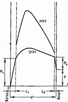
Распределение потенциала и концентрации плазмы в межэлектродном промежутке низковольтной дуги.
