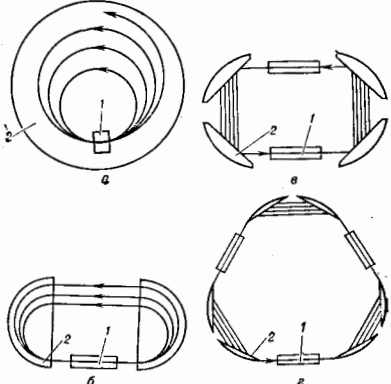
Схематическое изображение алектронных рециркуляторов, основанных на микротронном принципе ускорения: а — классический микротрон; б — разрезной микротрон; в — двухсторонний микротрон, или квадруплон; г — секстактрон; 1 — ускоряющий элемент; 8 — магнитный диполь.
