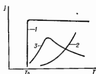
Рис. 2. Зависимости J(T) при \alpha > 1 : \gamma = 1 (1), \gamma возрастает с увеличением T (2), \gamma уменьшается с увеличением T (3).
