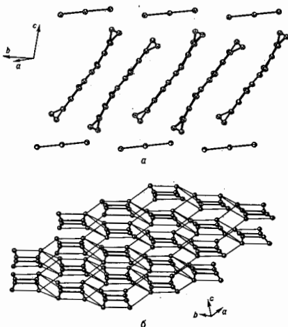
Рис. 5. Кристаллическая структура B(BEDT - TTF)_2I_3 : а — вид вдоль слоёв; б — сетка атомов S в слое BEDT - TTF (остальные атомы не показаны), по которой движутся \pi -электроны. Тонкими линиями показаны расстояния S — S между молекулами, которые меньше ван-дер-ваальсовых расстояний.
