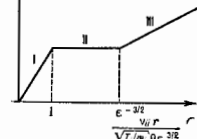
Рис. 3. Зависимость неоклассической ионной температуропроводности от частоты столкновений в токамаке: I — режим редких столкновений («банановый»); II — режим плаз.; III — гидродинамический режим.
