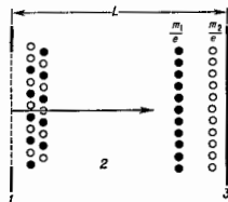
Рис. 5. Схема время-продольного масс-спектрометра. Пакет ионов с массами m_1 и m_2 (чёрные и белые кружки) движется в дрейфовом пространстве анализатора так, что тяжёлые ионы ( m_2 ) отстают от лёгких ( m_1 ).
