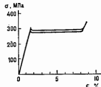
Рис. 2. Диаграмма растяжения монокристалла из сплава \text{Cu} - \text{Al} - \text{Ni} при комнатной температуре. Ориентировка осн. растяжения (100) \beta_1 ; M_s = 100^\circ \text{C} .
