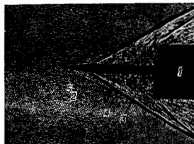
Рис. 3. Образование отрывного течения при сверхзвуковом обтекании затупленного тела 1 с острём 2; 3 — зона отрывного течения; 4 и 5 — ударные волны, возникающие при обтекании отрывной зоны и острья иглы.
