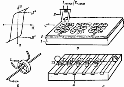
Рис. 2. Кривая намагничивания (а) и элементы магнитной памяти на ферритовых кольцах (б), движущемся магнитном носителе (в), цилиндрическом магнитном домене (г): 1 — подложка; 2 — магнитный носитель; 3 — головка записи/считывания; 4 — система проводников; ГЗ и ГЧ — головки записи и считывания.
