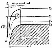
Рис. 4. Участок волевой диаграммы приповерхностной области МДП-структуры (рис. 3, в) в режиме сильной инверсии; \epsilon_F — середина запрещенной зоны; \Phi — электростатический потенциал; заштрихованы состояния, занятые электронами при T \rightarrow 0 К.
