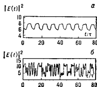
Рис. 5. Режимы периодического и хаотического изменений интенсивности света на выходе кольцевого ОР с нелинейной средой: а — при I_{\text{вх}} = 6,7 ; б — при I_{\text{вх}} = 11,6 .
