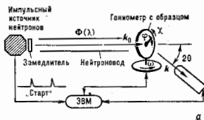
Рис. 2. а — схема дифрактометра по времени пролета на импульсном источнике нейтронов; б — построение Эвальда.
