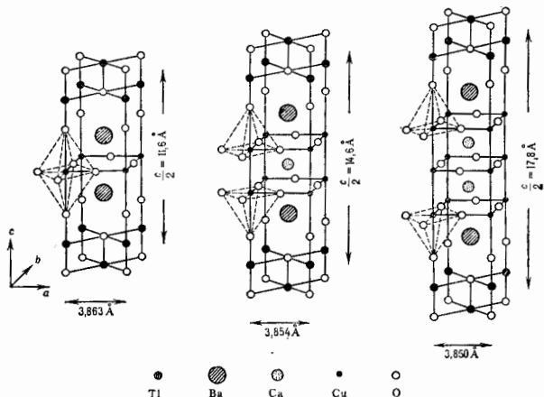
Рис. 4. Кристаллическая структура таллиевых (висмутовых) оксидных сверхпроводников: слева — \text{TlBa}_2\text{CuO}_4 ( \text{Bi}_2\text{Sr}_2\text{CuO}_4 ), в центре — \text{Tl}_2\text{Ba}_2\text{CuO}_4 ( \text{Bi}_2\text{Sr}_2\text{CaCuO}_4 ), справа — \text{Tl}_2\text{Ba}_2\text{CaCu}_2\text{O}_4 ( \text{Bi}_2\text{Sr}_2\text{Ca}_2\text{CuO}_4 ).
