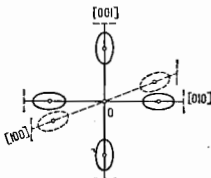
Рис. 1. Изоэнергетические поверхности электронов в зоне Бриллюэна для Si; пункт 1 — граница зоны Бриллюэна.
