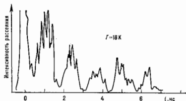
Рис. 7. Экспериментальные данные нестационарной КАРС-спектроскопии кристалла сорбидина, полученные при длительности импульса t_{\text{им}} , меньшей периода молекулярных колебаний T_M .
