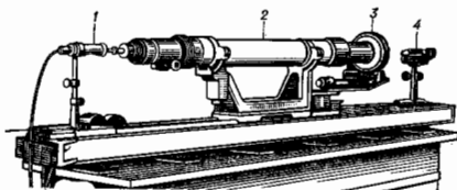
Оптическая скамья ОСК-2: 1 — осветитель; 2 — коллиматор; 3 — support с вращающейся универсальной оправкой; 4 — микрометр.
