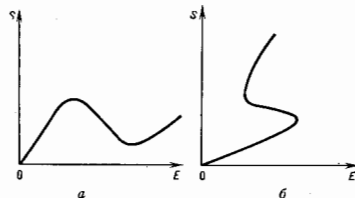
Рис. 4. N-образная (а) и S-образная (б) вольт-амперные характеристики.
