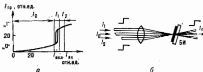
Рис. 2. Передаточная характеристика БИ в проходящем пучке (а) и схема устройства с логическими функциями «И», «НЕ», «ДЛИ» (б).
