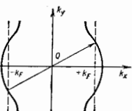
Рис. 2. Поверхность Ферми в квазиодномерном металле. Туннелирование показывает поверхность Ферми без учёта движения электронов между цепочками; переход на вектор Q смещает правую и левую части поверхности Ферми. Ось x направлена вдоль цепочек.
