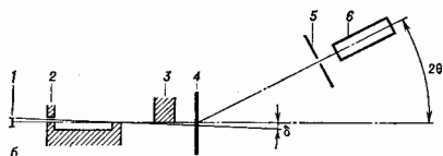
Рис. 7. Схемы малоугловых гониометров: а — трёхщелевая; б — по Кратки; 1 — фокус источника; 2 — формирующие ще- ли; 3 — щели образца; 4 — образцы; 5 — приемные щели; 6 — детектор (2θ — угол рассеяния; δ — угловая расходимость падающего пучка).
