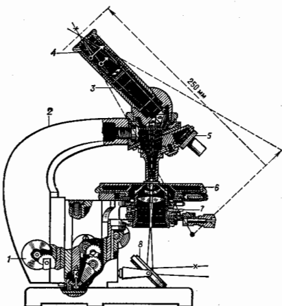
Рис. 4. Разрез биологического микроскопа и ход лучей: 1 — микрометр; 2 — тубодержатель; 3 — тубус; 4 — окуляр; 5 — объектив; 6 — предметный столик; 7 — конденсор; 8 — зеркало.
