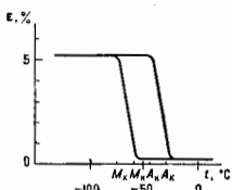
Рис. 1. Изменение длины образца из сплава \text{Cu} - \text{Al} - \text{Ni} при охлаждении и нагреве под действием постоянной нагрузки \sigma = 20 \text{ МПа} .
