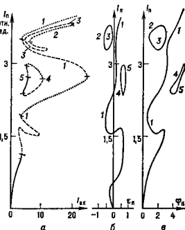
Рис. 3. Передаточные характеристики кольцевого оптического резонатора с нелинейной гиротропной средой при наличии поляризационного самодействия: а — зависимость I_{\text{вх}}(I_{\text{вых}}) ; б — \Phi_{\text{вх}}(I_{\text{вых}}) ; в — \Phi_{\text{вх}}(I_{\text{вых}}) . Цифрами помечены различные ветви оптической бистабильности.
