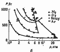
Рис. 5. Пороговые мощности, необходимые для поддержания непрерывного оптического разряда в атомарных (а) и молекулярных (б) газах (нижние ветви кривых). Верхние ветви кривых показывают верные пределы существования НОР.
