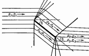
Рис. 3. Схема сверхзвукового обтекания пластины:
