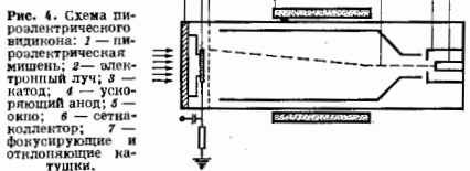
Рис. 4. Схема пирозлектрического видикона: 1 — пирозлектрическая мишень; 2 — электронный луч; 3 — катод; 4 — ускоряющий анод; 5 — окно; 6 — сетчатый коллектор; 7 — фокусирующие и отклоняющие катушки.
