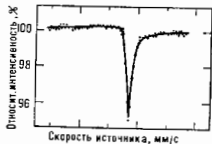
Рис. 6. Спектр поглощения мо- таллического Та; источник в спектрометре (рис. 3) ^{119}\text{Os} в мо- таллическом W.
