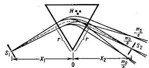
Рис. 3. Схема статического масс-спектрометра с однородным магнитным полем; S_1 , S_2 — щели ионного источника и приёмника ионов; треугольник — область однородного магнитного поля H ; перпендикулярная плоскость рисунка; тонкие сплошные линии — границы пучков ионов с разными m/e ; r — радиус центральной траектории ионов.
