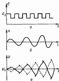
Рис. 1. Связь между изменениями емкости C конденсатора (а), заряда q на его обкладках (б) и напряжения U (в) при параметрическом резонансе в колебат. контуре.
