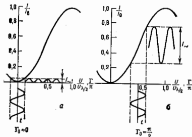
Рис. 2. Амплитудная характеристика модулятора света: а — работа на синусоидном участке при \Gamma_0 = 0 ; б — работа на линейном участке при \Gamma_0 = \pi/2 .
