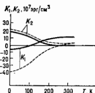
Рис. 1. Температурные зависимости констант анизотропии для \text{NdCo}_5 (пунктир) и \text{PrCo}_5 (сплошная линии).
