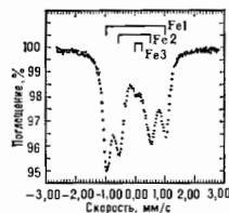
Рис. 6. Магнитное расщепление линий ^{57}\text{Fe} в спектре поглощения \text{YBaCu}_3 - x\text{Fe}_2\text{O}_6 при обычной температуре (а) и дополнительном расщеплении при T = 4,2 К (б); Fe1, Fe2, Fe3 соответствуют различным позициям атомов ^{57}\text{Fe} (рис. 4).
