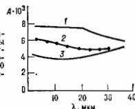
Рис. 2. Зависимости коэффициента поглощения серебра от длины волны при комнатной температуре: 1, 2 — расчет по теории аномального скин-эффекта при p=0 и p=1 соответственно; 2 — эксперимент.
