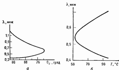
Рис. 2. Зависимость длины волн, генерируемой параметрическим генератором света, от угла синхронизма \theta_c (а) и температуры T (б) при \lambda_H = 0,266 мкм; e = \infty .
