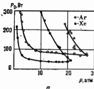
Рис. 5. Пороговые мощности, необходимые для поддержания непрерывного оптического разряда в атомарных (а) и молекулярных (б) газах (нижние ветви кривых). Верхние ветви кривых показывают верные пределы существования НОР.
