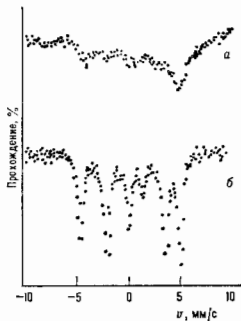
Рис. 8. Спектр поглощения монохроматизированного при T = 4,2 К без внешнего магнитного поля (а) и в поле H = 200 Э (б).
