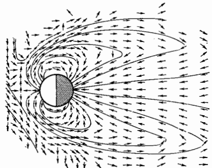
Рис. 3. Схема осесимметричной магнитосферы (возможная магнитосфера Урана) по данным лабораторного эксперимента. Стрелками показано направление магнитного поля, сплошными линиями — линия магнитного поля в магнитосфере.
