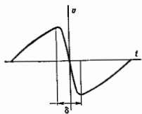
Рис. 1. Профиль волны конечной амплитуды.
