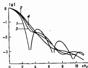
Рис. 3. Нормированные интенсивности малоуглового рассеяния частицами различной формы с одинаковыми R_g и т.: 1 — шаровой слой; 2 — трёхосный эллипсоид с отношением осей 0,5 : 1 : 1,5; 3 — четыре соприкасающихся эллипсоида вращения; 4 — литая модель по мотивам модели 3.
