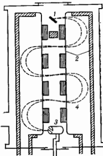
Рис. 4. Установка ИТФФ для измерения массы нейтрино: 1 — источник; 2 — питии магнитного спектрометра; 3 — ФЭУ; 4 — траектория электронов.
