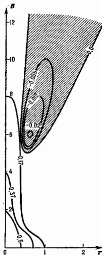
Рис. 1. Линии равной концентрации при диффузии точечного возмущения в одномерной неограниченной плазме. Размеры области возмущения вдоль поля в 10 раз больше области возмущения поперёк поля.
