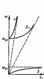
Рис. 1. Дисперсия нормальных волн в изотропной неэлектрохимической плазме: 1 — поперечные электромагнитные волны; 2 — лентморские волны; 3 — ионно-акустические волны.
