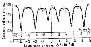
Рис. 5. Спектр резонансного поглощения выращенной линии 14,4 кэВ ^{57}\text{Fe} в металлическом железе, обусловленный внутренним магнитным полем, действующим на ядро ^{57}\text{Fe} в металле ( \Delta E \sim 10^{-4} эВ).
