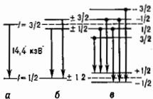
Рис. 2. Схема уровней ^{57}\text{Fe} и переходов между ними: а — без расщепления; б — нквдрупольное расщепление уровней в неоднородном электрич. поле; в — расщепление в неоднородном магнитном поле; I — спин ядра.
