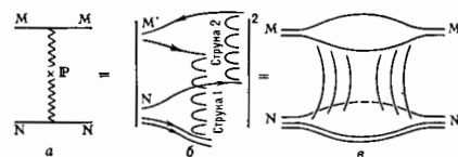
Рис. 2. Графики, описывающие вклад реджеона: а — обмен помероном P ; б — соответствующее сечение процесса множественного рождения, отвечающее разрыву двух струн; в — соответствующая кварковая диаграмма, имеющая топологию поверхности цилиндра.
