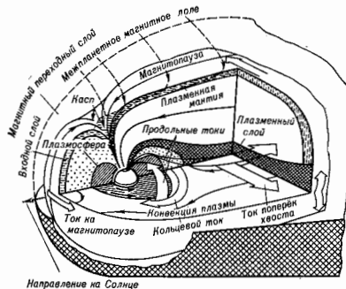
Рис. 1. Пространственное распределение плазмы, магнитных полей и электрических токов в магнитосфере Земли. Светлыми стрелками показаны токи на магнитопаузе и в плазменном слое, кольцевой и продольные токи. Тёмные стрелки указывают направление вращения плазмасферы совместно с Землей. Показаны также направления конвенции в хвосте магнитосферы. Точками отмечена область кольцевого тока.
