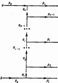
Диаграмма мультипериферического взаимодействия: а, б — первичные частицы; p_i , p'_i — их 4-импульсы.
