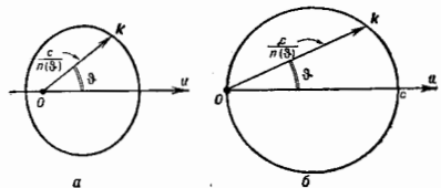
Рис. 1. Поверхности фазовой скорости в движущейся среде ( \theta — угол между направлением волнового вектора k и скоростью движения среды u ; a — для случая u < c/\sqrt{\varepsilon} ; b — для u = c ).
