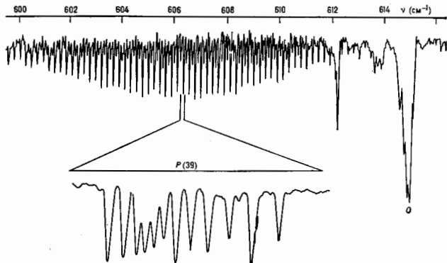
Рис. 2. ИК-полюса поглощения \nu_k молекулы SF_6 , полученная на фуре-спектрометре с разрешением 0,04 \text{ см}^{-1} ; ниже показана тонкая структура линии P(39), измеренная на диодном лазерном спектрометре с разрешением 10^{-4} \text{ см}^{-1} .
