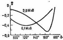
Рис. 2. Функция Шермана для золота при энергиях электронов 0,1 МэВ и 2,0 МэВ.
