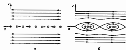
Рис. 2. Нейтральный слой в плазме: а — конфигурация неустойчива из-за притяжения друг к другу параллельных токов, текущих поперек магнитного поля (кружки); б — спонтанное пересоединение магнитных полей (образование магнитных островов).
