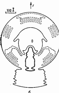
Рис. 4. а — Кривые рентгеновского малоуглового рассеяния бактериофага Т7 в растворе (1 — экспериментальная кривая; 2 — рассеяние восстановленной структуры); б — восстановление по данным малоуглового рассеяния структура Т7; рассчитанная в аксиально-симметричном приближении карта электронной плотности (сечение, содержащее ось вращения z). Сплошные изолинии соответствуют электронной плотности 0,38e \cdot \text{\AA}^{-3} (гидратированный белок), штриховые — 0,42e \cdot \text{\AA}^{-3} (сильногидратированная ДНК), жирная линия — 0,52e \cdot \text{\AA}^{-3} (слабогидратированная ДНК).
