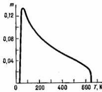
Рис. 2. Температурная зависимость магнитного момента m (в единицах \mu_B на молекулу) ортоферита дискет ( T_M = 40 К).
