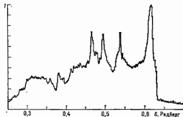
Рис. 3. Вычисленная зависимость плотности состояний от энергии g(\epsilon) для d -электронов в Ni.
