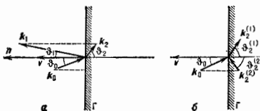
Рис. 3. Схема отражения и преломления волн на нормальном разрыве скорости движения сред: а) v < c/\sqrt{\epsilon_{1,2}\mu_{1,2}} — дисперсионное движение границы раздела двух сред; б) v > c/\sqrt{\epsilon_{1,2}\mu_{1,2}} — сверхсветовое движение границы раздела двух сред; \Gamma — граница раздела, движущаяся со скоростью v в направлении нормали n .
