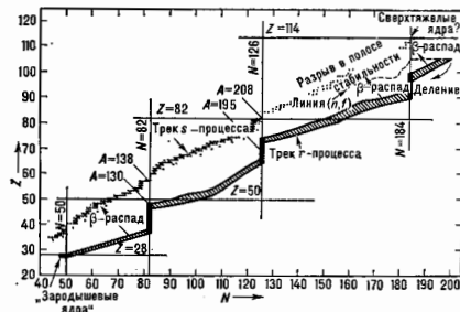
Рис. 2. Пути нейтронного захвата в s - и r -процессах. r -Процесс рассчитан для начальных температур 1,8-10^8 \text{ К} и концентрации нейтронов 10^{18} \text{ см}^{-3} . «Задержки» присоединения нейтронов в s - и r -процессах происходят, когда в ядрах число нейтронов N становится магическими ( N = 50, 82, 126 ). Этому соответствуют ниспа выходов нуклидов при массовых числах A , указанных на диаграмме наклонными линиями. Горизонтальными линиями показаны магические числа протонов, вертикальными — магические числа нейтронов. Направление \beta -распада показано стрелками. Линия (п, f) соответствует ядрам, которые испытывают деление при присоединении нейтрона. Разрыв в полосе стабильности связан со спонтанным делением. Деление обуславливает r -процесс в области ядер с Z \geq 100 , однако точная граница r -процесса неизвестна.
