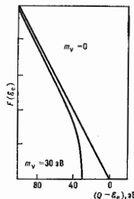
Рис. 3. График Кёри вблизи граничной точки без учёта фона и ночной разрешающей способности детектора.
