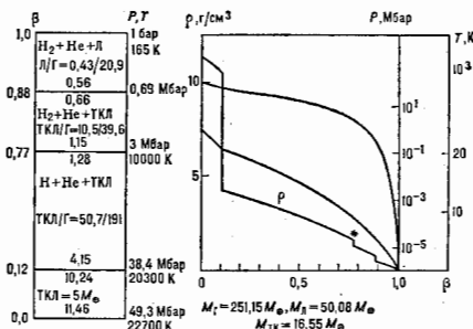
Рис. 2. Четырёхслойная модель Юпитера с двухслойной молекулярной оболочкой. Справа показано распределение давления P , темп-раты T и плотности \rho по относительному радиусу \beta = r/R_{\text{Ю}} ( R_{\text{Ю}} — радиус Юпитера). Слева даны расчёты модели с указанием значений плотности на границах раздела и отношения \text{Л}(\text{TKL})/\text{Г} в оболочках. Полные значения масс \text{Г} , \text{Л} и \text{TKL} -компонент выражены в массах Земли.
