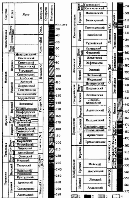
Рис. 1. Магнитостратиграфическая шкала докейнозойской части палеозоя СССР. Интервалы полярности: 1 — прямой, 2 — обратный, 3 — частое чередование, 4 — неисследованные.
