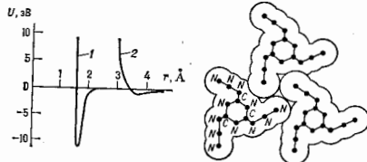
Рис. 1. Потенциалы химическ. (1) и физического (2) донца триатомной молекулы. На атомарный счет налета молекулярный «шуба».
