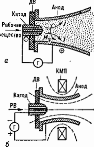
Рис. 4. Стационарные сильнотоковые плазменные ускорители: а — схема торцевого плазменного ускорителя (ДВ — диэлектрич. вставка); б — схема торцевого магнитоплазменного ускорителя (ДВ — диэлектрическая вставка; КМП — катушка магнитного поля; РВ — рабочее вещество).
