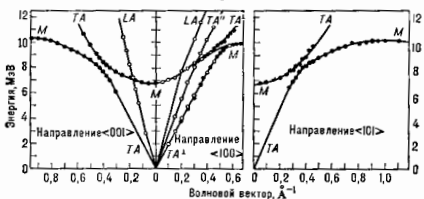
Рис. 4. Фононные и магнитная дисперсионные кривые в антиферромагнитном FeF_2 при T = 4,2 К. ТА — поперечный, LA — продольные акустические фононы, М — магнитоны.
