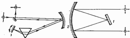
Рис. 2. Автоколлимационная схема: 1 — зеркало, вращением которого осуществляется сканирование спектра. Рис. 3. з-образная симметричная схема: 1 — дифракционная решётка; 2 — сферическое зеркало.
