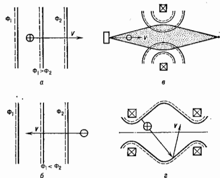
Рис. 2. Магнитоэлектрические плазменные устройства: а — ускорители компенсированных ионных пучков (КИП); б — рекуператоры энергии КИП; в — плазменная линза для фокусировки КИП; г — магнитоэлектрические плазменные ловушки; стрелочные линии — магнитные силовые линии; сплошные линии — эквипотенциалы.
