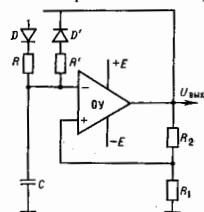
Рис. 2. Несимметричный мультивибратор на операционном усилителе.
