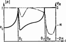
Рис. 2. Зависимость модуля коэффициента отражения звука |R| (сплошная линия) и его фазы \varphi_R (штрих-пунктирная линия) на границе жидкости и твёрдого тела от угла падения \theta_i .
