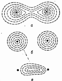
Рис. 4. а — электронная плотность, определенная методом РСА; б — вычисленная по нейтронам линия для сферически-симметричного атомного фактора; в — разностная плотность.
