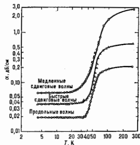
Рис. 7. Зависимость \alpha в монокристалле \text{AlO}_3 от темп-ры для продольных и поперечных волн с частотой 1 ГГц, распространяющихся вдоль оси C.
