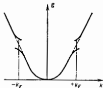
Рис. 1. Энергетический спектр электронов в пайерсовском диэлектрике (сплошные линии) и в металлической фазе (пунктир).
