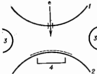
Рис. 11. Масс-спектрометр ионно-циклотронного резонанса.
