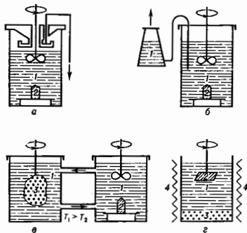
Рис. 2. Выращивания монокристалла из раствора: а — метод испарения растворителя; б — метод «подпитки»; в, г — метод температурного градиента. 1 — раствор; 2 — монокристалл; 3 — порошок; 4 — нагреватель.
