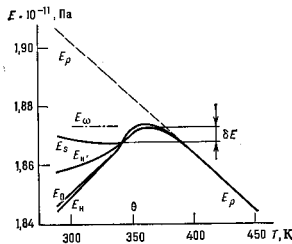
Рис. 2. Зависимости модуля упругости E поликристаллического образца выпарного сплава Fe—Ni—Cr от температуры T в различных магнитных полях.
