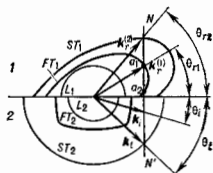
Рис. 3. Графический метод определения углов отражения и преломления на границе раздела кристаллических сред 1 и 2. L, FT и ST — поверхности волновых векторов для изаирипродольных, быстрых и медленных квазиизотропных волн соответственно.
