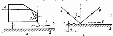
Рис. 3. Возбуждение поверхностных оптических волн: а — призмный метод, геометрия Отто; б — призмный метод, геометрия Кречмана; в — ретёничный метод, 1 — диэлектрик (воздух); 2 — ПАС (металл); 3 — призма; 4 — падающее излучение; 5 — поверхностная оптическая волна; 6 — зеркально отражённое излучение; 7 — ретётка; 1 — зазор размером \sim \lambda ; d — период ретётки.
