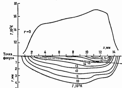
Рис. 6. Изотермы пространственного распределения температуры в НОР (низу) и распределение T на оси луча (вверху).
