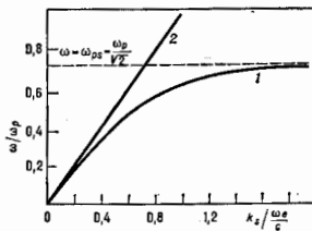
Рис. 2. Дисперсионная кривая поверхностных плазмон-полиритонов (1) на плоской границе раздела металла и вакуумом; \omega_p — плазменная частота электронов; 2 — свободная линия \omega = c k_y .
