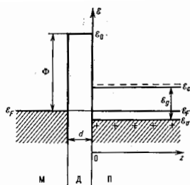
Рис. 2. Энергетическая диаграмма МДП-структуры на основе полупроводника p -типа при отсутствии напряжения V на затворе. Заштрихованы состояния, занимаемые электронами при T \rightarrow 0 К; \Phi — работа выхода металла; \epsilon_0 — энергия электрона в вакууме; \epsilon_F — потенциал валентной зоны; \epsilon_c — дно зоны проводимости; \epsilon_g — уровень Ферми; \epsilon_g — ширина запрещенной зоны полупроводника.
