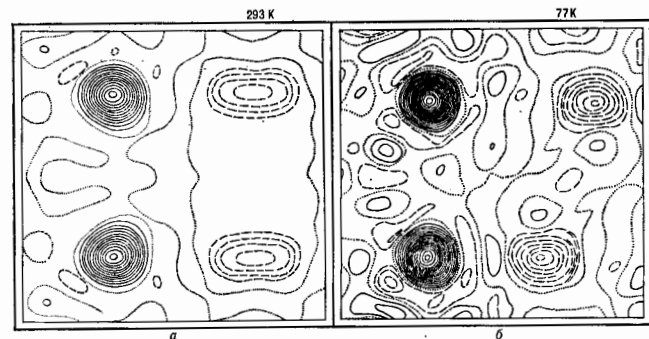
Рис. 3. Фрагмент проекции плотности амплитуды рассеяния \rho(r) на плоскость (001) в кристалле \text{KH}_2\text{PO}_4 при T = 293 \text{ K} (а) и T = 77 \text{ K} (б). Показаны 2 атома \text{O} ( \rho > 0 , непрерывные линии) и два атома \text{H} ( \rho < 0 , разрывные линии); точки соответствуют \rho = 0 .
