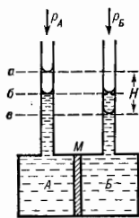
Схема осмометра: A — камера с растворителем, B — камера с раствором, M — мембрана; уровни жидкости в трубках при осмотическом равновесии: a и a' — в условиях равенства внешних давлений в камерах A и B (столб жидкости H уравновешивается \Delta p ); б — в условиях, когда \Delta p = \pi .
