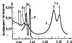
Рис. 2. Спектры одnofотонного (сплошная линия) и двухфотонного (пунктирная) поглощений в ZnO. Согласно правилам отбора, в одnofотонном спектре возникают только \sigma -висситные линии, в двухфотонном — только \pi -висситные линии.
