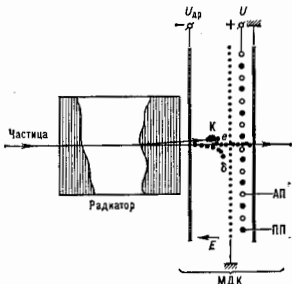
Рис. 2. Сечение детектора: МДК — многопроволочная дрейфовая камера; AP — анодные проволоки; PP — проволоки, формирующие поле; U_{др} — дрейфовый потенциал; U_{э} — электр. напряжение; \epsilon — электроны ионизации вдоль трека частицы; \delta — длина-электроны; K — кластер, образованный в результате фотоионизации газа фотоном рентгеновского переходного излучения.
