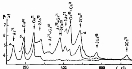
Рис. 5. Сигн. ЭПР в кристалле GaAs при T = 1,9 К и разных амплитудах переменного магнитного поля (рис. 2): а — односпинный резонанс ( H_1 \sim 0,16 Э), б — одно- и двухспинные ( H_1 \sim 1,6 Э), в — двух- и трёхспинные ( H_1 \sim 9,6 Э).
