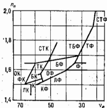
Диаграмма Аббе: ЛК — лёгкий кроун; ФК — флюатовый кроун; БК — баритовый кроун; ТК — тяжёлый кроун; СТК — сверхтяжёлый кроун; ОК — особый кроун; КО — кроун-флинт; ФЛ — флинт; ЛФ — лёгкий флинт и соответственно ТФФ, ТФ, СТФ, ОФ.
