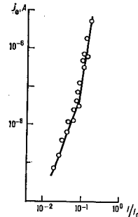
Рис. 2. Фотооток под действием резонансных импульсов рубинового лазера (натод из золота), I_0 = 14 МВт/см 2 .
