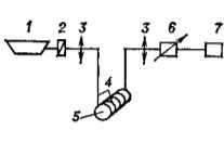
Рис. 2. Поляризационный приёмник звука: 1 — лазер; 2 — четвертьволновая пластина; 3 — микрообъектив; 4 — световод; 5 — упругий цилиндр; 6 — поляризационный анализатор; 7 — фотоприёмник.
