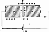
Рис. 1. Схематическое изображение р-п-перехода; чёрные кружки — электроны, светлые — дырки.
