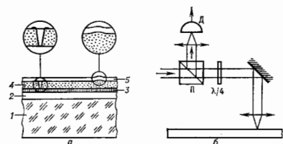
Рис. 1. Схема оптического диска (а) и устройства записи (считывания) информации (б): 1 — стеклянная подложка; 2 — отражающий зеркальный слой; 3 — прозрачный диэлектрик с низкой температурой; 4 — информационный носитель; 5 — прозрачный защитный слой; П — поляризационный оптический светоделитель; Д — детектор.
