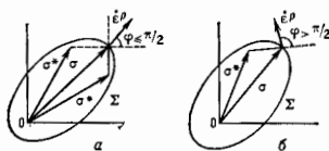
Рис. 4. а — вектор \epsilon^p ортогонален к поверхности нагружения; для любых \sigma^* неравенство Мизеса выполняется; угол между векторами \sigma - \sigma^* и \epsilon^p меньше или равен \pi/2 ; б — вектор \epsilon^p неортогонален к поверхности нагружения. Найдётся такое \sigma^* , при котором неравенство Мизеса не выполняется; угол между векторами \sigma - \sigma^* и \epsilon^p больше \pi/2 .
