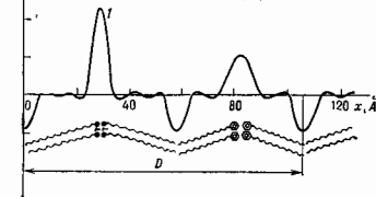
Рис. 6. Профиль электронной сверхрешётки (кривая 1) и схема расположе- ния молекул Бег. Ва и ОДФ в би- блиях. Период сверхрешётки D = 100 \text{ \AA} .
