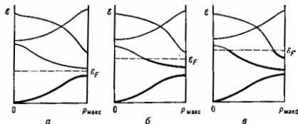
Рис. 1. Схема заполнения зон диэлектрика или полупроводника (а), металла (б), полуметалла (в). Жирные линии \mathcal{E}_i(p) — заполненные состояния, тонкие — пустые; нули — уровни химического потенциала, совпадающий в металлах с уровнем Ферми \mathcal{E}_F при T = 0 \text{ К} , p_{\max} — максимальный квазиимпульс, соответствующий границе зоны Бриллюэна.
