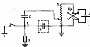
Рис. 2. Статический метод определения пирозлектрического коэффициента.
