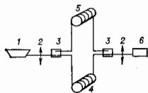
Рис. 1. Приёмник звука с интерферометром Маха-Цендера: 1 — лазер; 2 — микрообъектив; 3 — ответвитель; 4 — сигнальный световод на изгибе; 5 — опорный световод; 6 — фотоприёмник.
