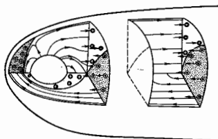
Рис. 2. Комбинированная магнитосфера. Линиями показаны силовые линии магнитного поля, крестиками и точками — направление магнитного поля, заштрихованные области соответствуют наведённому, незатрихованные — собственному магнитному полю.
