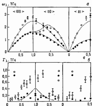
Рис. 1. а — фоновые дисперсионные кривые \omega_{\lambda}(q) ; б — затухание \Gamma_{\lambda}(q) для продольных (○) и поперечных (●) акустических фононов в гранцентрированной кубической решётке «Не» при T = 16 К (молярный объём 11,72 см 3 ); пунтир — теоретические кривые.
