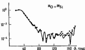
Рис. 9. Дифференциальное сечение упругого рассеяния ионов ^{40}\text{Ca} на ядрах ^{28}\text{Si} при энергии ионов E = 34,8 МэВ в зависимости от угла рассеяния \theta (в системе центра масс).
