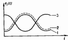
Рис. 2. Изменение амплитуд колебаний трёх взаимодействующих осцилляторов ( \omega_1 > \omega_2 ).
