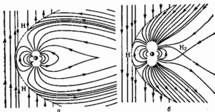
Рис. 2. Структура магнитного поля магнитосферы Земли (меридиональный разрез) при северном (а) и южном (б) направлении межпланетного магнитного поля (север вверх). Буквами H_1 , H_2 , N_1 отмечены области вблизи нейтральных точек магнитного поля.
