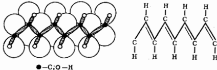
Рис. 6. Молекула полиацетилена: слева — распределение электронной плотности (затрихованы \sigma -связи); справа — структурная формула.
