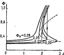
Рис. 4. Зависимость стационарной температуры \Phi от параметра p . Пунктиром обозначена спинопольная кривая, проходящая через точки, где \Phi(p) имеет вертикальную касательную. Для кривой \Phi_H = 0.22 стрелками показана петля гистерезиса.
