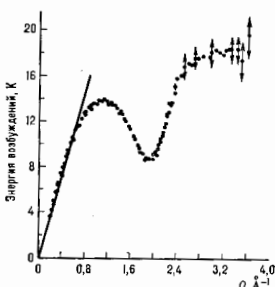
Рис. 3. Зависимость энергии коллективных возмущений Q от волнового вектора Q в сверхтекучем гелии при T = 1 К.
