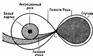
Сечение критической аккреционной поверхности орбитальной плоскости тесной двойной системы и схематическое представление перетекания газа от спутника через точку L_1 .
