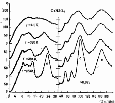
Рис. 2. Взвешенная плотность фоновых состояний \varphi в зависимости от энергии фононов при различных температурах.
