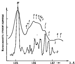
Рис. 1. Спектр вакуумной искры (I) и солнечной короны (S) (линии ионов Fe XXIV—XXV).
