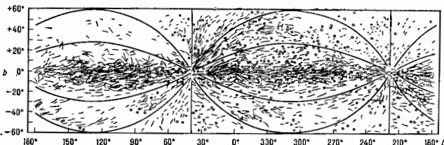
Рис. 1. Распределение межзвездной линейной поляризации в Галактике. Длина черточек пропорциональна степени наблюдаемой поляризации. Кружочки обозначены звезды с нулевой поляризацией. Дуговые линии показывают ход силовых линий межзвездного магнитного поля, которые, по данным оптической поляризации, сходятся в точках с галактическими координатами: l = 39^\circ , b = 0^\circ и l = 219^\circ , b = 0^\circ .
