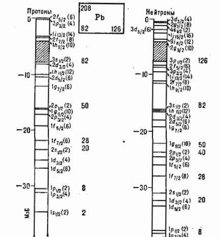
Схема одночастичных уровней ^{208}\text{Pb} ( N = 82 , Z = 126 ) в потенциале Саксона — Вудса. В круглых скобках даны числа частиц на отдельных уровнях ( N = 2, 4, 6 ); справа указаны магические (и полумагические) числа, отвечающие заполнению оболочек. Затрихованы магные просветы, отделяющие заполненные уровни от незаполненных.
