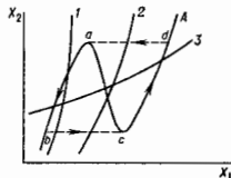
Рис. 6. N-образная нуль-изо-клина «быстрой» переменной (А), пересекающаяся с моно-тонной нуль-изо-клиной «медленной» переменной. Различ-ные случаи отвечают следующему (1), автоколебательному (2) и триггерному (3) режимам.
