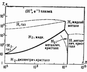
Рис. 1. Диаграмма состояния водорода.
