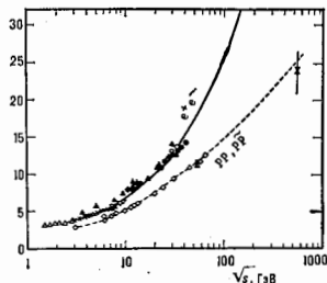
Рис. 2. Зависимость средней множественности заряженных частиц ( \langle n_{ch} \rangle ) от полной энергии в системе центра инерции \sqrt{s} для взаимодействий pp и p-p (пунктирная линия — формула (1)) и для e^+e^- (сплошная линия — формула (2)).
