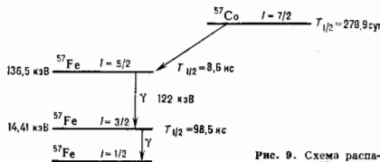
Рис. 9. Схема распада ^{57}Co .
