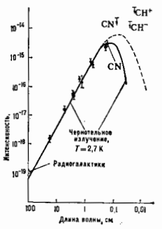
Рис. 1. Спектр микроволнового фоновое излучения Вселенной (интенсивность в эрг/(см 2 ·с·ср·Гц)). Эксперим. точки нанесены с указанием погрешностей измерений. Точки CN, CN¹ соответствуют результатам определения верхней границы (показана стрелкой) температуры излучения по населённости уровней соответствующих межзвёздных молекул.
