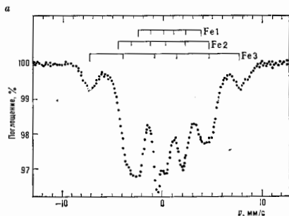
Рис. 5. Спектр резонансного поглощения выращенной линии 14,4 кэВ ^{57}\text{Fe} в металлическом железе, обусловленный внутренним магнитным полем, действующим на ядро ^{57}\text{Fe} в металле ( \Delta E \sim 10^{-4} эВ).
