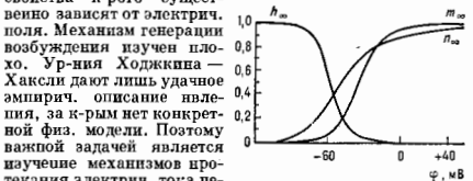
Рис. 4. Зависимость стационарных значений m , h и n от мембранного потенциала.
