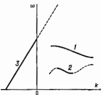
Рис. 1. Дисперсионные характеристики обратных волн (сплошные линии); нулевые линии соответствуют прямым волнам.
