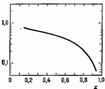
Рис. 4. Структурная функция заряженных пионов, характеризующая распределение входящих в пион кварков (партонов) в зависимости от условной доли x полного импульса пиона.
