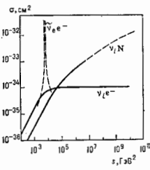
Рис. 8. Зависимости сечений рассеяния нейтрино и антинейтрино на нуклонах при s \approx m_W^2 (теоретические кривые).
