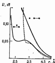
Рис. 3. Потенциалы взаимодействия He(2^1S) с молекулами водорода. Пунктирная кривая получена в экспериментах по рассеянию молекулярных пучков в сферически-симметричной аппроксимации. Теоретические кривые (сплошные) вычислены для различных взаимных расположений атомов He(^1S) и молекулы водорода (—•—).
