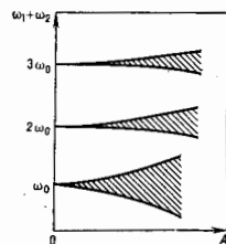
Рис. 1. Зоны распадной параметрической неустойчивости (Матье зоны) для основной частоты \omega_0 и гармоник ( n = 1, 2, 3 ).
