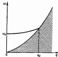
Рис. 1. Закон дисперсии плазмонов в металле (ионная р-ла). Затухающая область — одночастичные возбуждения; области q_c плазмоны сильно затухают.
