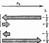
Рис. 5. Спиральности в состояниях левого нейтрино и правого антинейтрино. Длины стрел условно соответствуют вероятностям обнаружить \lambda = +1/2 и \lambda = -1/2 .
