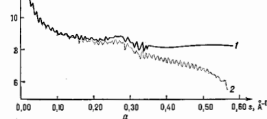
Рис. 4. а — Кривые рентгеновского малоуглового рассеяния бактериофага Т7 в растворе (1 — экспериментальная кривая; 2 — рассеяние восстановленной структуры); б — восстановление по данным малоуглового рассеяния структура Т7; рассчитанная в аксиально-симметричном приближении карта электронной плотности (сечение, содержащее ось вращения z). Сплошные изолинии соответствуют электронной плотности 0,38e \cdot \text{\AA}^{-3} (гидратированный белок), штриховые — 0,42e \cdot \text{\AA}^{-3} (сильногидратированная ДНК), жирная линия — 0,52e \cdot \text{\AA}^{-3} (слабогидратированная ДНК).
