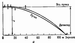
Рис. 2. Прибор для обнаружения заряда нейтрона.
