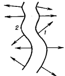
Рис. 1. Волновые фронты встречных волн: — падающей (1) и отраженной (2) — совпадают.
