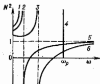
Рис. 10. Шесть типов волн в плазме при наличии магнитного поля: 1 — ионно-звуковая; 2 — альвеновская; 3 — быстрая магнитозвуковая (вистлер); 4 — легируемая; 5 — обыкновенная электромагнитная; 6 — необыкновенная.
