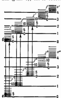
Рис. 1. Схема уровней энергии двухатомной молекулы: a, b, c — электронные уровни; 0, 1, 2, 3, 4, 5, 6 — колебательные квантовые числа; 0, 1, 2, 3, 4, 5, 6 — вращательные квантовые числа.
