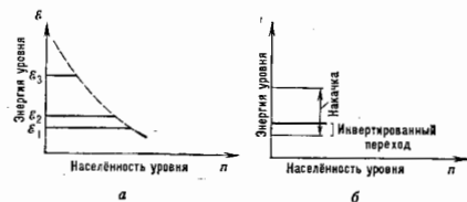
Рис. 1. Накачка трёхуровневой системы: распределение населённости уровней равновесное (а) и в условиях накачки перехода \mathcal{E}_1 - \mathcal{E}_3 (б).
