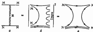
Рис. 1. Графики, описывающие вклад реджеона (R) в мнимую часть амплитуды упругого мезон-нуклионного (M — N) рассеяния: а — обмен реджеоном; б — соответствующее сечение (издают модули амплитуд) процесса множественного рождения адронов, отвечающее разрыву одной струны; в — соответствующая плоская топологическая кварковая диаграмма.
