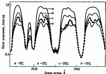
Рис. 1. Полоса поглощения TiO в спектре М-звезды. Относительное содержание редких изотопов титана определяют на сравнении рассчитанных профилей (отмечены буквами) с измеренными (точки).
