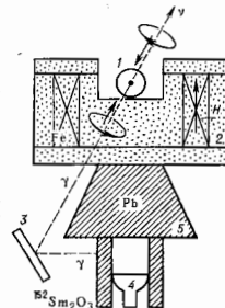
Рис. 2. Схема эксперимента М. Голдхабера, Л. Гродзинса, Э. У. Суныара: 1 — радиоактивный препарат ^{152}\text{Eu} ; 2 — магнитный анализатор (магнитное поле) для определения поляризации \gamma -кванта (рассеяние \gamma зависит от относительной поляризации \gamma и Fe); 3 — мишень, содержащая ^{152}\text{Sm} (резонансное рассеяние происходит в том случае, если \gamma и \nu испускаются в противоположных направлениях); 4 — детектор; 5 — свинцовый зашит.
