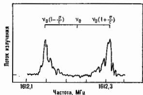
Рис. 2. Профиль линии мажорного излучения OH 1612 МГц, формирующийся в расширяющейся оболочке М-звезды. Скорость расширения оболочки v определяют по величине расщепления линии \Delta\nu = 2v_0/v_0 .
