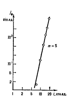
Рис. 1. Пятифотонная фотоэмиссия из золота под действием пикосекундных импульсов неодомового лазера.
