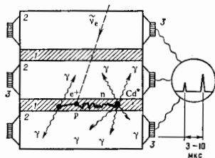
Рис. 1. Схема установки Райнса — Коузона (1956—57): 1 — мишени; 2 — сцинтилляционные детекторы; 3 — ФЭУ.
