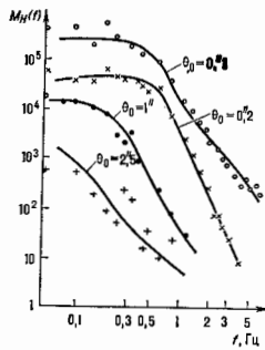
Рис. 2. Влияние угловых размеров источников \theta_0 на временные спектры межпланетных мерцаний. Сплошные линии — теоретические; точки — данные наблюдения, полученные на длине волны \lambda = 3 м, на угловых расстояниях от Солнца 30^\circ \pm 40^\circ , \circ — 58.2^\circ , \times — 43^\circ , \bullet — 3C 68,2, + — 3C 154.
