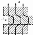
Рис. 4. Движение силовых линий магнитного поля B вместе с плазмой (свойство замкнутости силовых линий); v — скорость среды.
