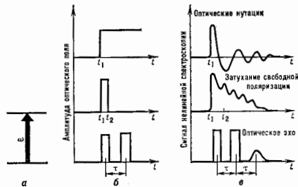
Рис. 4. Схемы когерентной нелинейной спектроскопии нестационарных процессов: а — двухуровневая система, с которой нестационарно взаимодействует резонансное оптическое поле; б — зависимость от времени амплитуды оптического поля в трёх различных схемах нелинейной когерентной спектроскопии: сверху — ступенчатое включение резонансного взаимодействия в момент времени t_1 ; средняя диаграмма — импульсное резонансное воздействие оптического поля на двухуровневую систему ( t_1 , t_2 — моменты начала и конца оптического импульса); внизу — резонансное воздействие оптического поля на двухуровневую систему в виде двух последовательных коротких импульсов, разделённых интервалом \tau ; г — временные диаграммы сигнала нелинейной спектроскопии, соответствующих амплитудам оптического поля на рис. б: сверху — сигнал оптических нутаций в амплитуде резонансной оптической волны, прошедшей сивоз образцы; средняя кривая — сигнал затухания свободной поляризации излучения, прошедшего через образцы; внизу — сигнал оптического эха в виде импульса излучения спустя время t после воздействия второго импульса.
