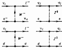
Рис. 6. Диаграммы рассеяния токов и измерения т. и. нейтринно на кварках и электронах.
