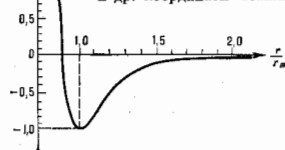
Рис. 2. Безразмерный потенциал взаимодействия симметричных пар атомов благородных газов. Отклонения от закона соответствующих состояний для различных атомов укладываются в различную ширину линии графика.
