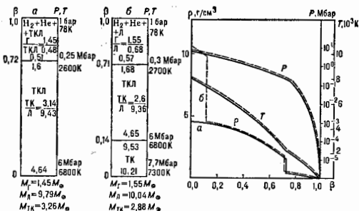
Рис. 3. Двух- и трёхслойные модели Урана с различной степенью смещения \Gamma , \Gamma - и ТК-компонент. Обозначения те же, что и на рис. 2.
