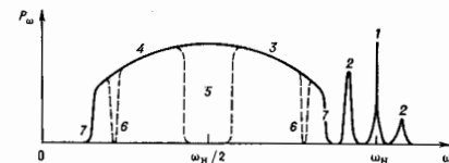
Рис. 4. Примерный вид спектра рассеяемого фазовоинтерференционного излучения: 1 — разное рассеяние; 2 — комбинационное рассеяние на поляритах и оптич. фононах; 3 — сигнальное параметрическое рассеяние; 4 — холодное параметрическое рассеяние; 5 — провал в области \omega_n/2 из-за отсутствия синхронизма; 6 — эффект «линейности» кристалла из-за прохождения квадратичной нелинейности через путь при смене знака; 7 — отсутствие синхронизма при уменьшении показателя преломления для холодной волны.
