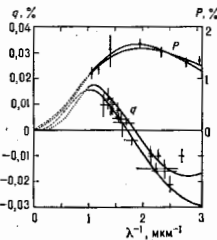
Рис. 2. Наблюдаемые и теоретические зависимости P(\lambda) и q(\lambda) для звезд \alpha Sco. Кривые — результаты расчетов для модели цилиндрических частиц с ненулевой длиной предельной m = 1,1 (точка) и m = 1,5-0,15 (штриховые).
