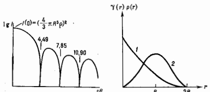
Рис. 1. Кривая интенсивности рассеяния однородным шаром радиуса R и плотности \rho : I(s) = (\frac{4}{3}\pi R^3 \rho)^2 [3(\sin sR - sR \cos sR)]^2 / (sR)^6 .
