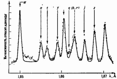
Рис. 3. Спектр плазмы тонамака (линии Fe XXIV–XXV).
