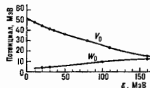
Рис. 2. Зависимость от энергии нейтронов \epsilon действительной и мнимой частей оптического потенциала (для случая обложного поглощения).
