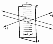
Рис. 3. Невязимый акустический элемент: 1 — возбуждающий звук; 2 — звукопровод; 3 — подложка звука.
