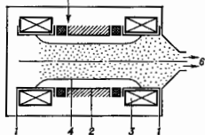
Рис. 1. Схема дугового плазмотрона постоянного тока: 1 — электроды; 2 — миниэлектронная установка; 3 — соленоиды; 4 — зона электрической дуги; 5 — подача рабочего тела; 6 — истечение плазмы.
