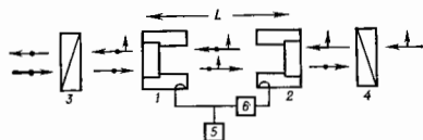
Рис. 2. Невязимый электрооптический элемент: 1, 2 — СВЧ-модуляторы света; 3, 4 — скрещённые поляризаторы; 5 — генератор СВЧ; 6 — фазовращатель.
