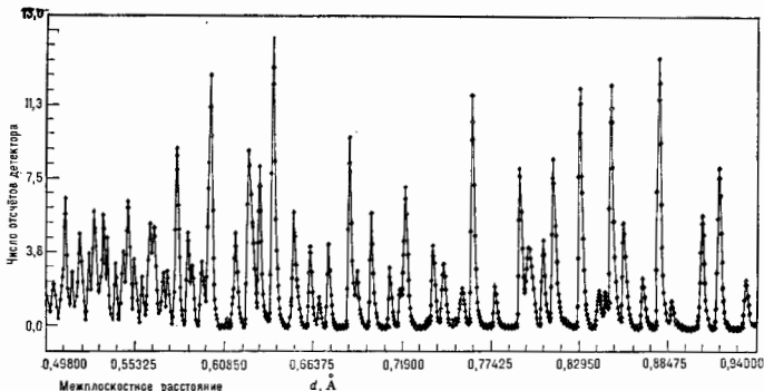
Рис. 5. Часть нейтронно-полюсристалла \text{Al}_2\text{O}_3 .
