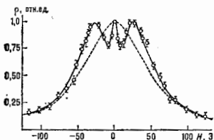
Рис. 4. Магнитная деполаризация люминесценции кристалла Al_{0.41}Ga_{0.59}As при T=77 К и \varphi=45^\circ ; при H=H_e \rho(H)=\rho(0) .
