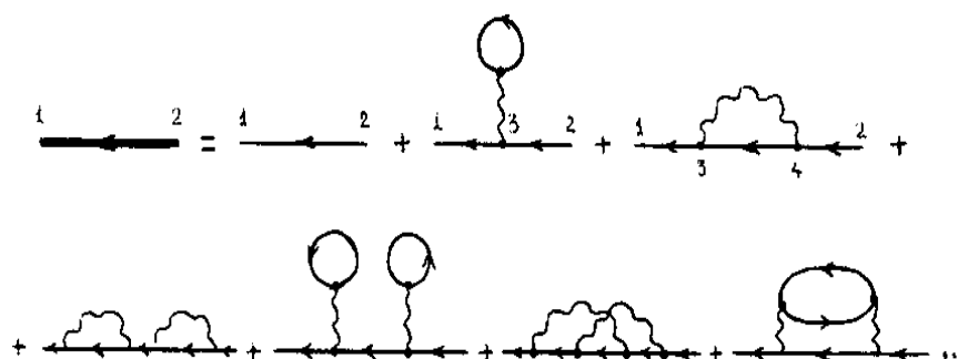
Рис. 11-6 Диаграммный ряд для полной (точной) функции Грина.
