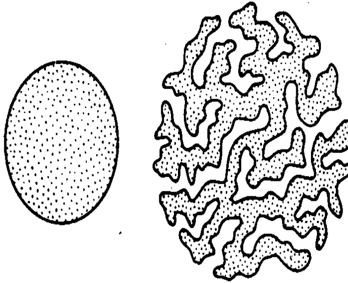
Рис. А-2 Качественная эволюция фазовой капли при перемешивании.
