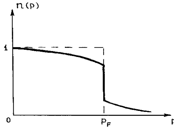
Рис. 11-2 Качественный вид функции распределения квазичастиц в ферми – жидкости при T = 0 .
