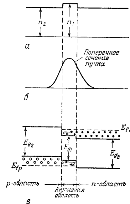
Рис. 6.44. а — профиль показателя преломления; б — поперечное сечение лазерного пучка; в — зонная структура полупроводника с двойным гетеропереходом, используемого в диодном лазере.
