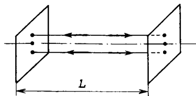
Рис. 4.1. Плоскопараллельный резонатор.
