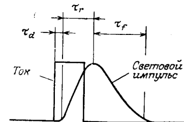
Рис. 6.50. Временная форма импульса, излучаемого полупроводниковым лазером при возбуждении прямоугольным импульсом тока.
