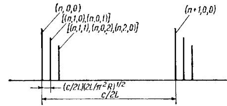
Рис. 4.36. Частотный спектр мод симметричного резонатора со сферическими зеркалами в случае, когда радиус кривизны зеркал R много больше длины резонатора L .
