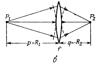
Рис. 4.11. Распространение сферической волны в свободном пространстве (а) и через линзу (б).
