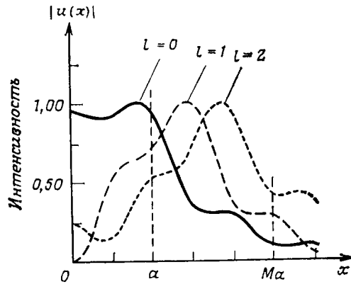
Рис. 4.43. Амплитудные профили трех собственных мод низшего порядка открытого неустойчивого резонатора с M=2,5 и N_{\text{экр}}=0,60 . (Согласно Сигмену [14].)
