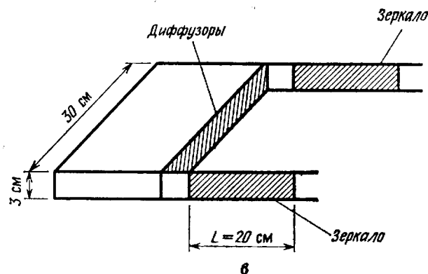
Рис. 6.22. Схема, иллюстрирующая работу газодинамического СО₂-лазера. а — принцип действия устройства; б — пространственное распределение населенности N^* верхнего и нижнего лазерных уровней (нормированной на населенность основного уровня N_{000} ); в — геометрия резонатора. (Рисунки а и б воспроизведены с разрешения редакции журнала IEE Spectrum, v. 7, № 11, 51—58 (1970); Copyright 1970 by the Institute of Electrical and Electronics Engineers, Inc.)
