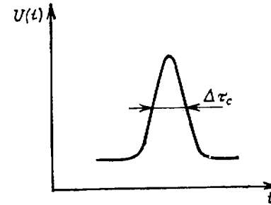
Рис. 3.26. Зависимость потенциала взаимодействия двух сталкивающихся частиц от времени.
