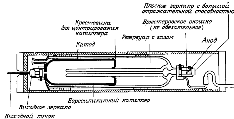
Рис. 6.6. Внутреннее устройство современного отпаянного гелий-неонового лазера (воспроизводится с любезного разрешения Мель Гриво).
