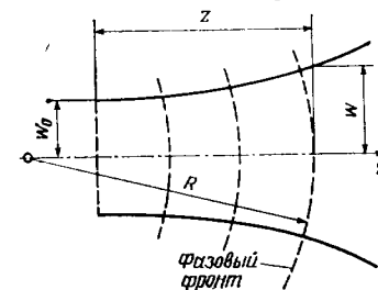
Рис. 8.1. Распространение гауссова пучка.
