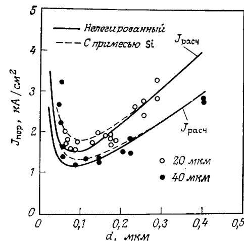
Рис. 6.46. Расчетные и экспериментальные значения пороговой плотности тока J_{\text{пор}} как функции толщины активного слоя d для ДГ-лазера на AlGaAs длиной 300 мкм с полосковой геометрией. Темные и светлые кружки представляют данные для ширины полосок соответственно 40 и 20 мкм. Расчетные кривые J_{\text{расч}} относятся к случаям собственного и слабо легированного кремнием активных слоев. (Согласно Киноне и др. [45].)
