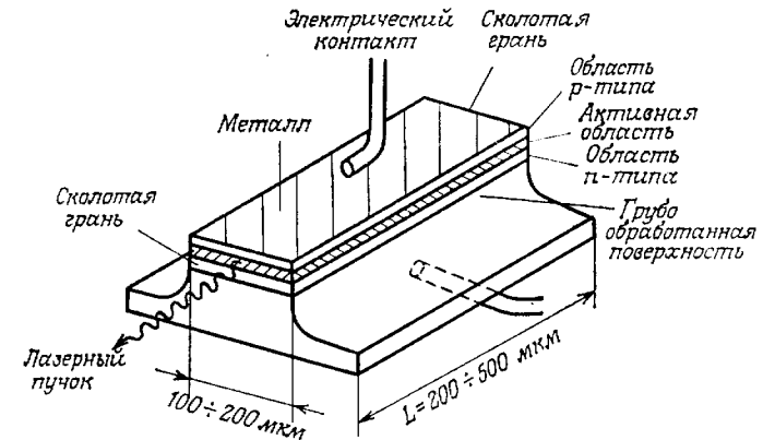
Рис. 6.42. Типичный GaAs-лазер с широким p-n -гомопереходом.
