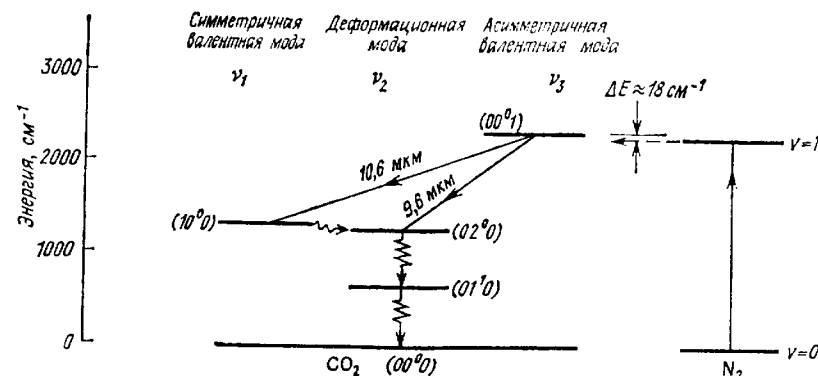
Рис. 6.14. Нижние колебательные уровни основного электронного состояния молекул \text{N}_2 и \text{CO}_2 (для простоты здесь не показаны вращательные уровни).
