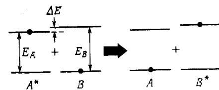
Рис. 3.17. Околорезонансная передача энергии.
