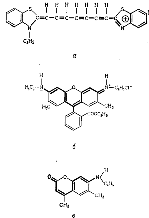
Рис. 6.28. Химическая структурная формула 3,3'-диэтилтиатрикарбоцианинидида подида (а), родамина 6G (б) и кумарина 2 (в). В каждом случае жирными линиями обозначен хромофорный участок молекулы красителя.
