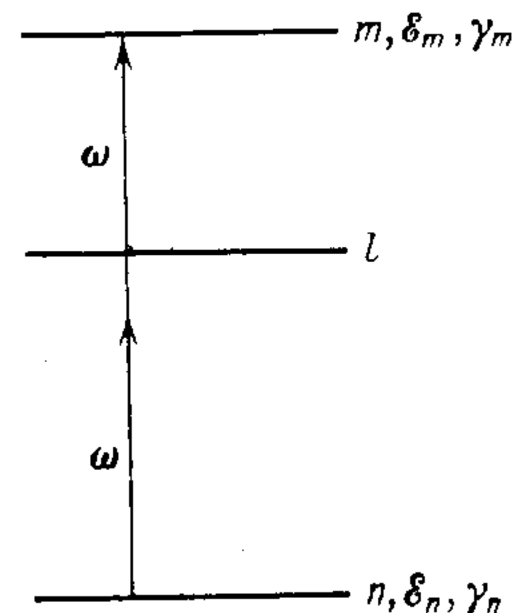
1. Схема процесса двухфотонного возбуждения: n, m — связанные электронные состояния; \varepsilon_n, \varepsilon_m — энергии; \gamma_n, \gamma_m — естественные ширины этих состояний; l — промежуточные состояния
