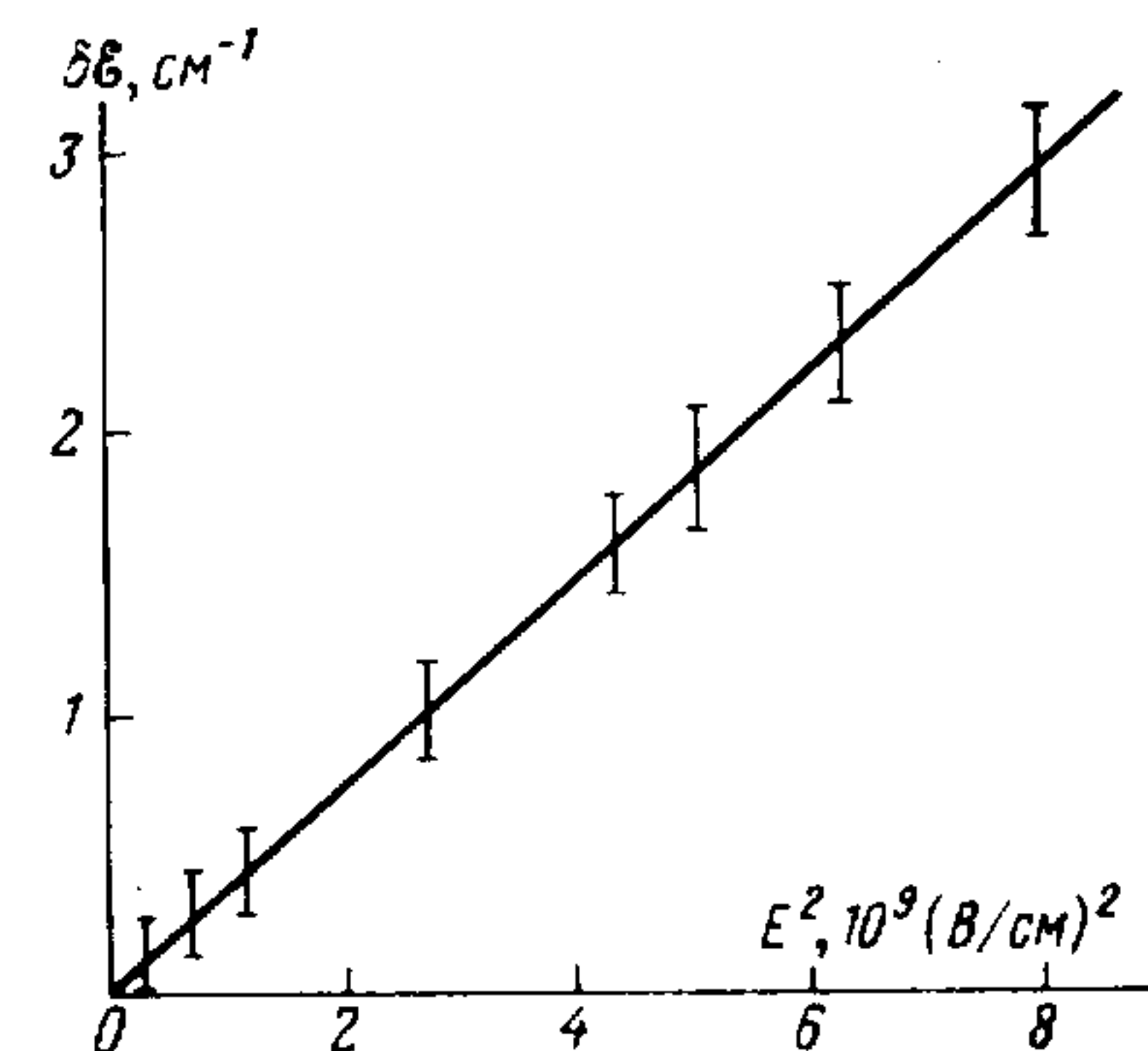
4. Результат измерения энергии \delta\mathcal{E} перехода 4S_{1/2} \rightarrow 4P_{3/2} в атоме калия в зависимости от квадрата напряженности поля излучения на нерезонансной частоте \omega
