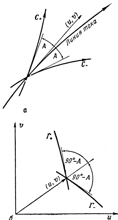
Рис. 7. Характеристические кривые.
