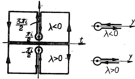
Рис. В.1. Контура интегрирования при вычислении интеграла Мельникова-Арнольда.
