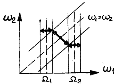
Рис.4.2. Перекрытие Трех резонансов: стрелками показаны вектора фазовых колебаний (\Delta\omega)^r для каждого резонанса.
