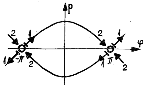
Рис. 2.1. Сепаратриса: О - усатый тор (точка); 1 - выходящие усы; 2 - входящие усы.
