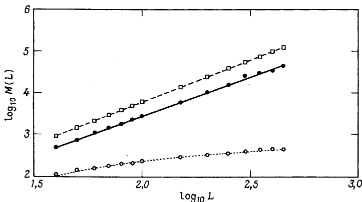
РИС. 7.4. Масса наибольшего кластера как функция линейного размера L квадратной решетки. Черные кружки соответствуют p = p_c = 0,593 . Сплошная
