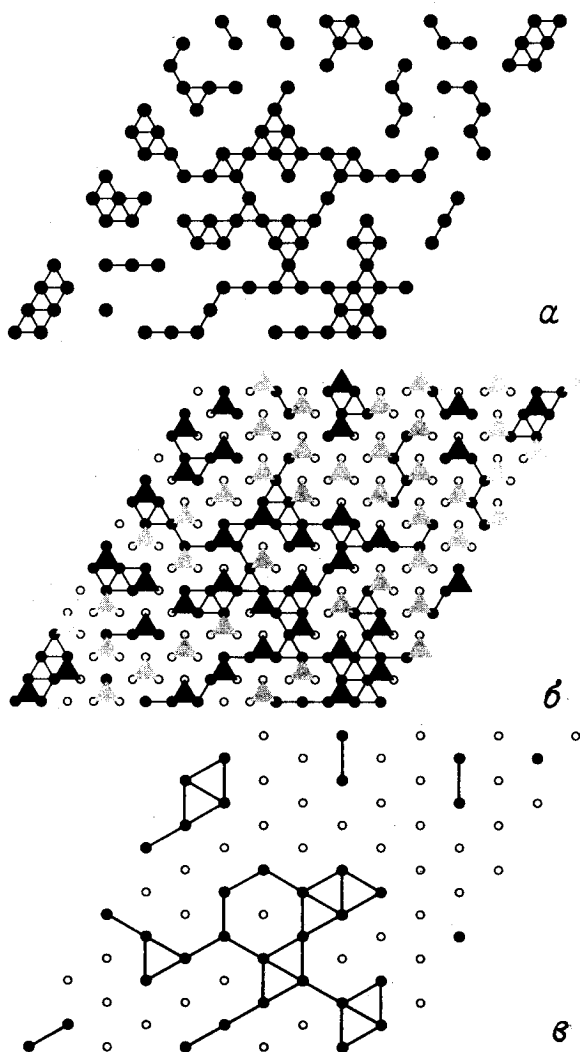
РИС. 7.7. a —кластеры на пороге кластеризации p_c на треугольной решетке; б —огрубление треугольной решетки в b = \sqrt{3} раз. Занятые узлы изображены черными кружками, незанятые (поры)—светлыми. Группы из трех узлов образуют блоки, обозначенные заштрихованными треугольниками. Если большинство узлов, принадлежащих треугольнику, занято, то треугольник выкрашен в черный цвет; в —огрубленная перколяционная решетка, на которой черные узлы соответствуют черным треугольникам на решетке б .
