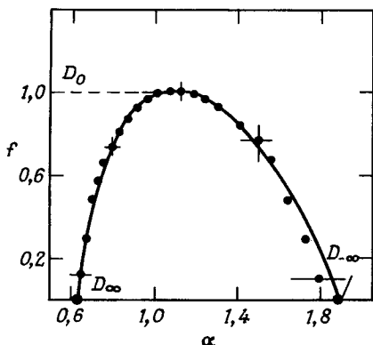
РИС. 6.11. Кривая f(\alpha) для тепловой конвекции. Точки заимствованы из наблюдаемого временного ряда. Показана кривая f(\alpha) для критического отображения окружности на себя. Следует подчеркнуть отсутствие свободных параметров и замечательное согласие теории с данными наблюдений [101].
