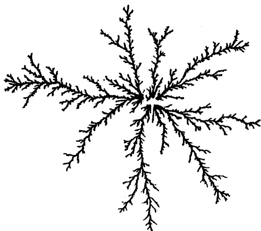
РИС. 3.4. Дендрит металла, выращенный электроосаждением цинка на поверхности раздела водного раствора сульфата цинка и n -бутилацетата. Фрактальная размерность D \approx 1,63 [150].
