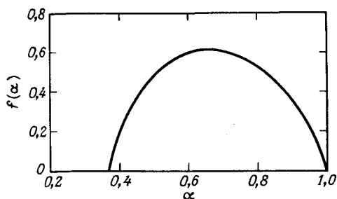
РИС. 6.8. Кривая f(\alpha) для двухмассовой фрактальной меры на канторовском стержне \mathcal{S} с l_0 = 1/4 , l_1 = 2/5 и массами p_0 = 3/5 , p_1 = 2/5 . Кривая описывает фрактальную размерность f подмножеств \mathcal{S}_\alpha с показателем Липшица – Гельдера \alpha как функцию \alpha .
