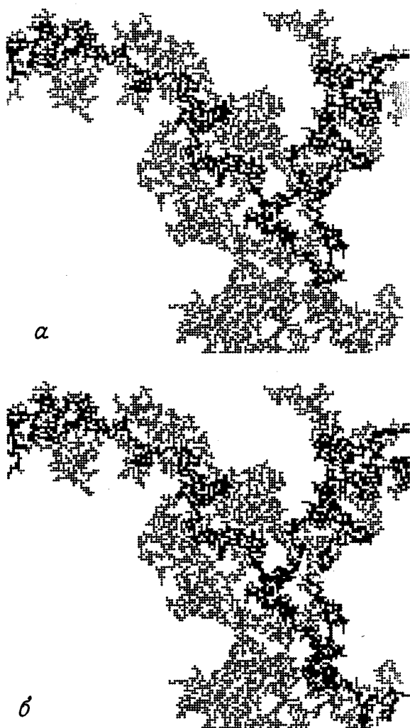
РИС. 7.15. Остовы перколяционного кластера на квадратной решетке, показанного на рис. 7.2, б, при критической концентрации p_c . a —Остов, связывающий отдельный узел на левой границе решетки размеров 160 \times 160 с отдельным узлом на правой границе; б —остов, связывающий все узлы на левой и правой границах.
