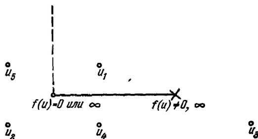
Рис. 6. Симметрии эллиптических функций Якоби.
