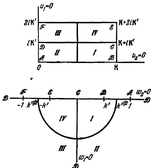
Рис. 10. Отображение w = \operatorname{dn}(u, k)
