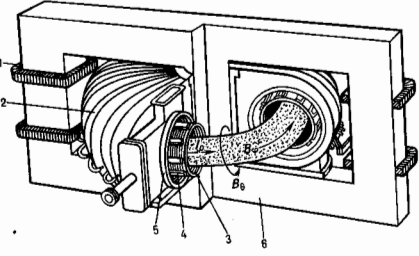
Рис. 1. Схема токамака: 1 — первичная обмотка трансформатора; 2 — катушки торoidalного магнитного поля; 3 — донорная катушка; 4 — катушки поперечного магнитного поля; 5 — вакуумная камера; 6 — железный сердечник (магнитопровод).
