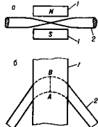
Рис. 2. Отклонение пучка заряженных частиц магнитной призмой: a — вид сверху; b — вид сверху; 1 — полюсы магн.та призмы; 2 — пучок заряженных частиц; AB — линейный фокус.
