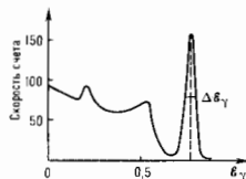
Рис. 4. Спектр импульсов от NaI(Tl) для E_{акт} = 661 КэВ.
