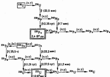
Рис. 1. Цепочки превращений ^{238}\text{U} — ^{239}\text{Pu} и ^{232}\text{Th} — ^{233}\text{U} .
