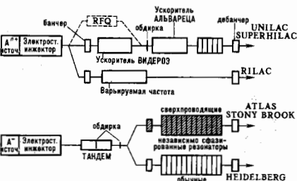
Рис. 6. Различные схемы линейных ускорителей тяжелых ионов.
