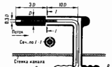
Рис. 1. Схема трубки Пито — Пранатля.
