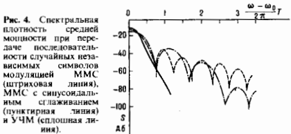
Рис. 4. Спектральная плотность средней мощности при передаче последовательности случайных независимых символов модуляцией ММС (штриховая линия), ММС с синусоидальным сглаживанием (пунктирная линия) и УЧМ (сплошная линия).
