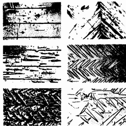
Рис. 2. Наблюдаемые доменные структуры в пластинах Fe 3% Si с поверхностью, оставшейся с осью [001] , лежащей в плоскости \{100\} , углы \beta=0^\circ (а), 2-4^\circ (б), 6-10^\circ (в), а также с поверхностями, составляющими с осями [001] и [010] углы \beta_{001}=\beta_{010}=0^\circ (с), \beta_{001}=0 , \beta_{010}=3-5^\circ (д), \beta_{001}=2-4^\circ и \beta_{010}=7-12^\circ (е). (Вильямс Х., Бозорт Р., Шоки Б., Шур Я. С., Драгошанский Ю. Н.)
