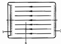
Рис. 1. Схема плоского электронно-оптического преобразователя: 1 — фотокатод; 2 — электронное поле; 3 — люминесцентный экран.
