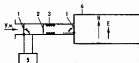
Рис. 3. Схема эксперимента по поиску электрического дипольного момента нейтрона: 1—клапаны впуска и выпуска нейтронов; 2—поляризатор; 3—контур спинового ротатора; 4—камера хранения; 5—детектор.
