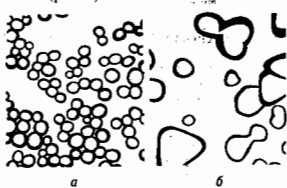
Рис. 1. Зёрна различных эмульсий (электронные микрофотографии, увеличение 20 000): а — ядерная фотозумульсия типа Илфорд-5; б — обычная фотозумульсия.
