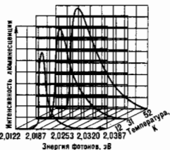
Рис. 2. Спектр люминесценции оксида меди: экситоны рекомбинируют из основного состояния, энергия рекомбинация равна сумме энергии основного состояния и кинетической энергии экситона. Ширина спектра уменьшается при понижении температуры.
