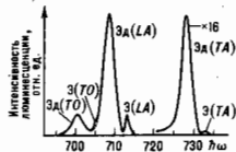
Рис. 3. Спектр люминесценции кристалла Ge при 4,2 К; Э—экситонные линии, Эд—линия электронно-дырочной жидкости (по В. М. В.).
