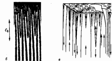
Рис. 1. Возможные типы доменных структур в магнитно-одноосных образцах с поверхностью, параллельной (а, б) и перпендикулярной (с) оси C_6 : а — схема, расшифровывающая наблюдаемые доменные структуры (Шур Я. С., Драгошанский Ю. Н.).
