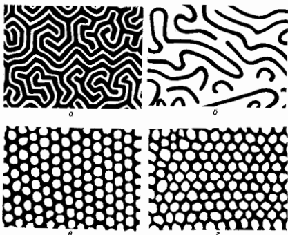
Рис. 2. Трансформация лабиринтной доменной структуры под действием внешнего поля: а — лабиринтная доменная структура; б — увеличение ЦМД; в — рёшётка ЦМД; г — сотовая доменная структура.
