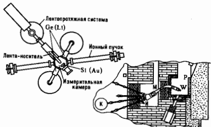
Рис. 1. Схема установки ЭЛПА для изучения радиоактивного распада короткоживущих нуклидов: р — выведенный пучок протонов синхротрона; W — вольфрамовая мишень, М — камера масс-сепаратора; И — ионопроводы; К — измерительная камера; Ge(Li), Si(Au) — полупроводниковые детекторы.
