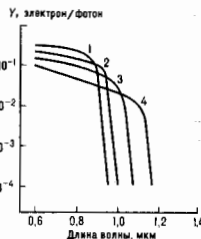
Рис. 4. Спектральные характеристики квантового выхода фотоэлектронов из полупроводников с ОЭС: Ga 1-x In x As—Cs—O. 1— \delta_p = 1,43 эВ; 2— \delta_p = 1,28 эВ; 3— \delta_p \approx 1,18 эВ; 4— \delta_p = 1,08 эВ.
