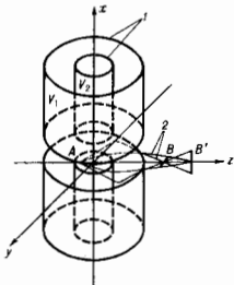
Рис. 10. Электростатическая трансаксальная электронная линза с электродами в виде двух соосных цилиндров с кольцевыми щелями для прохождения пучка электронов; 1—цилиндрические электроды; 2—траектории электронов; V_1 и V_2 —потенциалы электродов.
