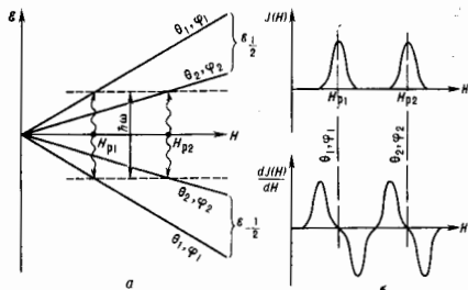
Рис. 1. Электронный парамагнитный резонанс: а—парамагнитная частица со спином S = 1/2 , помещённая во внешнее магнитное поле, имеет два подуровня ( \epsilon_{1,2} и \epsilon_{-1,2} ), каждый из которых изменяется пропорционально полю H и зависит от его ориентации по отношению к кристаллографическим осям, задаваемой углами \theta и \phi . При резонансных значениях магнитного поля H_{P1} и H_{P2} (углы \theta_1, \phi_1 и \theta_2, \phi_2 ) разность \epsilon_{1,2} - \epsilon_{-1,2} становится равной кванту энергии \hbar\omega СВЧ-излучения. При этом в спектре поглощения (б) наблюдаются характерные всплески вблизи H_{P1} и H_{P2} (приведены сигнал поглощения и его производная).
