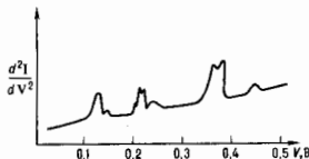
Рис. 3. Спектры примесей CH в туннельном переходе кремниевого диода.
