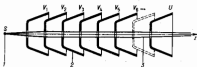
Рис. 5. Ускоритель прямого действия, состоящий из последовательности иммерсионных линз, электроды к-рых в форме усечённых конусов экранируют электронный нучок от внешних полей: 1 — источник электронов (им может быть кроссовер электронной пушки); 2 — электроды; 3 — электронный пучок; V_1, V_2, \dots — промежуточные потенциалы электродов; U — ускоряющее напряжение.
