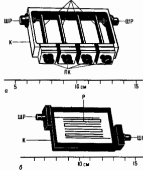
Рис. 3. Электрические фильтры — гребенчатый (а) и шпильный (б); ШР — шпильный резонатор, Р — резонатор, ПК — постстроенные конденсаторы, К — корпус (со снятой крышкой).
