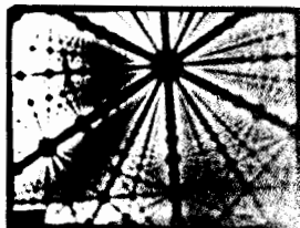
Рис. 3. Ионограмма монокристалла вольфрама.
