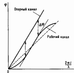
Рис. 2. Фазочастотные характеристики рабочего и опорного каналов фазовращателя на связанных линиях передачи.
