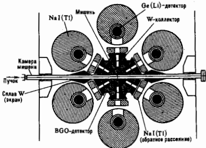
Рис. 3. Многодетекторный \gamma -спектрометр для исследования высококиповых состояний ядер, возбуждаемых в реакции с тяжелыми ионами.
