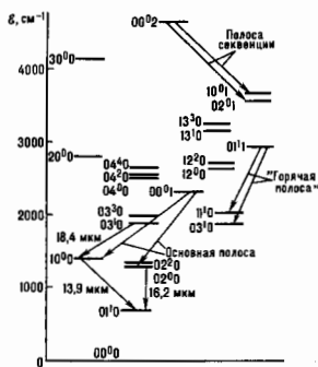
Рис. 2. Схема нескольких нижних колебательных уровней основной изотопической модификации ( ^{12}\text{C}^{16}\text{O}_2 ) молекулы \text{CO}_2 . Стрелками обозначены некоторые лазерные переходы; наиболее сильные из них — с уровня 00^1 на уровни 10^0 и 02^0 .
