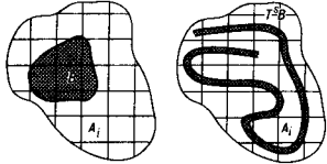
Рис. 3. Под действием перемешивающей системы образ множества B (т. е. T^t B ) с течением времени всё более равномерно заполняет фазовое пространство.
