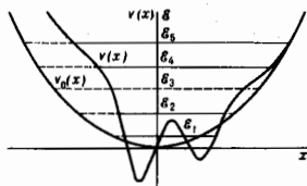
Рис. 6. Изменение формы потенциальной ямы [ v_0(x) \rightarrow v(x) ], необходимое для уничтожения уровня \epsilon_3 (пунктир). Сужение ямы вызвано сокращением числа колебаний собственных функций состояний, расположенных выше ликвидированного уровня. Форма дна ямы обеспечивает неизменность положения уровней \epsilon_1 и \epsilon_2 (в основном опускает уровень \epsilon_2 , поднимающийся при сужении ямы).
