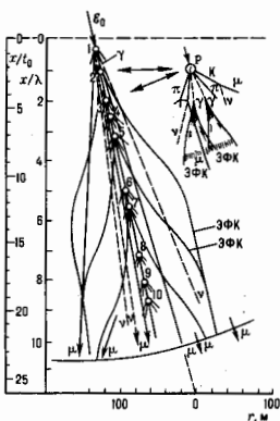
Fig. 2. Ядерный каскад в атмосфере. Цифрами показаны точки последовательных взаимодействий адрона высокой энергии; ЭФХ — электронно-фотонный каскад, l_0 — радиационная единица ливня.
