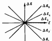
Рис. 1. Зависимость величины расщепления уровней энергии \Delta E от напряжённости электрического поля E при линейном эффекте Штарка (расщепление уровня энергии атома H , определяемого главным квантовым числом n=3 , на 5 подуровней).
