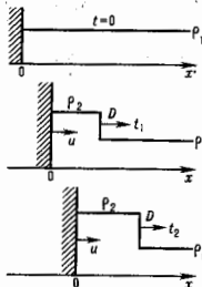
Рис. 1. Распределение плотности в последовательные моменты времени t=0 , t_1 , t_2 в ударной волне, возбуждаемой поршнем, движущимся с постоянной скоростью u ( D — скорость ударной волны; D > u ).
