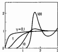
Рис. 1. Расчётные бинарные корреляционные функции ипов g(r/r_s) при различных параметрах неидеальности однокомпонентной плазмы (по горизонтальной оси r/r_s ).
