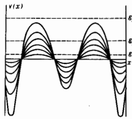
Рис. 2. Возмущения потенциала, вызывающие подъём уровня \epsilon_2 к \epsilon_3 . Увеличение v в области максимумов |\psi_2| сдвигает \epsilon_2 вверх, версильная линия: ямок притяжения вблизи узлов \psi_2 . Влияние барьеров и ямок на остальные уровни взаимно компенсируются — они остаются на прежних местах.
