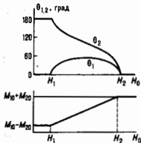
Рис. 2. Полевые зависимости углов между намагниченно- стями подрешоток и постоян- ным магнитным полем, а так- же суммарной постоянной на- магнитченности двухподре- шоточного ферримагнетика.
