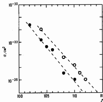
Рис. 2. Зависимость сечения образования трансуроновых элементов от их атомного номера Z . Светлые и черные кружки — соответственно реакции холодной и горячей слияния.
