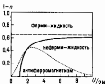
Рис. 4. Фазовая диаграмма при T=0 на плоскости (n, U) [7].
