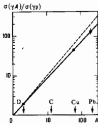
Рис. 3. Отношение R = \sigma(\gamma A) / \sigma(\gamma \pi) полных сечений адронного поглощения фотонов с \epsilon_s = 16 ГэВ на ядрах и на протонах в зависимости от числа A нуклонов в ядре.
