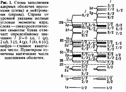
Рис. 1. Схема заполнения ядерных оболочек протонами (слева) и нейтронами (справа). Справа от уровней указаны полные угловые моменты ядра; слева — спектроскопические символы: буква отвечает определённому значению l ( l = 0 (s), 1 (p), 2 (d), 3 (f), 4 (g), 5 (h), 6 (i)); цифра — главное квантовое число. Пунктиром отмечены магические числа заполнения оболочек.
