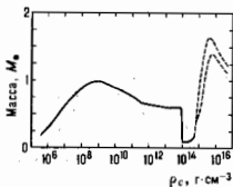
Рис. 6. Зависимость массы от центральной плотности для равновесных холодных звезд. Верхняя штриховая линия соответствует равновесию состояния для «холодных» нейтронов, нижняя — с учётом гравитации.
