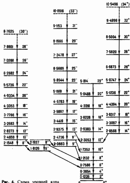
Рис. 4. Схема уровней ядра ^{104}\text{Hg} , возбуждаемых в реакции ^{124}\text{Sn} (^{48}\text{Ti}, 4n)^{104}\text{Hg} . Разделены ротационные полосы, основанные на состояниях различной природы.
