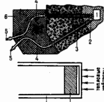
Рис. 2. Получение ультрахолодных нейтронов (горизонтальные каналы): 1—активная зона реактора; 2—конвертор внутри нейтронного канала; 3, 4—изогнутые участки нейтронного канала; 5—детектор нейтронов; 6—защита. Внизу показано расположение конвертора в нейтронном доде.
