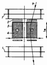
Рис. 6. Подземный магнитный спектрометр (МГС) для изучения мюонов высокой энергии: 1 — искровые камеры; 2 — сцинтилляционные детекторы; 3 — обмотка электромагнита; 4 — намагниченное железо; \mu — трек мюона.
