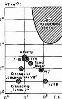
Рис. 3. Параметры, достигнутые на различных установках для изучения проблемы управляемого термоядерного синтеза к 1991. Т-10 — установка токамак Института атомной энергии имени И. В. Курчатова (СССР); ПЛТ — установка токамак Принстонской лаборатории (США); Агрегат — установка токамак Массачусетского технологического института (США); ТФР — установка токамак в Фонтене-о-Роз (Франция); 2 ХПВ — открытая ловушка Ливерморской лаборатории (США); лазер «Шива» (Ливерморская лаборатория, США); стелларатор «Ливень» (ФИАН, Москва); стелларатор «Венделштерн УП» (Гарнинг, ФРГ).
