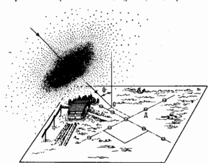
Рис. 1. Диск, образованный частицами широкого атмосферного ливня, приближается к установке под углом \theta ; Д — детекторы.
