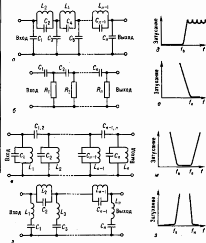
Рис. 1. Принципиальные схемы некоторых электрических фильтров на катушках индуктивности, конденсаторах и резисторах — нижних частот (а), верхних частот (б), полупропускающего (в), режекторного (г) и их частотные характеристики; L_1, L_2, \dots, L_n — катушки индуктивности, C_1, C_2, \dots, C_n — конденсаторы, R_1, R_2, \dots, R_n — резисторы, f — частота, f_n и f_n — граничные частоты.
