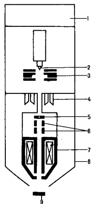
Рис. 6. Схема растрового оже-электронного микроскопа (РОЭМ): 1 — нонный насос; 2 — катод; 3 — трёхэлектродная электростатическая линза; 4 — многоканальный детектор; 5 — апертурная диафрагма объектива; 6 — двухъярусная отклоняющая система для развёртки электронного зонда; 7 — объектив; 8 — наружный электрод цилиндрического зеркального анализатора; 9 — обект.
