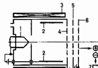
Рис. 2. Схема ионного двигателя с объемной ионизацией конструкции Г. Кауфмана: 1 — катод газоразрядной камеры; 2 — анод; 3 — магнитная катушка; 4 — эмиттирующий электрод; 5 — ускоряющий электрод; 6 — внешний электрод; 7 — нейтрализатор.
