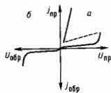
Рис. 2. ВАХ тиристора: а — при прямом смещении; б — при обратном смещении.
