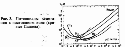
Рис. 3. Потенциалы зажигания в постоянном поле (кривые Пашена).
