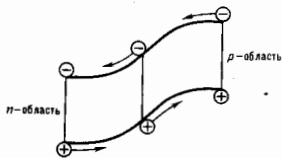
Рис. 1. Разделение возбуждаемых светом электронно-дырочных пар на r — n -переходе.
