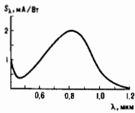
Рис. 3. Спектральная характеристика фотокатода на основе Ag—O—Cs.
