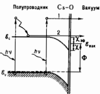
Рис. 3. Энергетическая схема приповерхностной области полупроводника с ОЭС. Стрелками показан выход в вакуум горячих (1) и термализованных (2) электронов.
