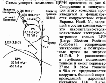
Рис. 6. Схема ускорительного комплекса ЦЕРН (Швейцария).
