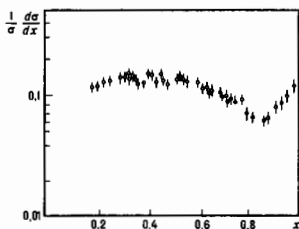
Рис. 2. Спектр лидирующих протонов в протон-протонных столкновениях при энергии 200 ГэВ; x —отношение энергии лидирующего протона к энергии первичного протона.
