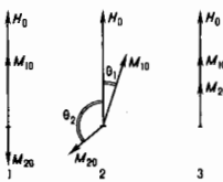
Рис. 1. Основные состояния изотропного двухподре- шоточного ферримагнетика: 1 — антипараллельное; 2 — неколлинеарное; 3 — параллельное.
