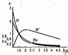
Рис. 2. Зависимость сечения фотоэффекта \sigma из основных состояний атомов H, He и иона H + от энергии фотонов. Масштабы осей кривых (в относительных единицах) выбраны так, чтобы \sigma = 1 при h\nu/I = 1,5 .
