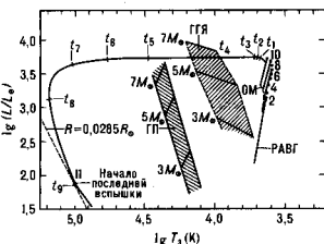
Рис. 4. Эволюционный трек звезды, превращающейся в белый карлик, с M = 0,6 M_{\odot} , начиная от РАВГ; начальный состав: X_{\text{H}} = 0,749, X_{\text{He}} = 0,25, X_2 = 0,001 . Точками даны положения звезды перед очередной тепловой вспышкой, указан ее номер. OM — обозначение минимума светимости при вспышке. Показаны треки звезды в области минимумов вспышек № 7, 9 и 10. Штрихованы участки на ГП и в области горения гелия в ядре (ГЯЯ), где даны приближенные эволюционные треки звезд с M = 3, 5, 7 M_{\odot} . Штриховая линия слева соответствует звезде потейного радиуса R = 0,0285 R_{\odot} .
