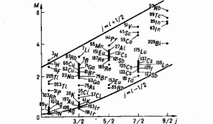
Рис. 2. Линия Шмидта для ядер с нечётным числом протонов Z.
