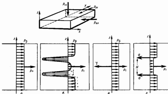
Рис. 3. Связь натяжения \gamma плёнки и межфазного натяжения \sigma в плёнке с компонентами обобщённого тензора гидростатического давления: \sigma —зависимость нормальной компоненты P_{zz} = P_\beta тензора давления от z ; \beta —зависимость тангенциальной компоненты P_i = P_{xx} = P_{yy} тензора давления от z ; \sigma —результат замены ТЖП на мембрану нулевой толщины; \sigma —результат замены ТЖП на две разделяющие поверхности.
