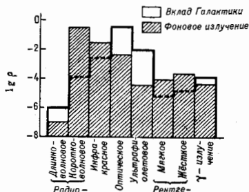
Рис. 2. Соотношение плотностей энергии фонового излучения Вселенной и диффузного излучения галактического происхождения; \rho в \text{эВ}/\text{см}^3 .
