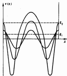
Рис. 3. Возмущение дна бесконечной прямоугольной потенциальной ямы, вызывающее опускание лишь уровня \epsilon_1 .
