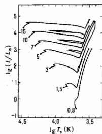
Рис. 2. Эволюционные треки звезд с начальным химическим составом X_H=0,7 , X_{He}=0,27 , X_Z (содержание элементов тяжелее гелия) = 0,03 от главной последовательности до гелиевой вспышки (для M=0,8 и 1,5 M_{\odot} ) или до возгорания углерода в центре (для M=3-15 M_{\odot} ). Цифры указывают массу звезды в M_{\odot} , точки соответствуют главной последовательности и моментам возгорания гелия и углерода в ядре.
