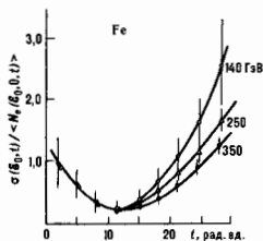
Рис. 4. Флуктуации электронно-фотонных каскадов при разных \theta_0 в Fe.
