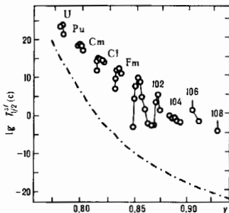
Рис. 1. Зависимость периода полураспада ядер относительно спонтанного деления T_{1/2}^{сп} от параметра деления y : штрих (шпунтир)—теория (модель жидкой капли), кружки—эксперимент.
