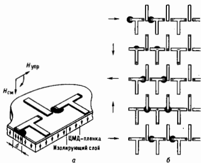
Рис. 7. а — Доменопроводящая ТГ-структура из пермалловых аппликаций; H_{норм} и H_{танг} — магнитные поля смещения и управления, d — диаметр ЦМД; б — схема перемещения ЦМД вдоль ТГ-структуры.
