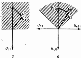
Рис. 1. Векторные диаграммы сигналов и помех для двухпозиционной (а) и четырехпозиционной (б) ФМН: U_{00}, U_{01}, U_{10}, U_{11} — векторы напряжений сигналов при передаче информационных символов 0 и 1 соответственно; U_{000}, U_{001}, U_{010}, U_{011}, U_{100}, U_{101}, U_{110}, U_{111} — векторы напряжений сигналов при передаче комбинаций из двух информационных символов 00, 01, 10, 11 соответственно; U_{\Sigma} — вектор напряжения помехи; U_{\Sigma} — вектор суммы напряжений сигналов и помехи. Штриховкой отмечены области, в которых сигнал с наложенной помехой может быть правильно принят приёмным устройством.
