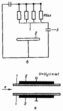
Рис. 3. Схемы возбуждения самостоятельного тлеющего разряда: a —импульсного, квазистационарного и стационарного разрядов в потоке газа, 1—анод, 2—штырь или узкие пластины для разряда в потоке газа, R_0 —балластные сопротивления; b —импульсного: 1—катодная пластина, 2—анод, 3—ёмкость самостоятельного разряда; U=U_0 \sin \omega t —электрические пластины, 2—электроды.
