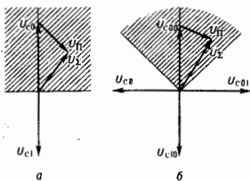
Рис. 1. Векторные диаграммы сигналов и помех для двухпозиционной (а) и четырехпозиционной (б) ФМН: U_{00}, U_{01}, U_{10}, U_{11} — векторы напряжений сигналов при передаче информационных символов 0 и 1 соответственно; U_{000}, U_{001}, U_{010}, U_{011}, U_{100}, U_{101}, U_{110}, U_{111} — векторы напряжений сигналов при передаче комбинаций из двух информационных символов 00, 01, 10, 11 соответственно; U_{\Sigma} — вектор напряжения помехи; U_{\Sigma} — вектор суммы напряжений сигналов и помехи. Штриховкой отмечены области, в которых сигнал с наложенной помехой может быть правильно принят приёмным устройством.
