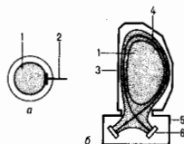
Рис. 2. Поперечный разрез плазмы круглого сечения (а) и вертикально вытянутого с образованием диверторной конфигурации (б): 1 — плазма; 2 — диаметр; 3 — стенка камеры; 4 — сепаратриса; 5 — диверторная камера; 6 — диверторные пластины.
