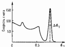
Рис. 4. Спектр импульсов от NaI(Tl) для E_\gamma = 661 КэВ.
