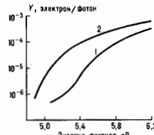
Рис. 2. Спектральная зависимость квантового выхода фототомиссии для сильнолегированного кремния n - и p -типов ( \phi_p = 1,1 эВ, \chi = 4 эВ); — n -тип, 2 — p -тип.
