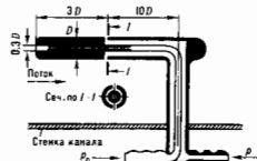
Рис. 1. Схема трубки Пито — Пранатля.
