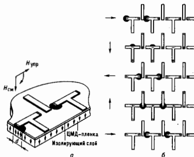
Рис. 7. а — Доменопроводящая ТГ-структура из пермалловых аппликаций; H_{нм} и H_{нр} — магнитные поля смещения и управления, d — диаметр ЦМД; б — схема перемещения ЦМД вдоль ТГ-структуры.
