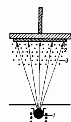
Рис. 3. Схема метода катодного осаждения: 1—источник; 2—подложка; 3—плазма.
