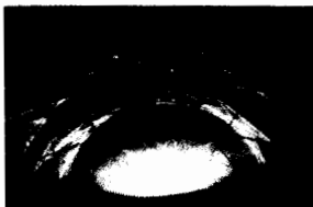
Рис. 2. Кикучи-электронограмма, полученная методом «ока отражения» (симметрично расположены тёмные и светлые кикучи-линии).
