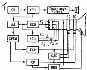
Рис. 9. Упрощённая функциональная схема цветного телевизионного приёмника.
