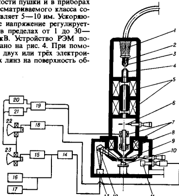
Рис. 4. Схема растрового электронного микроскопа (РЭМ): 1 — изолятор электронной пушки; 2 — V -образный термокатод; 3 — фокусирующий электрод; 4 — анод; 5 — конденсорные линзы; 6 — диафрагма; 7 — двухлучевая отклоняющая система; 8 — объект; 9 — апертурная диафрагма объекта; 10 — объект; 11 — детектор вторичных электронов; 12 — кристаллический спектрометр; 13 — пропорциональный счётчик; 14 — предварительный усилитель; 15 — блок усиления; 16, 17 — аппаратура для регистрации рентгеновского излучения; 18 — блок усиления; 19 — блок регулировки увеличения; 20, 21 — блоки горизонтальной и вертикальной развёртки; 22, 23 — электронно-лучевые трубки.
