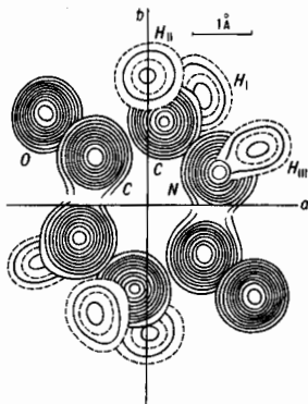
Рис. 3. Электрический потенциал молекулы диэктопиперазина в кристаллической структуре, полученных трёхмерным фурье-синтезом: a и b — оси симметрии молекулы. Ступени линий соответствуют положениям атомов.
