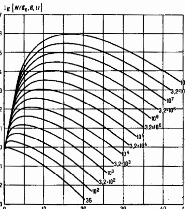
Рис. 1. Каскадные кривые в Рб для первичного фотона при различных первичных энергиях (в МэВ) и \delta = 0 .
