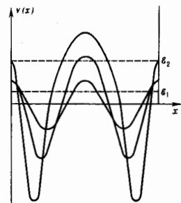
Рис. 3. Возмущение дна бесконечной прямоугольной потенциальной ямы, вызывающее опускание уровня \epsilon_2 .
