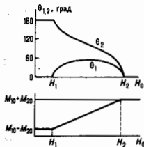
Рис. 2. Полевые зависимости углов между намагниченностями подрешёток и постоянным магнитным полем, а также суммарной постоянной намагнитченности двухподрежёточного ферримагнетика.
