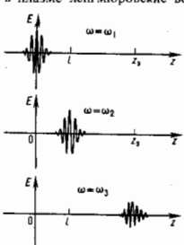
Схема возникновения пространственного плазменного эха второго порядка.
