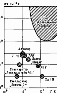
Рис. 3. Параметры, достигнутые на различных установках для изучения проблемы управляемого термоядерного синтеза к 1991. Т-10 — установка токамак Института атомной энергии имени И. В. Курчатова (СССР); ПЛТ — установка токамак Принстонской лаборатории (США); Агрегатор — установка токамак Массачусетского технологического института (США); ТФР — установка токамак в Фонтене-о-Роз (Франция); 2 ХПВ — открытая ловушка Ливерморской лаборатории (США); лазер «Шива» (Ливерморская лаборатория, США); стелларатор «Ливень» (ФИАН, Москва); стелларатор «Венделштерн УП» (Гарнинг, ФРГ).
