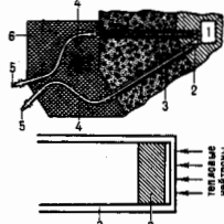
Рис. 2. Получение ультрахолодных нейтронов (горизонтальные каналы): 1—активная зона реактора; 2—конвертор внутри нейтронвода; 3, 4—изогнутые участки нейтронвода; 5—детектор нейтронов; 6—защита. Внизу показано расположение конвертора в нейтронводе.
