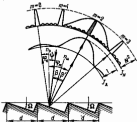
Рис. 1. Схематическое изображение функций J_n , J_0 и их произведения J_n J_0 = 1/N^2 (заштриховано); направления \phi_n на центр дифракционного максимума функции J_n совпадает с интерференционным максимумом функции J_0 при m=2 ; n_x — нормаль к плоскости эшелетта, n_m — нормаль к грани штриха.
