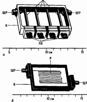
Рис. 3. Электрические фильтры — гребенчатый (а) и шпильный (б); ШР — штенсельный резань, Р — резонаторы, ПК — построенные конденсаторы, К — корпус (со снятой крышкой).
