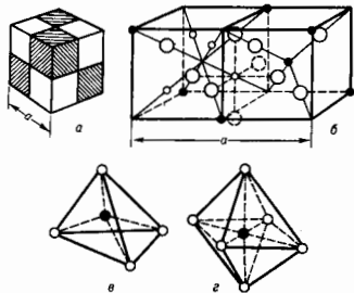
Рис. 1. Кристаллическая структура ферритов-шпинелей: а — схематическое изображение элементарной ячейки шпинельной структуры, разделённой на 8 октаэдов; б — расположение ионов в смежных октаэдах ячейки; белые кружки — анионы O^{2-} , образующие остов решетки, чёрные — катионы в октаэдрических и тетраэдрических позициях; в — катион в тетраэдрическом окружении; г — катион в октаэдрическом окружении.
