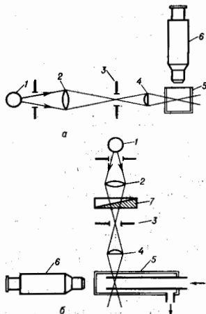
Принципальные схемы щелевого (а) и поточного (б) ультрафиолетового спектроскопа.
