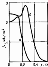
Рис. 2. Распределение плотности тока на катоде в тлеющем разряде в азоте (расчёт) при давлении p=5 тор, межэлектродном расстоянии 1 см; a —при токе I=0,75 мА, b —при I=1,5 мА.
