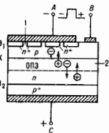
Рис. 1. Четырёхслойная p-n-p-n -структура тиристора: АС—основная цепь; АВ—цепь управления; I_1 —шунтирующие каналы; 2—ОПЗ коллектора.
