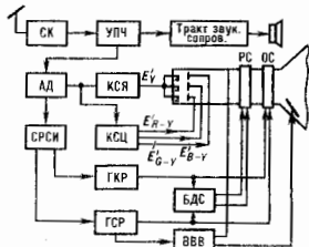
Рис. 9. Упрощенная функциональная схема цветного телеприемника.
