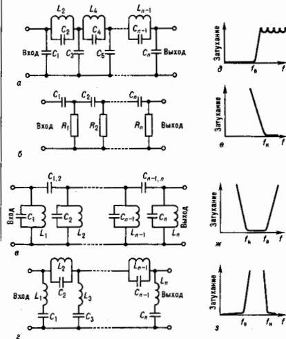
Рис. 1. Принципиальные схемы некоторых электрических фильтров на катушках индуктивности, конденсаторах и резисторах — нижних частот (а), верхних частот (б), полосу-пропускающего (в), режктерного (г) и их частотные характеристики; L_1, L_2, \dots, L_n — катушки индуктивности, C_1, C_2, \dots, C_n — конденсаторы, R_1, R_2, \dots, R_n — резисторы, f — частота, f_n и f_{n-1} — граничные частоты.
