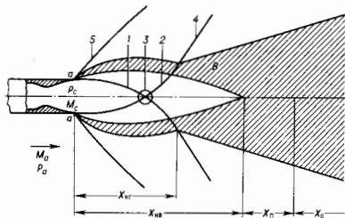
Рис. 2. Сверхзвуковая нерасчётная струя в сверхзвуковом сплунном потоке.
