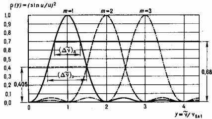
Рис. 4. График коэффициента отражения \rho(y) = (\sin u / u)^2 , y = \sqrt{v} / v_{0.1} ; (\Delta v)_z — область дисперсии и (\Delta v)_y — область энергетической эффективности, не зависящие от m .
