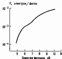
Рис. 1. Спектральная зависимость квантового выхода фототомиссии для чистой поверхности Cu.
