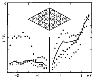
Рис. 4. Спектры туннельной проводимости dI/dV в функции напряжения менее острым и образом, полученные для Si(111)-(7x7) поверхности. Сплошная линия — спектр, усреднённый по элементарной ячейке (врезка), локальные спектры даны при расположении острого кончика (квадратики) и в промежутках между ними (точки и крестики) соответствующим позициям, помеченным теми же символами на схеме элементарной ячейки.
