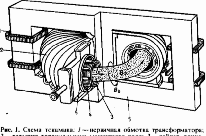
Рис. 1. Схема токамака: 1 — первичная обмотка трансформатора; 2 — катушки тороидального магнитного поля; 3 — линзер, тонкостенная внутренняя камера для выравнивания тороидального электрического поля; 4 — катушки поперечного магнитного поля; 5 — вакуумная камера; 6 — железный сердечник (магнитопровод).
