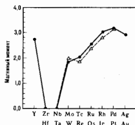
Рис. 6. Атомный магнитный момент в единицах \mu_B на атом Fe в окружении атомов переходных 4d(0) и 5d(-\Delta) металлов в гипотетическом сплаве OLCk FeT; (по теории Жакардино—Уокера).
