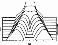
Рис. 1. Изменение плотности состояний \rho(\omega) с ростом параметра U (выражение роста указано стрелкой) в приближении «Хаббард-3» для простой кубической решётки.
