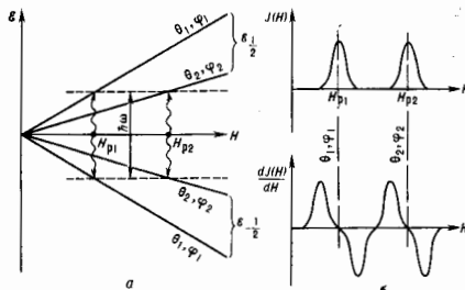
Рис. 1. Электронный парамагнитный резонанс: а—парамагнитная частица со спином S = 1/2 , помещенная во внешнее магнитное поле, имеет два подуровня ( \epsilon_{1,2} и \epsilon_{-1,2} ), каждый из которых изменяется пропорционально полю H и зависит от его ориентации по отношению к кристаллографическим осям, задаваемой углами \theta и \phi . При резонансных значениях магнитного поля H_{P1} и H_{P2} (углы \theta_1, \phi_1 и \theta_2, \phi_2 ) разность \epsilon_{1,2} - \epsilon_{-1,2} становится равной кванту энергии \hbar\omega СВЧ-излучения. При этом в спектре поглощения (б) наблюдаются характерные всплески вблизи H_{P1} и H_{P2} (приведены сигнал поглощения и его производная).
