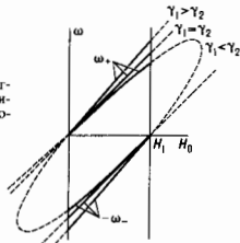
Рис. 4. Частоты ферримагнитного резонанса и антипараллельного основного состояния.
