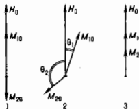
Рис. 1. Основные состояния изотропного двухподрежёточного ферримагнетика: 1 — антипараллельное; 2 — неколлинеарное; 3 — параллельное.
