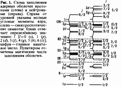
Рис. 1. Схема заполнения ядерных оболочек протонами (слева) и нейтронами (справа). Справа от уровней указаны полные угловые моменты ядра; слева — спектроскопические символы: буква отвечает определённому значению l ( l = 0 (s), 1 (p), 2 (d), 3 (f), 4 (g), 5 (h), 6 (i) ); цифра — главное квантовое число. Пунктиром отмечены магические числа заполнения оболочек.
