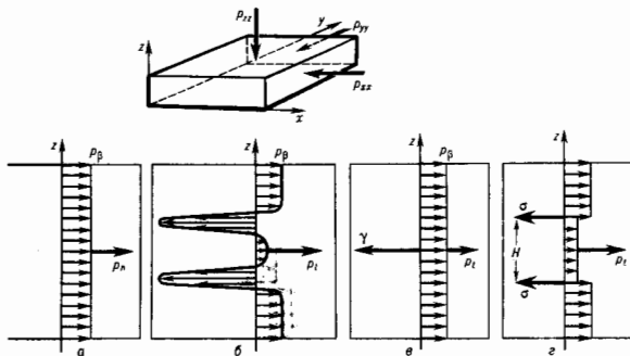
Рис. 3. Связь натяжения \gamma плёнки и межфазного натяжения \sigma в плёнке с компонентами обобщённого тензора гидростатического давления: \sigma —зависимость нормальной компоненты P_{zz} = P_\beta тензора давления от z ; \sigma —зависимость тангенциальной компоненты P_i = P_{xx} = P_{yy} тензора давления от z ; \sigma —результат замены ТЖП на мембрану нулевой толщины; \sigma —результат замены ТЖП на две разделяющие поверхности.
