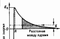
Рис. 1. Потенциальная энергия междуядерного взаимодействия как функция расстояния между ядрами; \phi — относительная энергия ядер, отвечающая глубоко подбарьерному прохождению. Штриховкой показано «срезание» барьера отталкивания на борковом радиусе a , отрицательного мюона в кулоновском поле одного из сталкивающихся ядер, лежащее в основе явления \mu -катализа.
