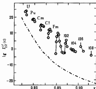
Рис. 1. Зависимость периода полураспада ядер относительно спонтанного деления T_{1/2}^{sp} от параметра деления y : штрих (шпунтир)—теория (модель жидкой капли), кружки—эксперимент.
