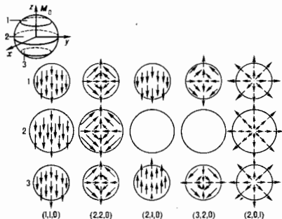
Рис. 2. Распределения перемешной намагнитченности M_1 в трех плоскостях z = \text{const} в некоторый момент времени.
