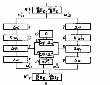
Рис. 2. Схема дифференциального ядерного гироскопа на базе четырёх СГ с двумя ячейками на изотопах ртути ^{199}\text{Hg}, ^{201}\text{Hg} : 1, 2—фильтры на частотах \omega_{L1}, \omega_{L2} ; 3, 4—умножители частоты K\omega ; 5, 6—фильтры на частотах \omega_{L1}, \omega_{L2} ; 7, 8—датчики разностей фаз \Delta\varphi_1 (между частотами \omega_{L1} и K\omega_{L1}^I ) и \Delta\varphi_2 (между частотами \omega_{L2} и K\omega_{L2}^I ); 9—схема суммирования разностей фаз \Delta\varphi_1 + \Delta\varphi_2 ; 10—схема управления полем H^I ; 11—схема вычитания разностей фаз \Delta\varphi_1 - \Delta\varphi_2 ; 12—система регистрации и обработки выходного сигнала.
