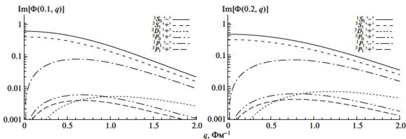
Рис. 2. То же, что и на рис. 1, но для мнимой части амплитуд.
