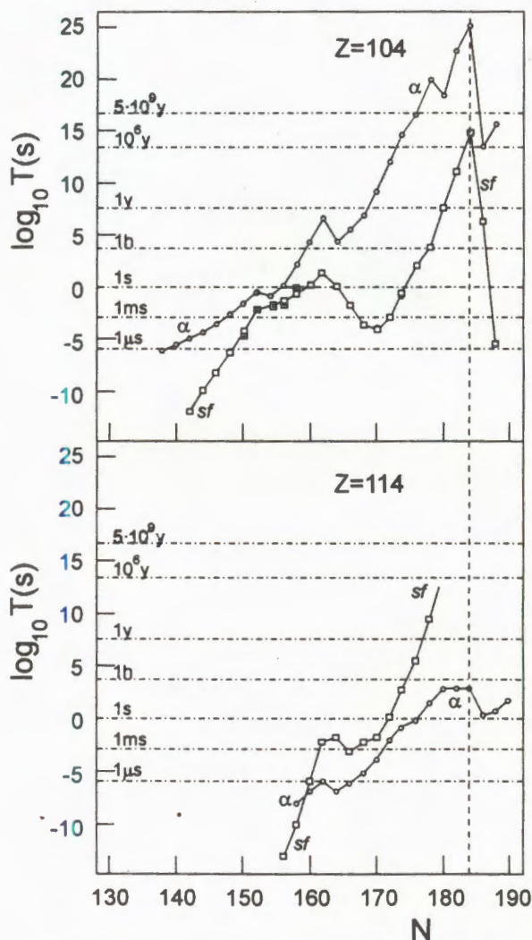
Рис.2. Парциальные периоды спонтанного деления (квадраты) и \alpha -распада (кружки) изотопов 104 и 114 элементов. Открытые символы — расчет [26,27], черные точки и квадраты — экспериментальные значения, полученные для изотопов с Z = 104 . Сплошные линии проведены через расчетные значения
