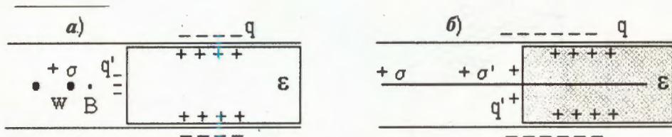
Рис.12. Схема пропорциональной камеры вблизи диэлектрической рамки \epsilon , \sigma — линейная плотность заряда проволоки, q — поверхностная плотность зарядов катода, q' — поверхностная плотность зарядов рамки за счет поляризации диэлектрика. Сечение камеры плоскостью, перпендикулярной плоскости проволок (а), w — проволока. Сечение камеры вдоль проволоки (б), \sigma' — линейная плотность заряда проволоки у ее конца
