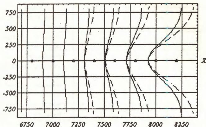
Рис.5. Конфигурация элементарных ячеек камеры из 83 проволок в медианном сечении на одном из ее краев в районе 8 крайних проволок. Видно изменение формы прямоугольных ячеек камеры. Сплошными кривыми показаны границы между ячейками для камеры, у которой диаметры 4-х крайних проволок увеличены. Пунктирные кривые — границы ячеек камеры с проволоками равных диаметров. По каждой из осей X и Y 100 делений соответствуют 1 мм.
