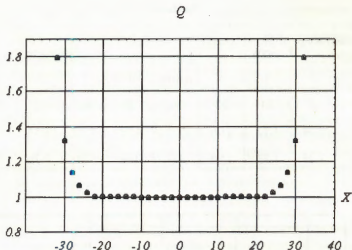
Рис.4. Величина заряда на проволоке в зависимости от ее положения для камеры из 33 проволок. Диаметры всех проволок равны 20 мкм за исключением 4-х крайних, равных 25, 30, 40 и 50 мкм
