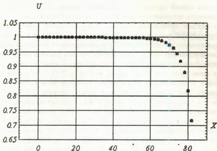
Рис.1. Разность потенциалов U проволочка—катод в зависимости от положения проволочки. Линейные плотности зарядов всех проволочек одинаковы. Диаметры всех проволочек одинаковы и равны 20 мкм. X = 0 соответствует центру камеры
