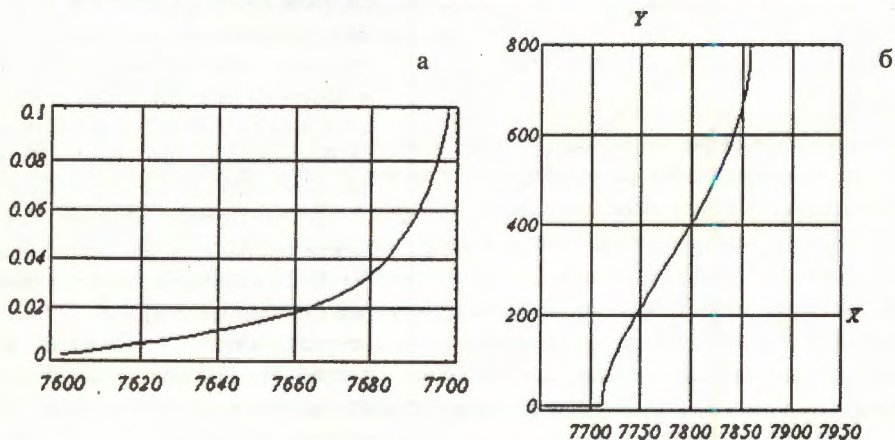
Рис.6. Линия электрического поля в медианной плоскости, начинающаяся на 4-й от края проволоке. Линия проходит через точку, расположенную посередине между 4-й и 3-й крайними проволоками по оси X и смещенную на 1 мкм по оси Y. а — ее начальный участок, б — вся линия поля от проволоки до катодной плоскости.
