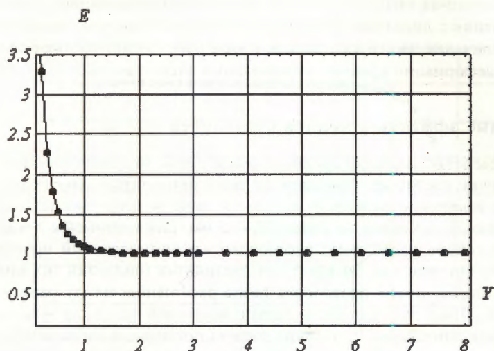
Рис.8. Изменение электрического поля по линии, проходящей через центр одной из проволок камеры вдоль направления, перпендикулярного плоскости проволок
