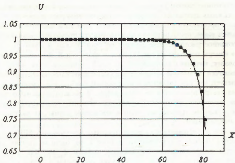
Рис.10. Разность потенциалов U проволочка — катод вдоль диагонали камеры. Линейная плотность заряда вдоль каждой проволочки постоянна, линейная плотность заряда при переходе от проволочки к проволочке соответствует рис.2
