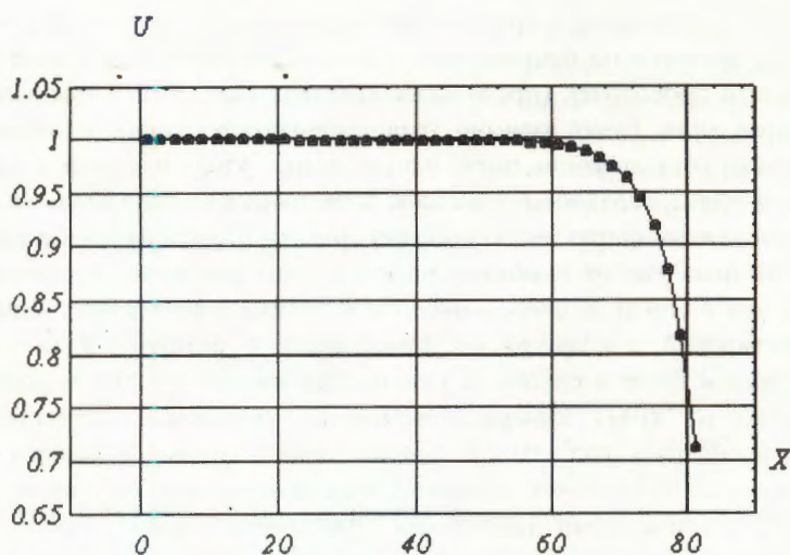
Рис.9. Разность потенциалов U провололка — катод вдоль центральной провололки камеры. Линейная плотность заряда вдоль всей провололки одинакова, линейная плотность заряда на всех провололках одинакова. X = 0 соответствует центру камеры
