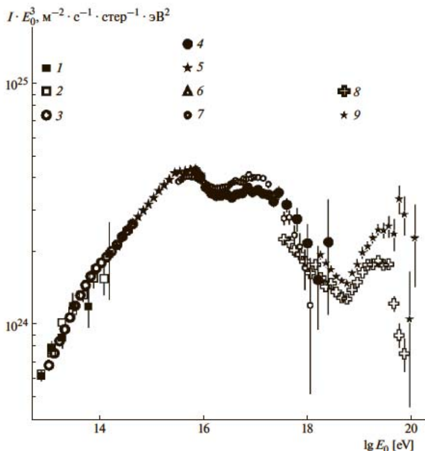
Рис. 2. Сравнение с данными других работ: 1 – АТИК2, 2 – НУКЛОН (КЛЕМ), 3 – HAWC, 4 – Тунка-133, 5 – TAIGA-HiSCORE, 6 – KASCADE-Grande, 7 – IceTOP, 8 – TA, 9 – PAO.
