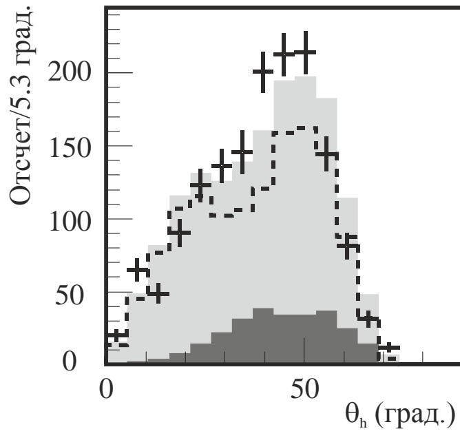
Рис. 6. Экспериментальное распределение по гипер-углу \vartheta_h , полученное в реакции {}^4\text{He}({}^6\text{He}, 2\alpha)2n при условии P_{2n}^Z > 80 МэВ/с. Обозначения объясняются в подписи к рис. 5.
