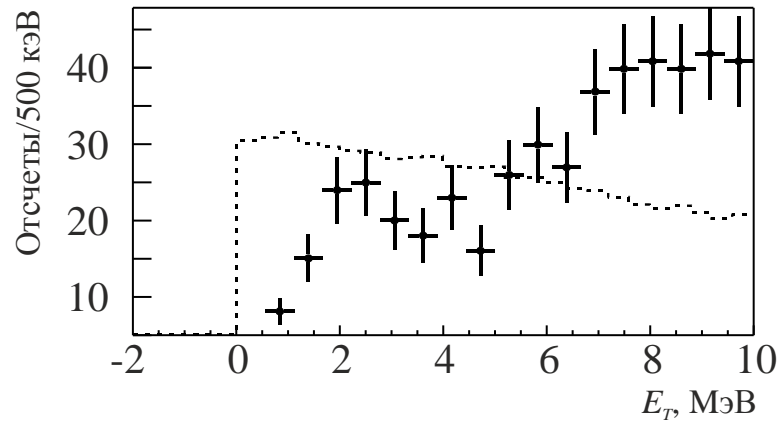
Рис. 1. Спектр недостающей массы ^{10}\text{He} . Пунктирная гистограмма показывает зависимость эффективности регистрации от энергии ^{10}\text{He} .
