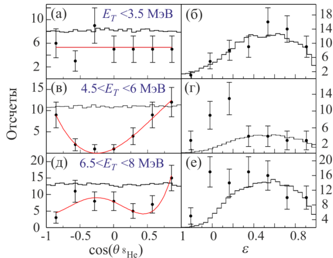
Рис. 2. Угловые распределения (три левые панели) и распределение по \varepsilon (три правые панели), полученные для различных диапазонов возбуждения ^{10}\text{He} . Гистограммы и красные линии на левых панелях (а), (в) и (д) показывают, соответственно, эффективность регистрации и результаты подгонки спектров. Гистограммы на правых панелях (б), (г) и (е) получены в результате симуляции трехфазового объема.
