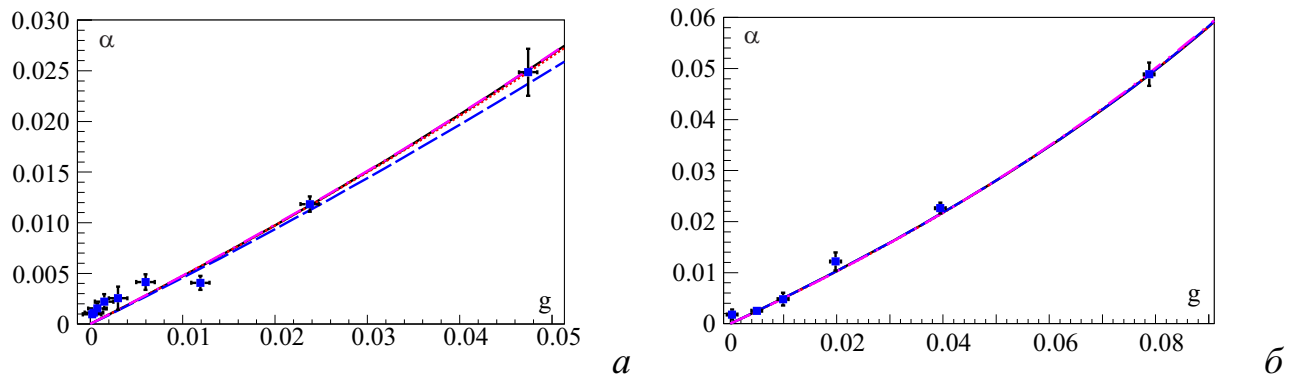
Рис. 2. Расчетные декременты затухания и результаты измерений горизонтальных (а) и вертикальных (б) когерентных поперечных колебаний пучка протонов с энергией 3.5 ТэВ в LHC [5, 15]
