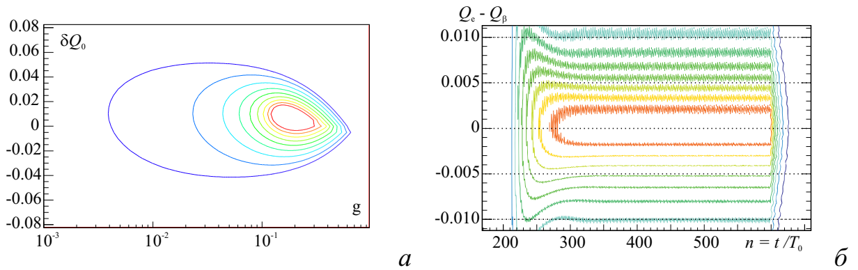
Рис. 3. Карты: (а) изолиний \alpha(g, \delta Q_0) = \alpha_l [4] и (б) изоамплитуд a_c(n, Q_e - Q_\beta) = a_l [5]
