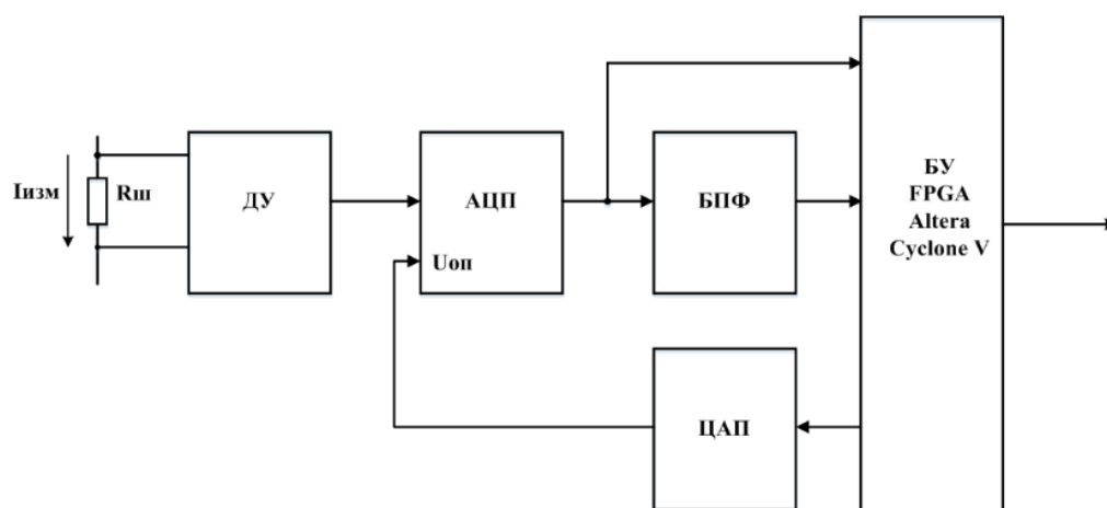
Рис. 1. Структурная схема измерительного преобразователя тока
