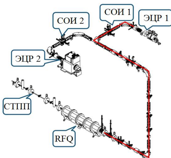
Рис. 11. Общий вид системы инжекции.
