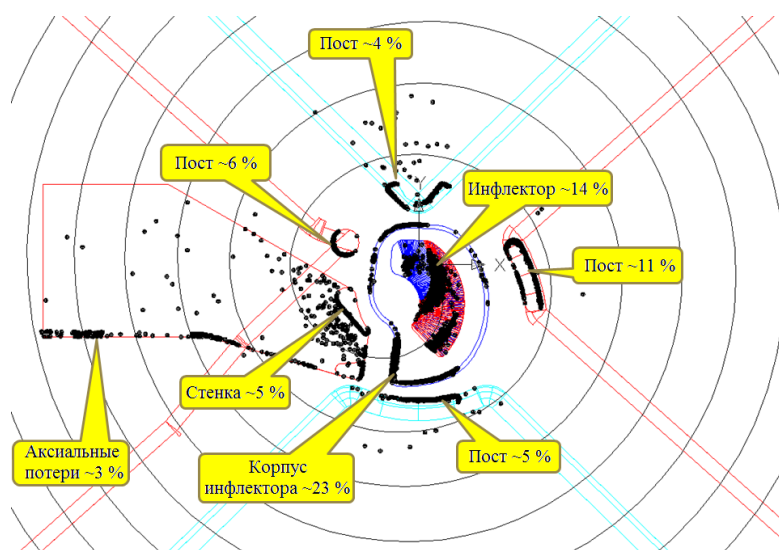
Рис. 10. Распределение потерянных частиц в центральной области циклотрона.
