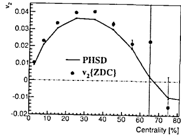
Рис. 7: Зависимость эллиптического потока v_2 от центральности ( AuAu@9ГэВ ).
