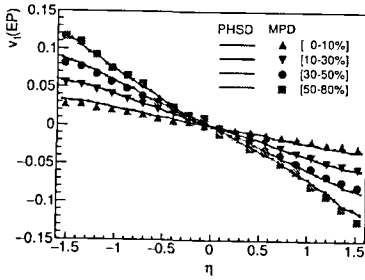
Рис. 6: Зависимость прямого потока v_1 от псевдобыстроты ( AuAu@9ГэВ ).
