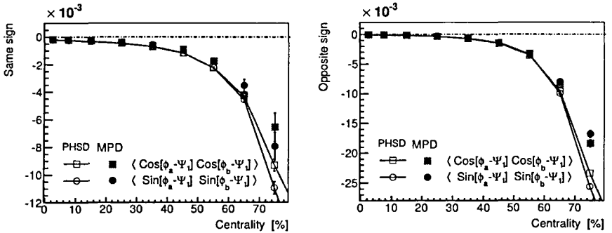
Рис. 10: Компоненты азимутального углового коррелятора для одноименно (слева) и разноименно (справа) заряженных частиц ( AuAu@9ГЭВВ ).
