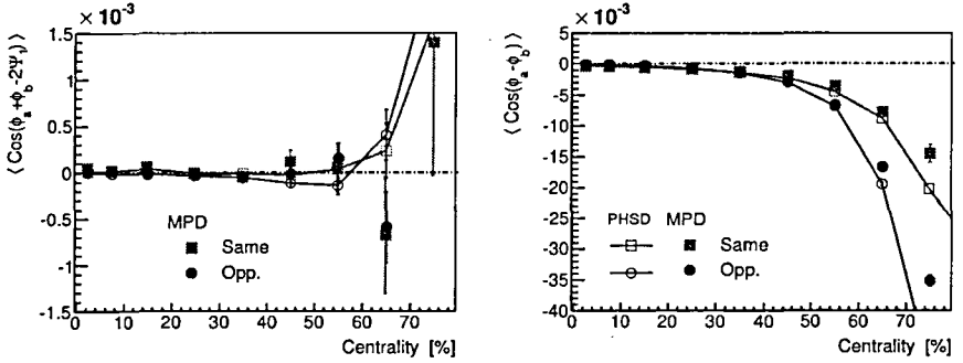
Рис. 9: Азимутальные угловые корреляции ( AuAu@9ГЭВ )
