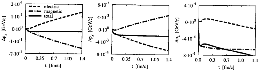
Рис. 3: Зависимость от времени приращения импульса \Delta p для вперед-летищих положительно заряженных мезонов рожденных в AuAu столкновении при энергии \sqrt{s_{NN}} = 200 ГэВ и прицельным параметром b = 10 фм в HSD модели.
