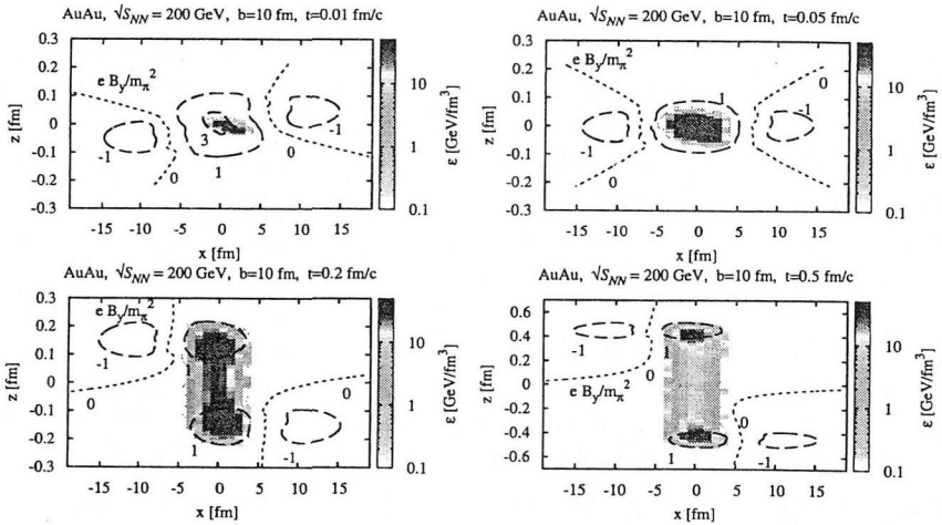
Рис. 2: Пространственная взаимосвязь между величиной магнитного поля и плотностью энергии для AuAu столкновения при энергии \sqrt{s_{NN}} = 200 ГэВ и прицельным параметром b = 10 фм. Уровни магнитного поля показаны пунктирной линией, в то время как плотность энергии показана цветом.
