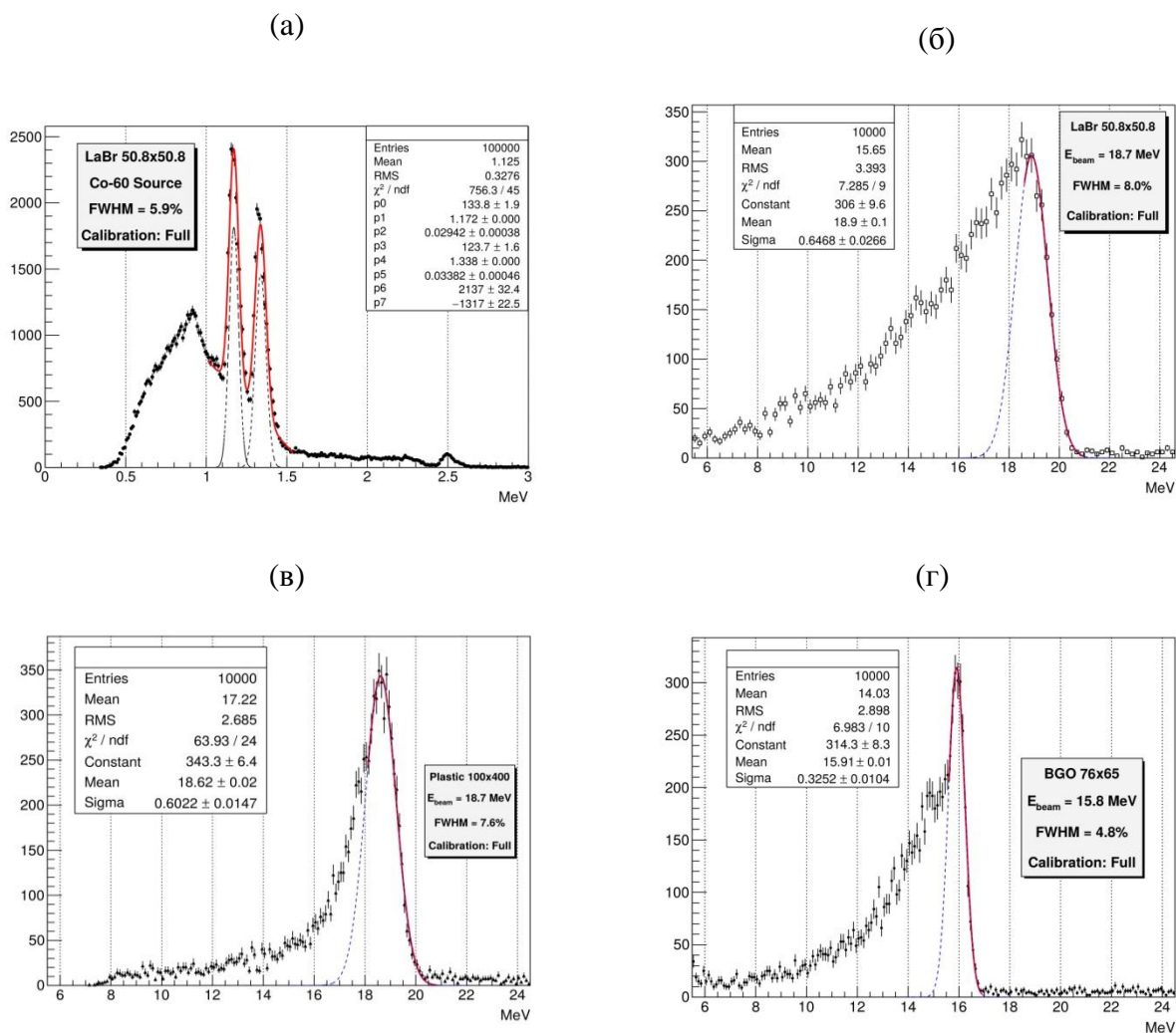
Рисунок 1 – \gamma -спектр ^{60}\text{Co} , измеренный детектором LaBr (а) и спектры электронов ускорителя ЛИНАК-200: энергией 18,7 МэВ, измеренный детектором LaBr (б); энергией 18,7 МэВ, измеренный пластиковым сцинтиллятором (в); энергией 15,8 МэВ, измеренный детектором BGO (г)
