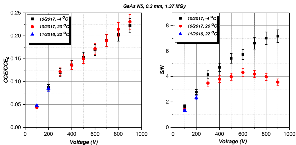
Рисунок 7 – Зависимости CSE и соотношения сигнал-шум (S/N) от U_{bias} для сенсора GaAs:Cr N5, облученного до 1,37 МГр, измеренные при различных температурах
