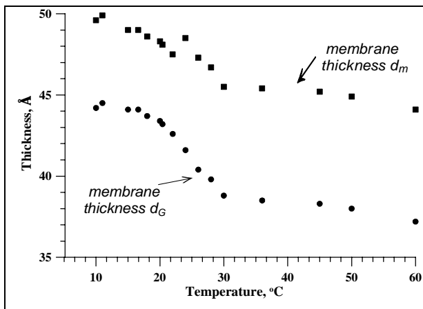
Рисунок 6. Зависимость толщины мембраны ДМФХ d_G и толщины мембраны d_m от температуры. Величина d_G определена из спектра МУРН в приближении Гинье. Величина d_m рассчитывается на основе поправок, сделанных по результатам расчетов на основе РФФ метода [10].
