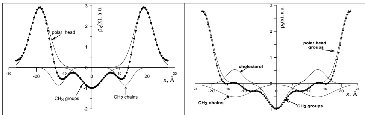
Рисунок 8. Распределение плотности длины рассеяния нейтрона \rho_s(x) в многослойной мембране ДМФХ при RH = 60\% , T=32^\circ\text{C} и 8\% содержании \text{D}_2\text{O} (точки) и расчетные кривые (сплошная линия). Стрелки показывают положение трех молекулярных групп: \text{CH}_3 группы, \text{CH}_2 цепочки и группы полярных голов.
