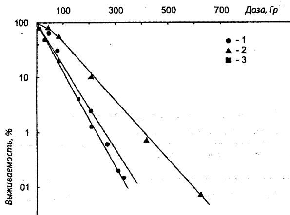
Рис. 3. Кривые выживания клеток бактерий E. coli K-12 штаммов АВ 1157 (1), BL 1114 (2), АВ 2463 (3), облученных \alpha -частицами.
