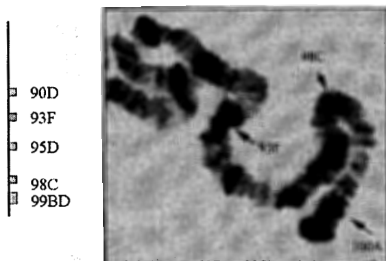
Рис. 3. Локализация ретротранспозона mdg1 (сайты 93F и 98C) и hobo -транспозона на фрагменте третьей хромосомы линии u sn bw sp Drosophila melanogaster по данным in silico (1992 г., слева) и FISH (2005 г., справа).
