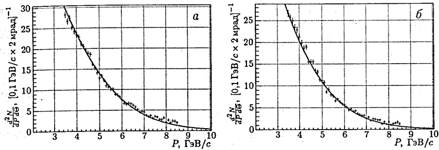
Рис. 4. Форма распределения \frac{d^2N}{dP d\Theta} (p + Ni \rightarrow \pi^+\pi^- X) при фиксированных полярных углах вылета \pi^+\pi^- -пары \Theta : 0,089 (а), 0,108 (б) /9/
