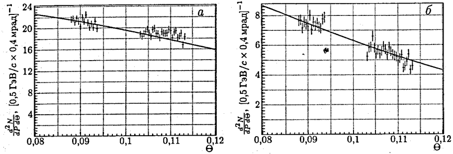
Рис. 5. Форма распределения \frac{d^2N}{dP d\Theta} (p + Ni \rightarrow \pi^+\pi^- X) при фиксированных импульсах \pi^+\pi^- -пары P : 4,2 ГэВ/с (а), 6 ГэВ/с (б) /9/
