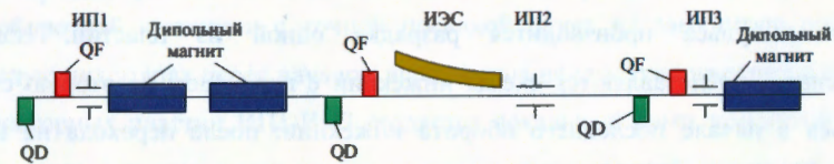
Рис. 1. Схема размещения элементов системы инжекции пучка в Бустер. Обозначения: QF, QD – фокусирующие и дефокусирующие квадрупольные линзы [3].
