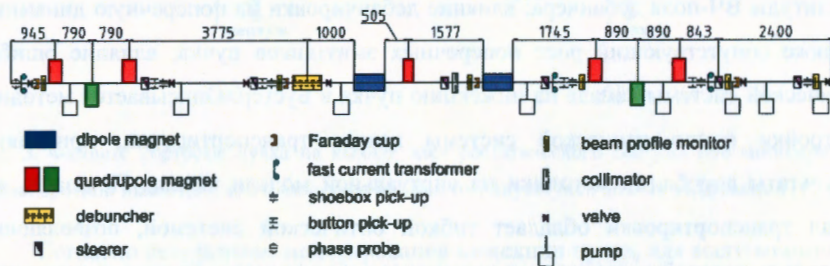
Рис. 4. Компоновка канала транспортировки пучка ЛУТИ-Бустер [17].
