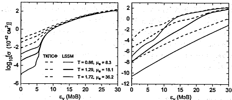
Рис. 11. Сравнение ТКПСФ и LSSM сечений реакции ^{56}\text{Fe}(\nu_e, e^-) . Сечения показаны как без учёта (рисунок слева), так и с учётом (рисунок справа) блокировки вылетающих электронов. Температура T и химический потенциал \mu_e указаны в МэВ.
