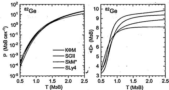
Рис. 10. Скорость потери энергии (слева) и средняя энергия излучённой \nu\bar{\nu} -пары (справа) ядром ^{82}\text{Ge} как функции температуры.
