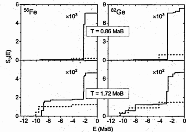
Рис. 5. Бегущие суммы для экзоэнергетической ( E < 0 ) компоненты \Gamma T_0 силовой функции, рассчитанные с использованием (штриховые линии) и без использования гипотезы Бринка-Акселя. На каждом рисунке приведены масштабирующие множители.
