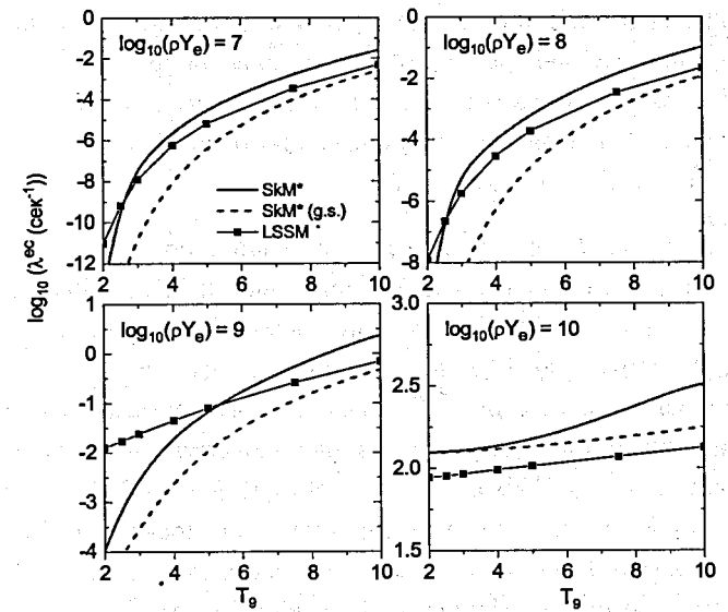
Рис. 2. Скорости e^- -захвата ядром ^{56}\text{Fe} , рассчитанные с учётом и без учёта (g.s.) влияния тепловых эффектов на силовую функцию G_{T+} переходов. Скорости показаны как функция температуры ( 1 T_9 = 10^9 К) для нескольких значений плотности \rho Y_e (в г/см 3 ). Результаты ТКПСФ вычислений с параметризацией сил Скирма \text{SkM}^* сравниваются с результатами LSSM.
