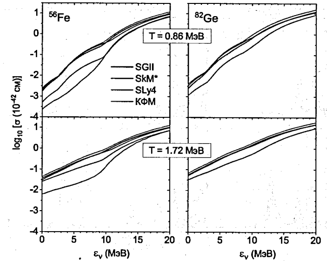
Рис. 7. Сечение неупругого рассеяния нейтрино на ^{56}\text{Fe} и ^{82}\text{Ge} при T = 0.86 \text{ МэВ} и T = 1.72 \text{ МэВ} . Сравниваются сечения рассчитанные в ТКПСФ с гамильтонианом КФМ и с различными параметризациями сил Скирма. Для ^{56}\text{Fe} приведены сечения, рассчитанные в LSSM (чёрная линия).
