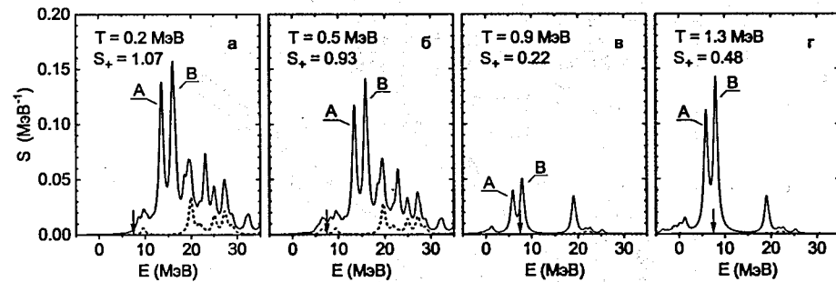
Рис. 3. Распределение силы разрешённых ( 0^+ и 1^+ ) p \rightarrow n переходов в 76 Ge при различных значениях температуры T . Вклад 0^+ переходов показан штриховой линией. S_+ обозначает полную силу переходов. Стрелка указывает на положение порога e^- -захвата при T = 0 ( Q = 7.52 МэВ). Пики, обусловленные одночастичными резонансными ГТ + переходами 1f_{7/2}^p \rightarrow 1f_{5/2}^n , 1g_{9/2}^p \rightarrow 1g_{7/2}^n , помечены соответственно символами А и В.
