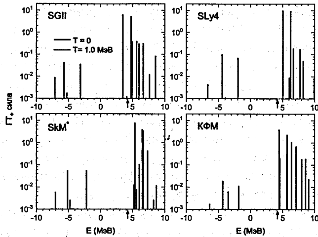
Рис. 1. Силовая функция G_{T+} переходов в ^{56}\text{Fe} для двух значений температуры. Результаты самосогласованных ТКПСФ расчётов с силами Скирма сравниваются с результатами, полученными с использованием гамильтониана КФМ. Стрелка указывает положение порога e^- -захвата при T = 0 ( Q = 4.21 МэВ).
