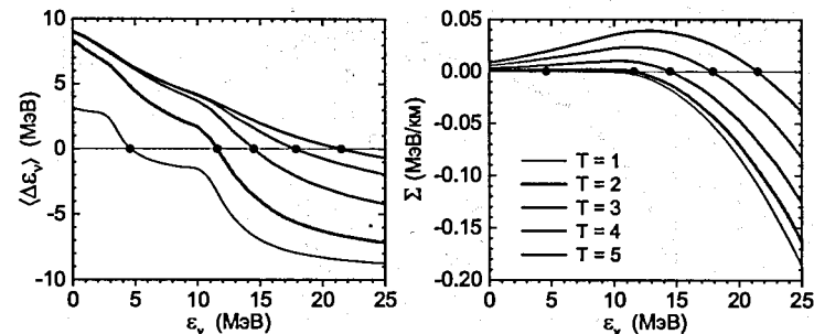
Рис. 9. Слева: среднее изменение энергии нейтрино при неупругом рассеянии на ^{56}\text{Fe} как функция энергии налетающего нейтрино \epsilon_\nu для нескольких значений температуры T (в МэВ). Справа: тормозная способность вещества состоящего из ^{56}\text{Fe} при плотности \rho = 10^{12} г/см 3 как функция энергии нейтрино для нескольких значений температуры. Закрашенные кружки отмечают значения (T, \epsilon_\nu) , при которых происходит смена режима рассеяния: (T, \epsilon_\nu) = (1, 4.6), (2, 11.6), (3, 14.5), (4, 17.9), (5, 21.5) .
