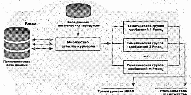
Рис.2. Схема второго уровня «Фильтрация и рубрикация сообщений»
