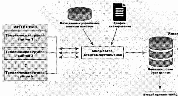
Рис.1. Схема первого уровня «Сбор информации с внешних сетевых источников»
