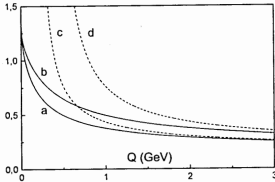
Рис. 2: Поведение инвариантного аналитического заряда \bar{\alpha}_{\text{an}}(Q^2) : (a) - для \Lambda = 200 МэВ, (b) - для \Lambda = 400 МэВ. Кривые (c) и (d) соответствуют теории возмущений для тех же значений параметра \Lambda .
