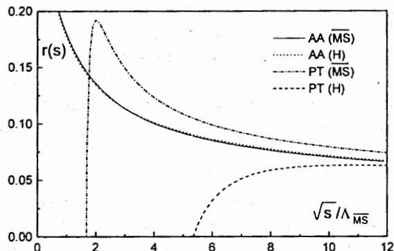
Рис. 3: График функции r(s) , вычисленной в теории возмущений (PT) и в аналитическом подходе (AA) для двух схем перенормировки H и MS.
