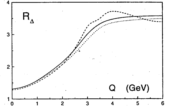
Рис. 1: График функции R_\Delta(s = Q^2) для \Delta = 3 \text{ ГэВ}^2 . Сплошная кривая соответствует ВТВ результату. Экспериментальная кривая обозначена пунктиром, а результат оптимизации третьего порядка пертурбативного разложения, выполненный в соответствии с принципом минимальной чувствительности, обозначен точками.
