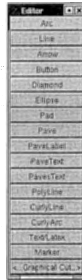
Рис. 4: Графический редактор
