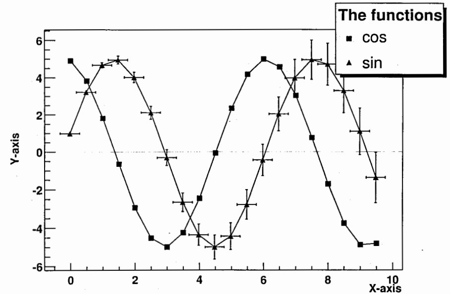
Рис. 5: Граф
