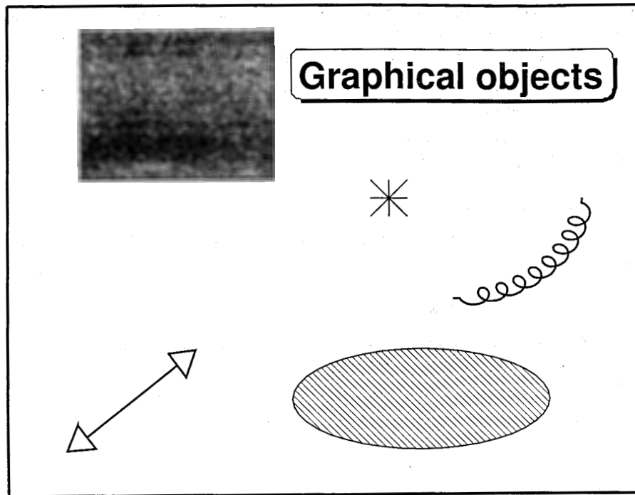
Рис. 3: Графические примитивы
