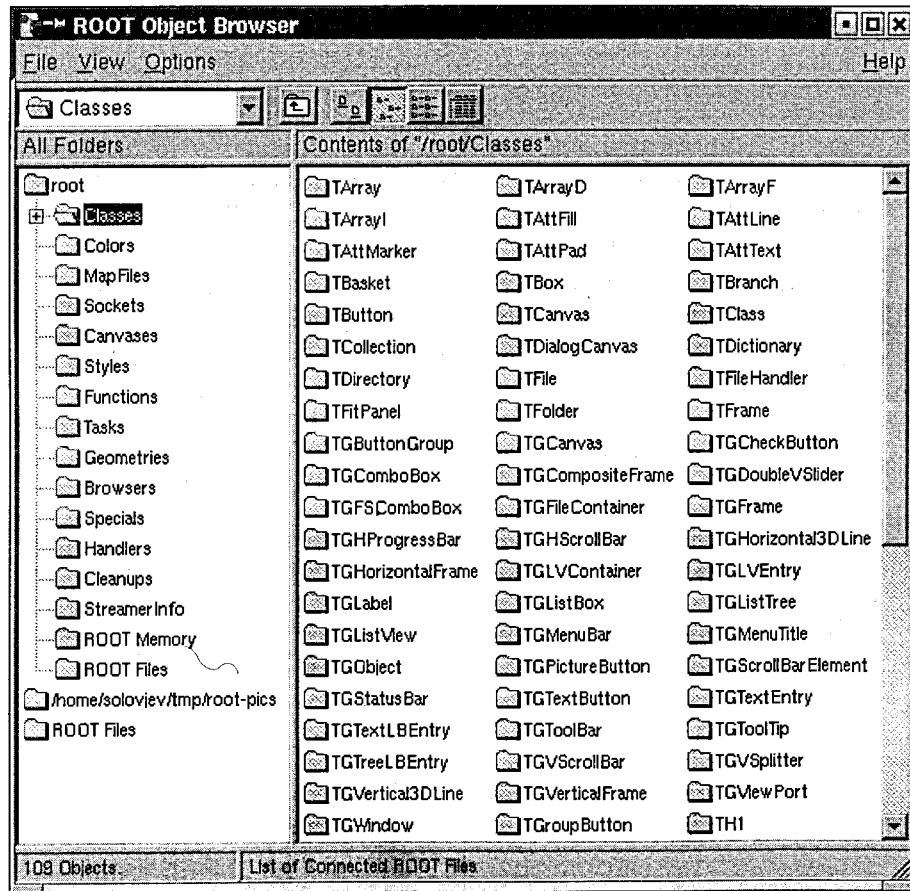
Рис. 1: Окно просмотра
