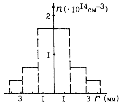
Рис. 5. Зависимость плотности лазерной плазмы от расстояния до оси вертикального канала для основной части плазменного сгустка.
