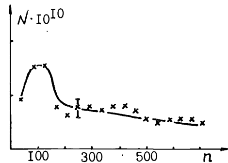
Рис. 10. Зависимость среднего количества N ускоренных ионов \text{C}_{12}^{3+} за один импульс лазера от числа выстрелов n по одной точке мишени для L = 3,3 см.
