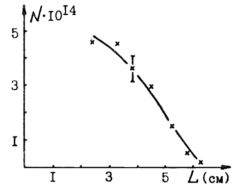
Рис. 6. Зависимость количества ионов N , проходящих около эмиссионной щели и регистрируемых зондом диаметром 3 мм, от расстояния L .
