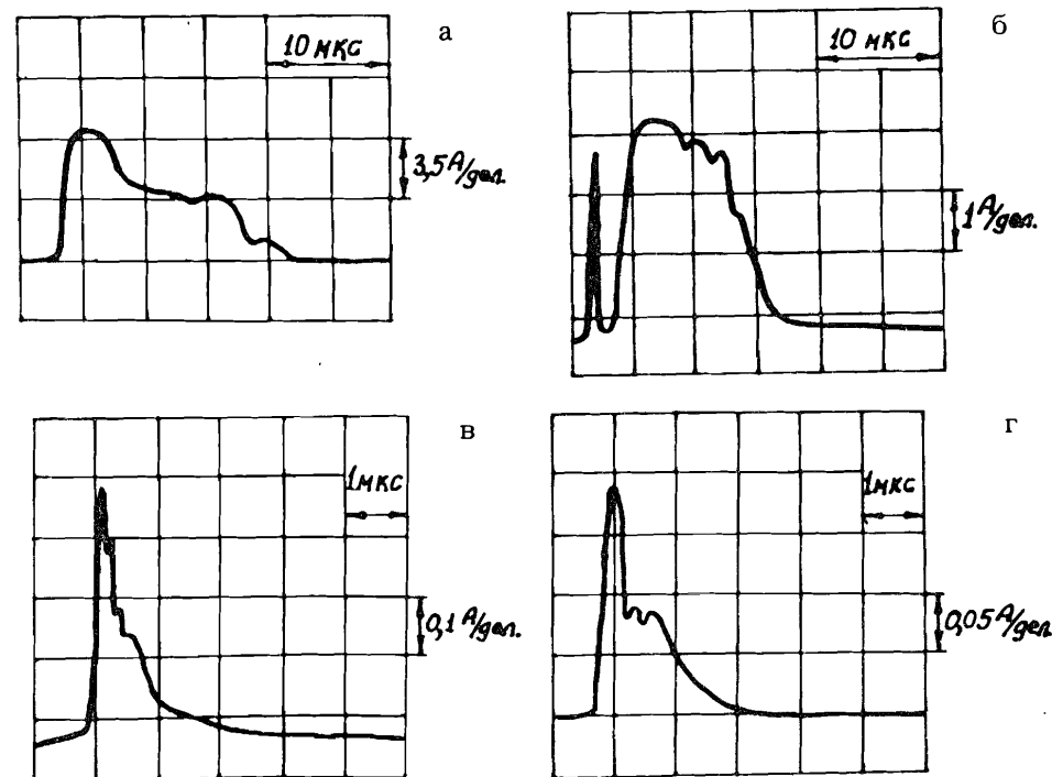
Рис. 4. Характерные осциллограммы сигналов с центрального зонда на различных расстояниях L в отсутствие и при наложении магнитного поля. H_{\text{макс}} : а — L = 2,4 см; б — L = 5 см; H = 0 : в — L = 5 см; г — L = 9,5 см.
