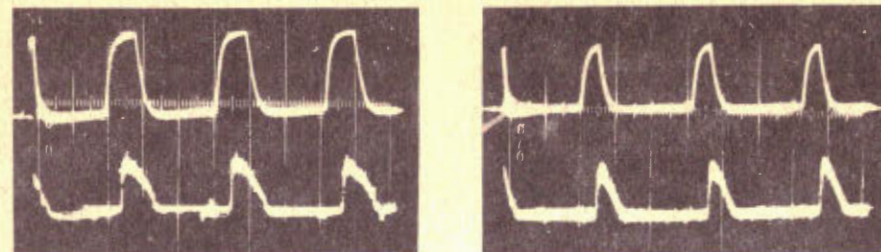
Рис. 5. Осциллограммы импульсов ионного тока /нижние лучи/ и импульсов напряжения на пьезоэлементе. Развертка - 2 мс/дел., масштаб по вертикали - 1 В/дел. /нижние лучи/, 50 В/дел. - верхние лучи.
