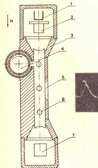
Рис.3. 1 - нить накала, 2 - катод, 3 - разрядная камера, 4 - модулятор, 5 - эмиссионная щель, 6 - фотодиод.
