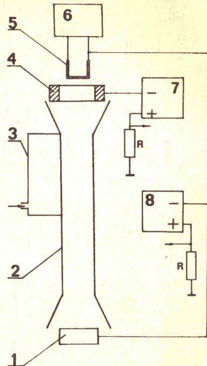
Рис.2. 1 - антикатод, 2 - разрядная камера, 3 - клапан, 4 - коллектор ионов, 5 - нить накала, 6,7,8 - выпрямители.
