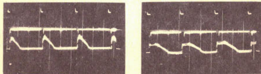
Рис. 6. Осциллограммы импульсов ионного тока /нижние лучи/ и импульсов напряжения на обмотке рамки. Развертка - 2 мс/дел., масштаб по вертикали - 2 В/дел. /нижние лучи/, 1 В/дел. /верхние лучи/.
