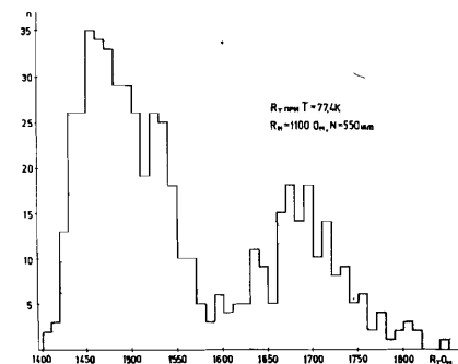
Рис. 11. Гистограмма распределения сопротивления резисторов ТВО ( R_H = 1,1 кОм) в партии 550 шт. при T = 77,4 К.
