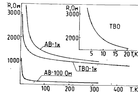
Рис. 3. Зависимость сопротивления R резисторов ТВО ( R_H = 1 кОм) и "Аллен-Бредли" (АВ, R_H = 1 кОм и R_H = 100 Ом) от температуры T .
