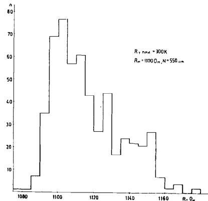
Рис. 12. Гистограмма распределения сопротивления резисторов ТВО ( R_n = 1,1 \text{ кОм} ) в партии 550 шт. при T = 300 \text{ К} .
