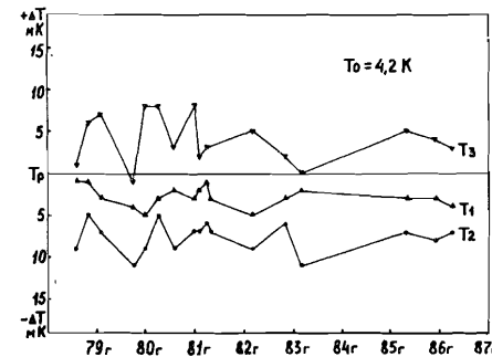
Рис. 4. Относительное отклонение показаний \Delta T 3 контрольных термометров ( T_1 \div T_3 ) в течение 7 лет проверки при температуре 4,2 К.
