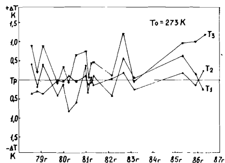
Рис. 6. Относительное отклонение показаний \Delta T 3 контрольных термометров ( T_1 \div T_3 ) в течение 7 лет проверки при температуре 273 К.
