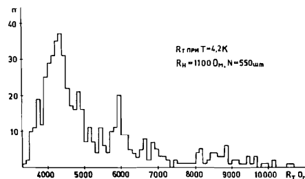
Рис. 10. Гистограмма распределений сопротивления резисторов ТВО ( R_H = 1,1 кОм) в партии 550 шт. при T = 4,2 К.
