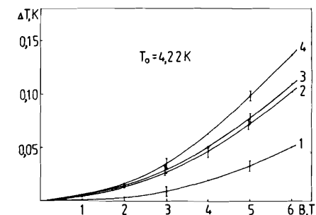
Рис. 7. Зависимость погрешности показаний \Delta T_B от величины магнитного поля B для термометров с различной температурной чувствительностью S_T при T_0 = 4,22 К; 1 - S_T = 570 Ом/К; 2 - S_T = 710 Ом/К; 3 - S_T = 920 Ом/К; 4 - S_T = 1670 Ом/К.
