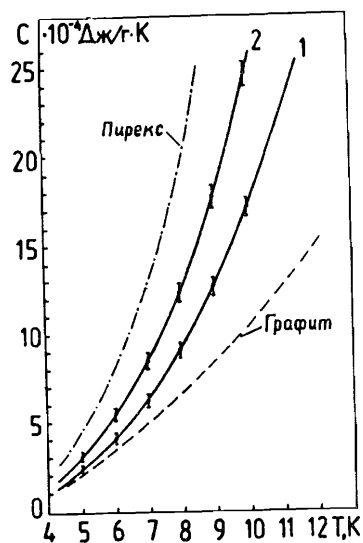
Рис. 9. Зависимость теплоемкости C термометра ТСК от температуры T : 1 – собственная теплоемкость (композит), измеренная по импульсной методике; 2 – полная теплоемкость, измеренная методом термической релаксации.
