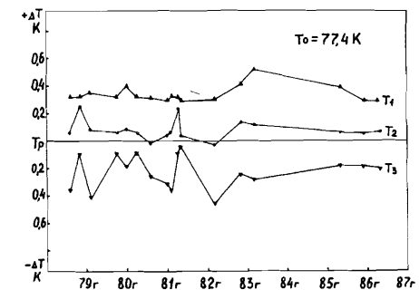
Рис. 5. Относительное отклонение показаний \Delta T 3 контрольных термометров ( T_1 \div T_3 ) в течение 7 лет проверки при температуре 77,4 К.
