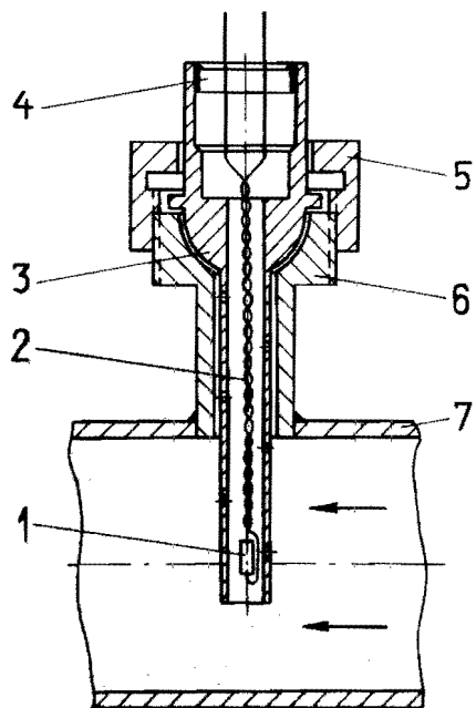
Рис. 14. Конструкция крепления ТСК в гелиевом трубопроводе: 1 – термометр ТСК, 2 – измерительные провода (скрутка 2 МГТФ-0,07), 3 – защитный чехол, 4 – доннышко с выводами, 5 – накидная гайка, 6 – штуцер, 7 – труба.
