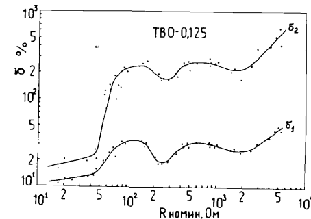
Рис. 2. Зависимость температурных коэффициентов сопротивления \delta_1 и \delta_2 резисторов ТВО-0,125 от номинала R_H ( T_0 = 300 К);
