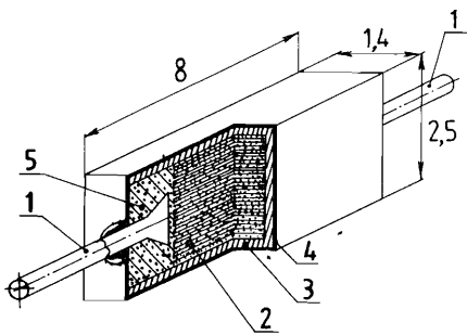
Рис. 1. Конструкция и размеры композиционного резистора ТВО-0,125. 1 – платиновые выводы, 2 – токопроводящая объемная композиция, 3 – керамическая оболочка, 4 – стеклоэмаль, 5 – серебряный порошок.
