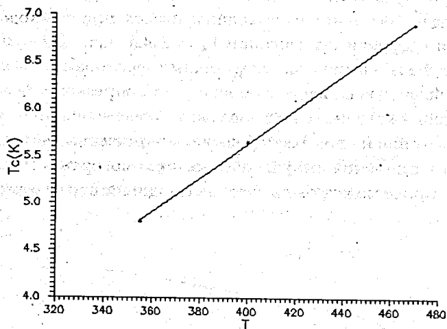
Рис.5. Зависимость температуры T_c (K) перехода в сверхпроводящее состояние пленок Nb толщиной 3,9 нм от температуры подложки T (°C)
