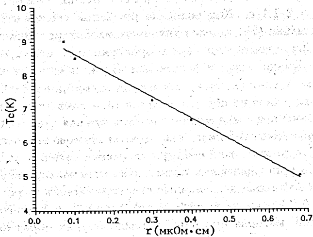
Рис.3. Зависимость температуры T_c перехода в сверхпроводящее состояние Nb пленки от остаточного сопротивления r , измеренного при 10 \text{ K}
