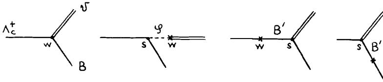
Рис. 3. Процесс распада \Lambda_c^+ \rightarrow 1/2^+ + 1^- .
