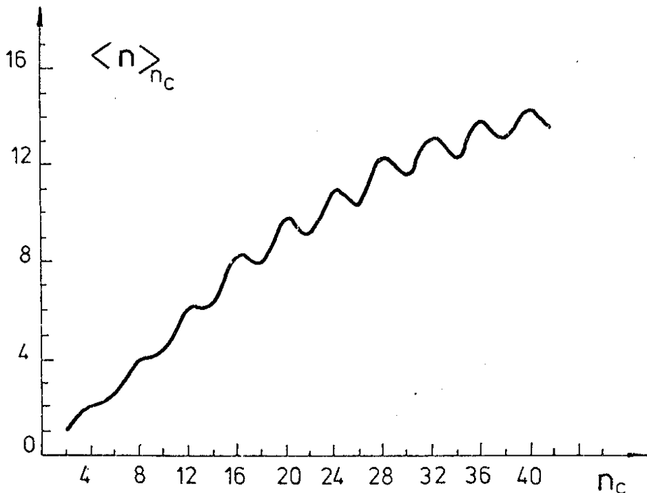
Рис.2. Поведение \langle n \rangle_{n_c} , полученное с использованием формулы /П1/.
