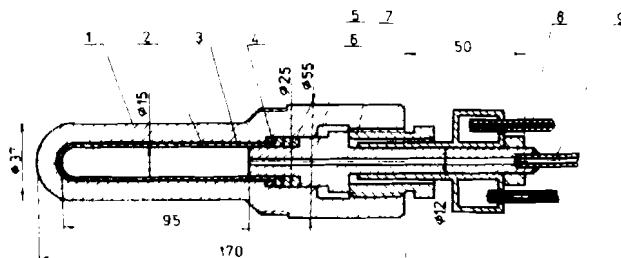
Рис. 1. Чертеж мишени.
