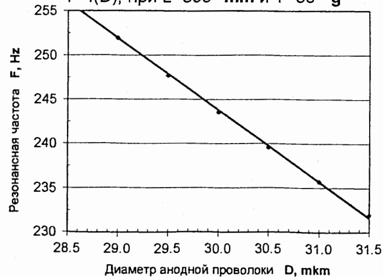
Рис.7. Зависимость резонансной частоты от диаметра анодной проволоки при длине L=393 мм и натяжении T=50 г
