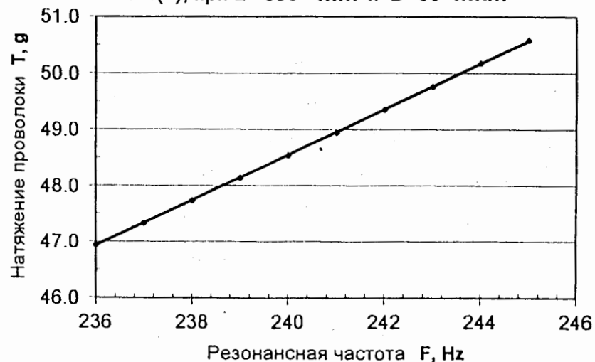
Рис.6. Зависимость натяжения анодной проволоки от резонансной частоты при длине L=393 мм и диаметре D=30 мкм
