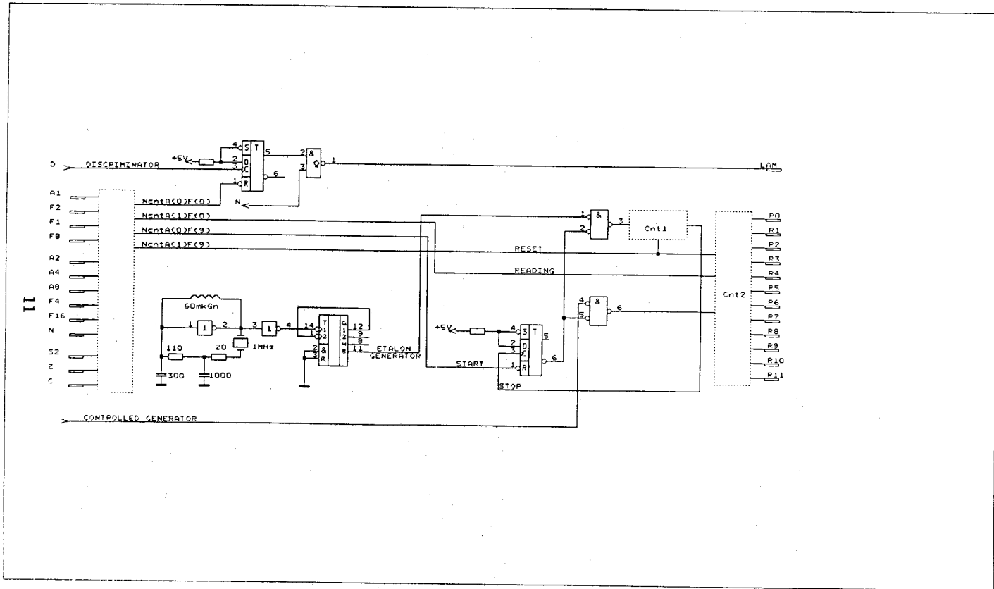
Рис.2. Упрощенная схема частотомера
