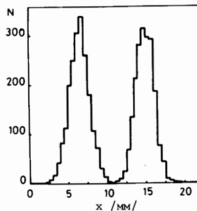
Рис.3. Распределения вычисленных по центру тяжести координат для двух положений светодиода. Ширина коллиматора 0,8 мм.
