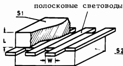
Рис.1. Конструкция сцинтилляционного счетчика.
