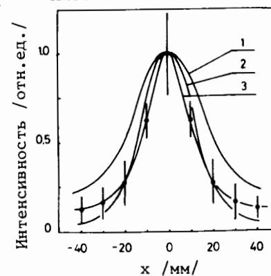
Рис.4. Форма световой вспышки в сцинтилляторе от различных источников. Кривая 1 - радиоактивный источник ^{106}\text{Ru} , кривая 2 - светодиод, кривая 3 - частицы космического излучения.
