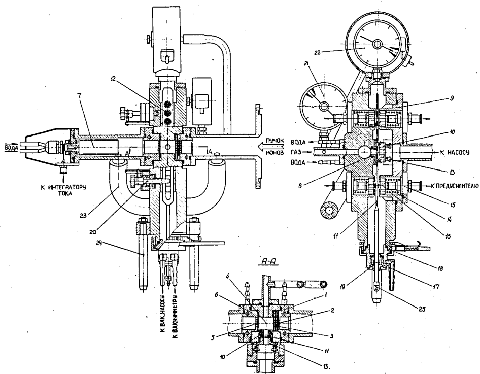
Рис. III. Реакционная камера и камера со сборниками и детекторами. 1 - входная решетка, 2 - входная фольга, 3 - мишень, 4 - реакционная камера, 5 - выходная решетка, 6 - выходная фольга, 7 - цилиндр Фарадея, 8 - корпус, 9 - крышка, 10 - бужа уплотнительная, 11 - рейка-держатель фильтров, 12 - фильтр-сборник, 13 - прижимная каретка, 14 - детектор, 15 - разъем вакуумный, 16 - пружина, 17 - шлюз, 18 - быстродействующий зажим, 19 - уплотнительная втулка, 20 - устройство для калибровки детектора, 21 - электроконтактный вакуумметр, 22 - дифференциальный вакуумметр, 23 - шланг для откачки объема с цилиндром Фарадея, 24 - направляющая, 25 - серьга для соединения с пневмоприводом.
