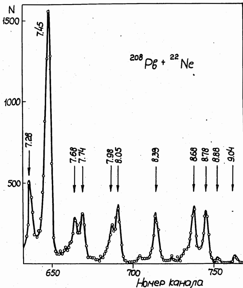
Рис. VIII . Амплитудный спектр \alpha -частиц продуктов реакций \text{Pb}^{208} + \text{Ne}^{22} . Время движения сборника равно 0,045 сек, время стоянки - 0,850 сек.
