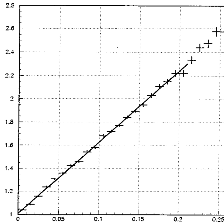
Рис. 6: Зависимость средней ширины кластера от ctg \gamma для моделированных событий
