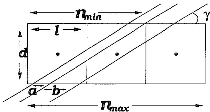
Рис. 1: Проекция трека на плоскость, перпендикулярную всем сигнальным проволочкам
