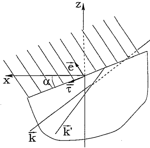
Рис. 3: Прохождение трека \vec{k} через ПК и плоскость, содержащую ось Z и вектор \vec{r}
