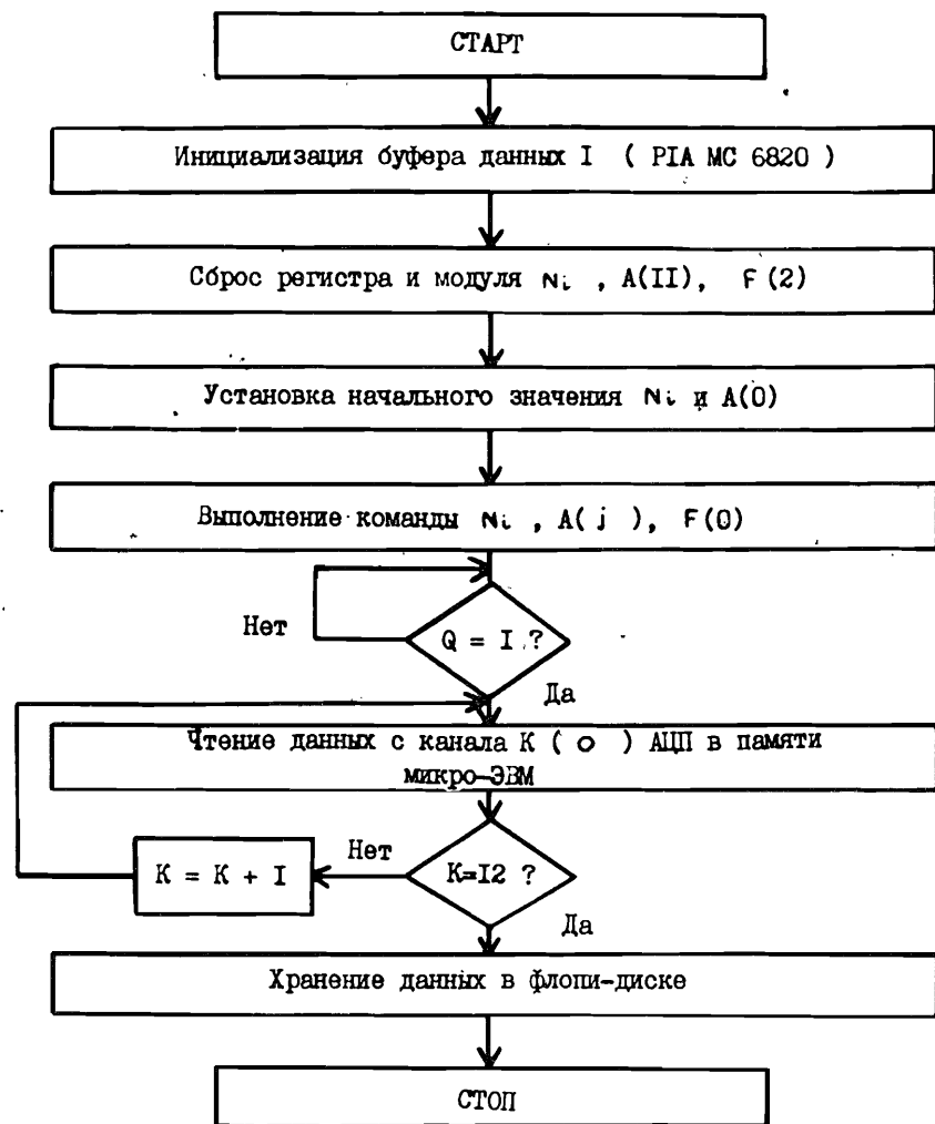
Рис.2. Алгоритм программы чтения информации с АЦП 2249А.
