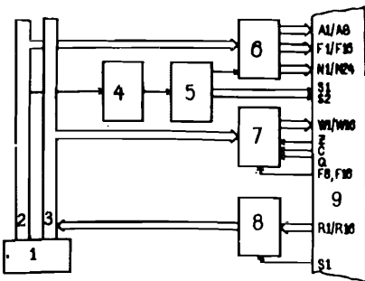
Рис.1. Блок-схема интерфейса КАМАК с микро-ЭВМ. 1 - микро-ЭВМ М6800; 2 - адресная шина; 3 - шина данных; 4 - дешифратор опроса КАМАК; 5 - блок таймера; 6 - буфер команд КАМАК /БК/; 7 - буфер данных I /БДИ/; 8 - буфер данных II /БДИИ/; 9 - магистраль КАМАК.
