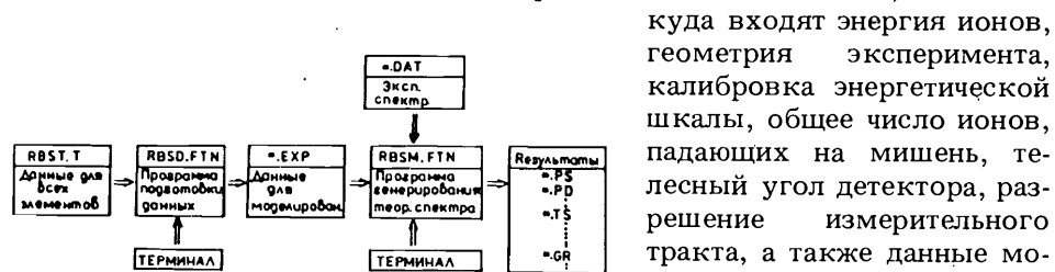
Рис. 1. Общая схема компьютерной обработки спектров упруго рассеянных ионов.
