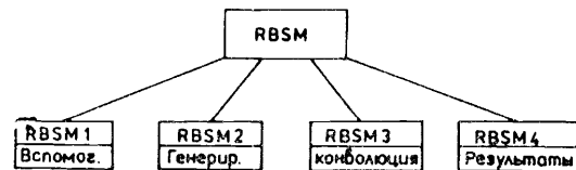
Рис. 2. Структура программы RSBM.
