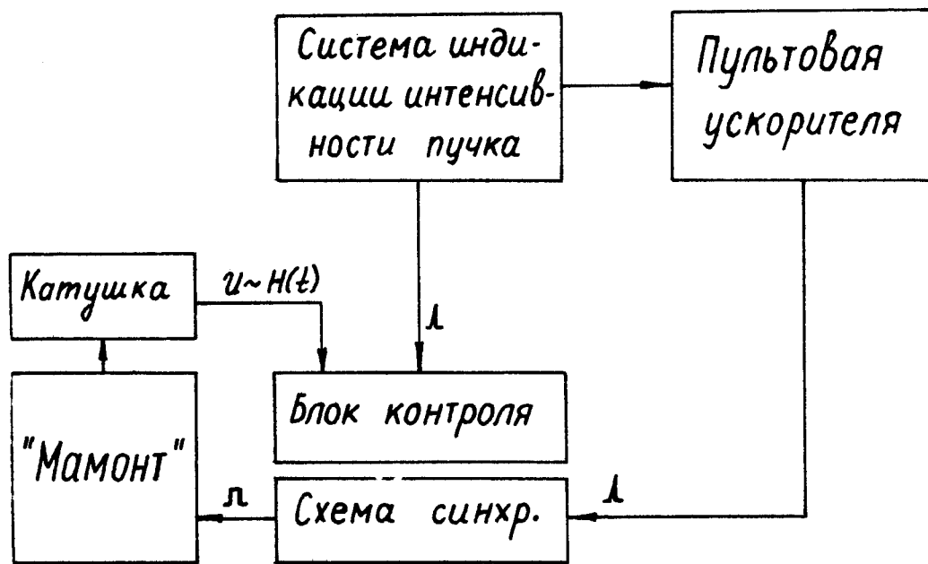
Рис. 4. Блок-схема установки "Мамонт".
