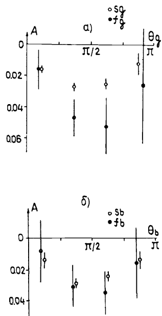
Рис. 5 Зависимости A_{sq} и A_{fg} от \theta_g (а) и A_{sb} и A_{fb} от \theta_b (б) для ^{22}\text{Ne}-E_m событий.
