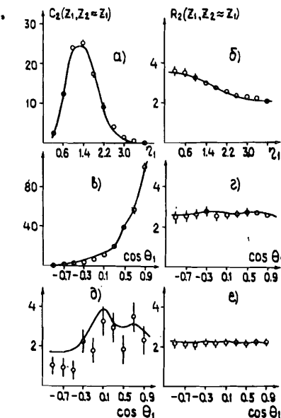
Рис. 1 Зависимости корреляционных функций C_2 (а, в, д) и R_2 (б, в, е.) при z_2 = z_1 от z_1 для s (а, б), g (в, в) и b (д, е) частиц из ^{22}\text{Ne} - \text{Em} взаимодействий.
