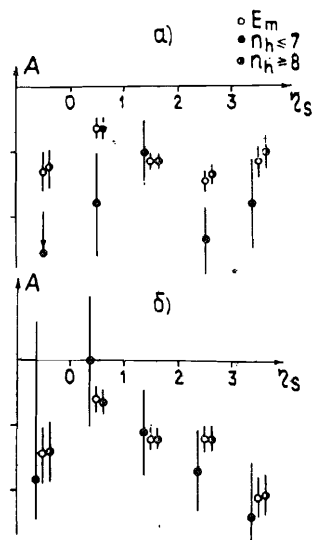
Рис. 6 Зависимости A_{sq} (а) и A_{sb} (б) от \eta_s для соударений ^{22}\text{Ne}-E_m и подгрупп с n_h \leq 7 и n_h \geq 8 .
