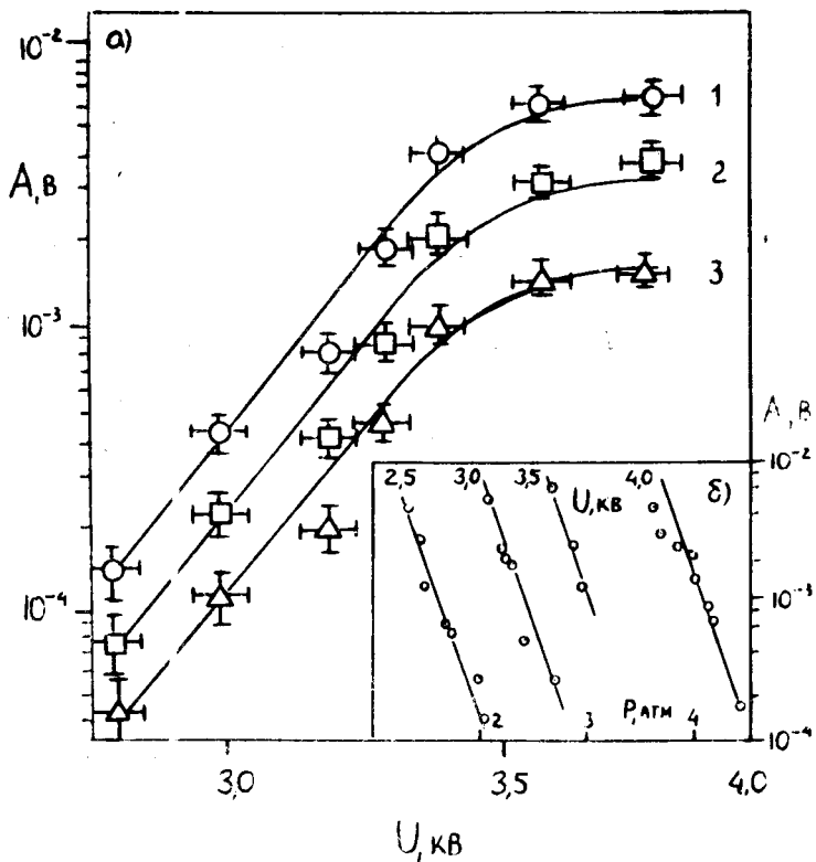
Рис. 6. а) Зависимость амплитуды сигнала A от напряжения U при различной поглощенной энергии E : 1-2 Мэв, 2-1 Мэв, 3-0,5 Мэв. Давление p = 3, 3 атм.. б) Зависимость A от давления P при различных рабочих напряжениях U . Поглощенная энергия E = 0,5 Мэв. Нить 100 мкм, ток накала 0,3 а.
