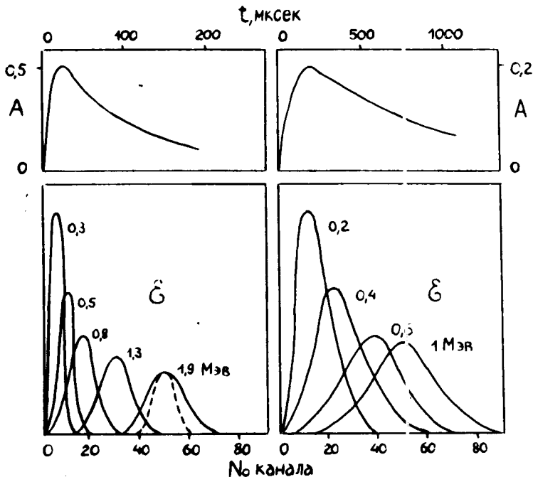
Рис. 4. Типичные осциллограммы сигналов и амплитудные спектры сигналов в детекторе с регистрирующей нитью, помещенной над поверхностью жидкого аргона (слева, нить 100 мкм) и под поверхностью жидкого аргона (справа, нить 30 мкм). Пунктиром показан амплитудный спектр сигналов при поглощенной энергии около 1 Гэв без газового усиления вблизи поверхности нити. Ионизация рентгеновскими лучами. Амплитуда сигналов A на верхних рисунках - в относит. ед. (за единицу принята амплитуда сигнала при полном собирании электронов на емкости 300 пф).
