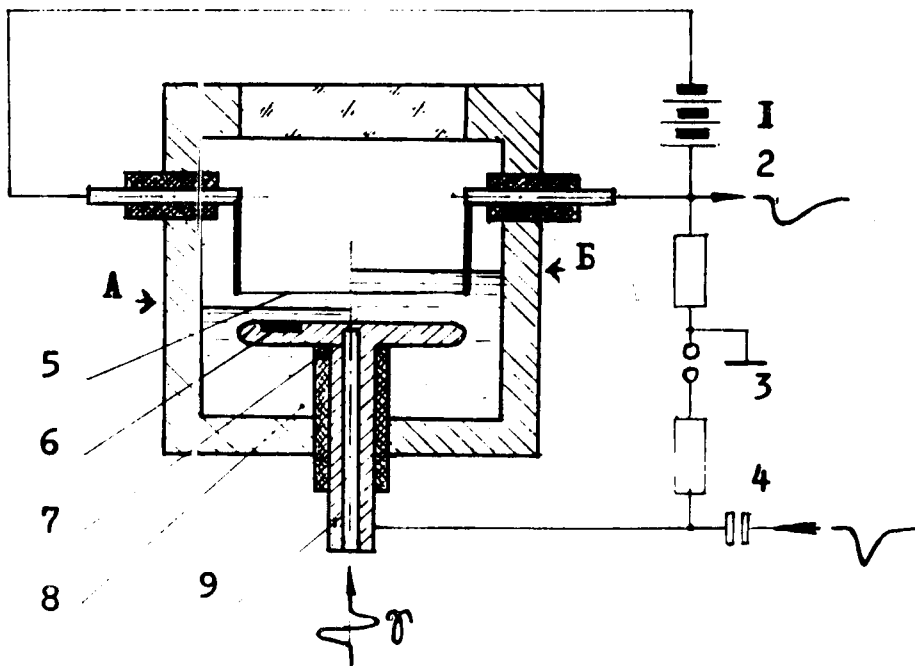
Рис. 2. Исследовательская камера. А - вариант детектора с нитью, расположенной над поверхностью жидкого аргона; Б - вариант детектора с прогреваемой нитью, погруженной в жидкий аргон. 1 - батарея аккумуляторов, обеспечивающая прогрев нити; 2 - выход сигнала; 3 - ввод высокого напряжения; 4 - ввод высоковольтного импульса при исследовании импульсного режима работы детектора (вариант В); 5 - проволочный анод; 6 - \alpha -источник; 7 - изолятор; 8 - жидкий аргон; 9 - коллиматор.
