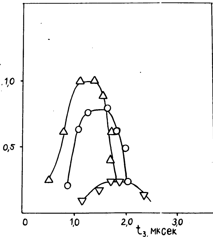
Рис. 3. Зависимость амплитуды добавочной вспышки электролюминесценции от времени задержки подачи высоковольтного импульса в камеру ( T - 108^\circ ). Совершенно идентичные кривые наблюдались для всех температур от 94^\circ\text{K} до 120^\circ\text{K} . \nabla E/p = 1,6 ; \circ E/p = 2,0 ; \Delta E/p = 2,7 ; E - суммарная напряженность постоянного и импульсного электрических полей, в/см; p - давление, мм. рт. ст.
