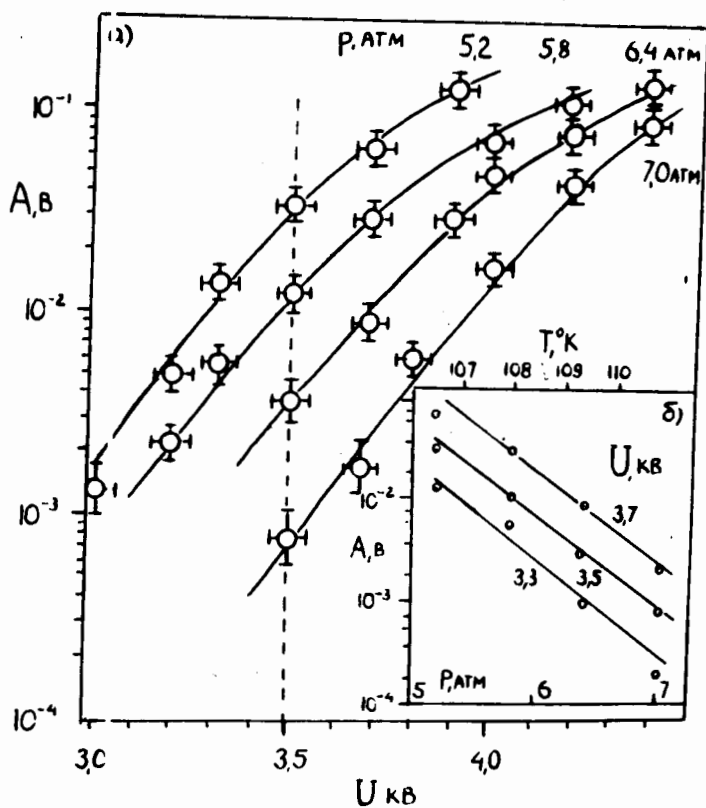
Рис. 10. а) Зависимость амплитуды сигнала A от напряжения U при различных давлениях P внутри камеры. б) Зависимость амплитуды сигнала A от давления внутри камеры P при различных напряжениях на камере U . Нить 100 мкм, ток накала 0,3 а, E = 1 МэВ.
