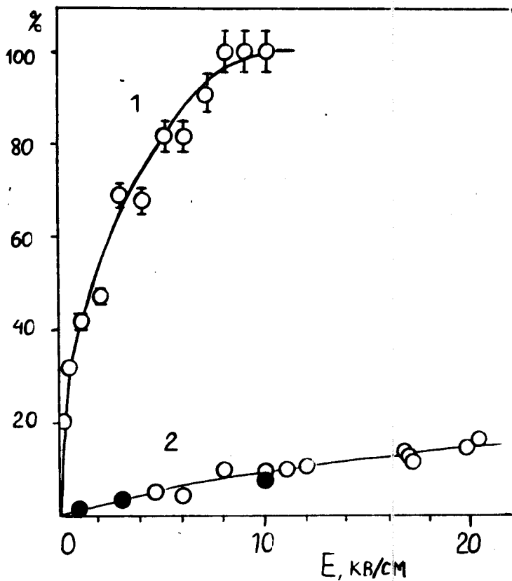
Рис. 1. Относительный выход электронов с трека рентгеновского фотоэлектрона (1) и \alpha -частицы (2) в зависимости от напряженности электрического поля в жидком аргоне. На кривой 2 светлыми кружками - результаты ионизационных измерений в жидком аргоне (16).
