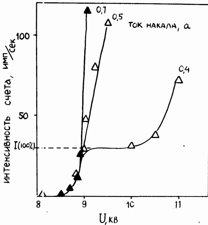
Рис. 7. Счетная характеристика детектора, регистрирующего \alpha -частицы для различных токов накала проволоки. В используемых электрических полях с трека \alpha -частицы вытягивается \sim 6 \cdot 10^3 электронов (эквивалентные потери энергии для релятивистской частицы \sim 150 кэВ). При токе накала 0,5 а счет отсутствует вплоть до напряжения 15 кв. Нить 100 мкм, давление 4,6 атм. I(100\%) - интенсивность счета при 100%-ной эффективности регистрации \alpha -частиц.
