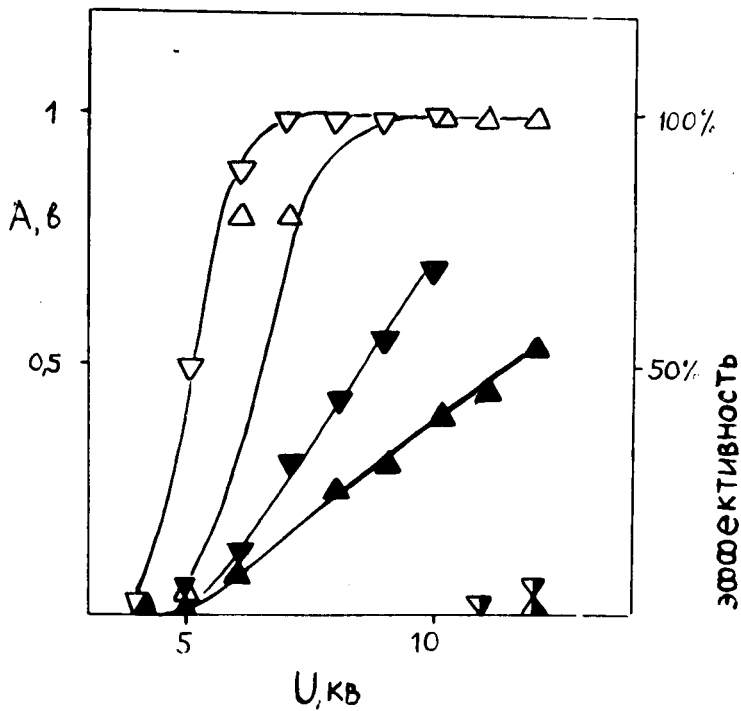
Рис. 11. Зависимость амплитуды сигнала A ( \blacktriangle , \triangledown ); эффективности регистрации рентгеновских лучей и интенсивности шумов ( \triangle , \triangledown и \blacktriangle , \blacktriangledown в %, шкала справа) от импульсного напряжения U , кВ. Ток накала: \blacktriangle , \triangle , \blacktriangledown - 0,5 а; \triangledown , \triangledown , \blacktriangledown - 0,7 а. E = 1 МэВ, T = 108^\circ\text{К} .
