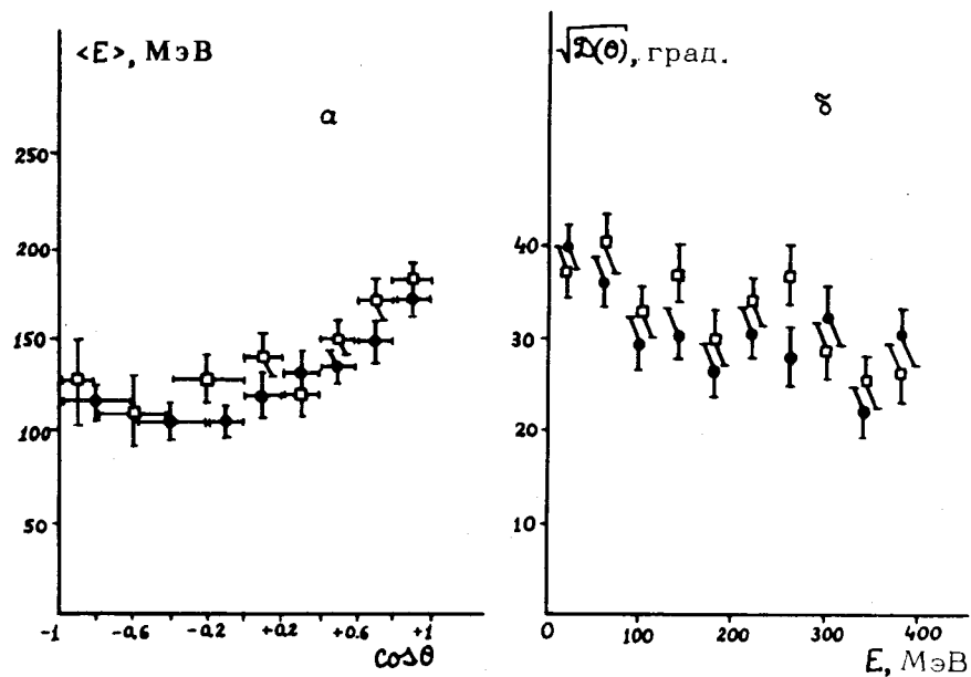
Рис.3. а/ Зависимость средней энергии g -протонов от угла испускания. \square - взаимодействия с N_h \geq 28 , \bullet - взаимодействия с N_h \geq 28 .
