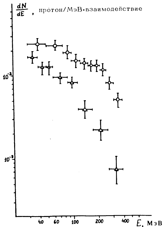
Рис.2. Энергетическое распределение протонов в диапазоне 30-400 МэВ, испущенных: o - в переднюю полусферу /0-90°, Δ - в заднюю полусферу /90-180°/.
