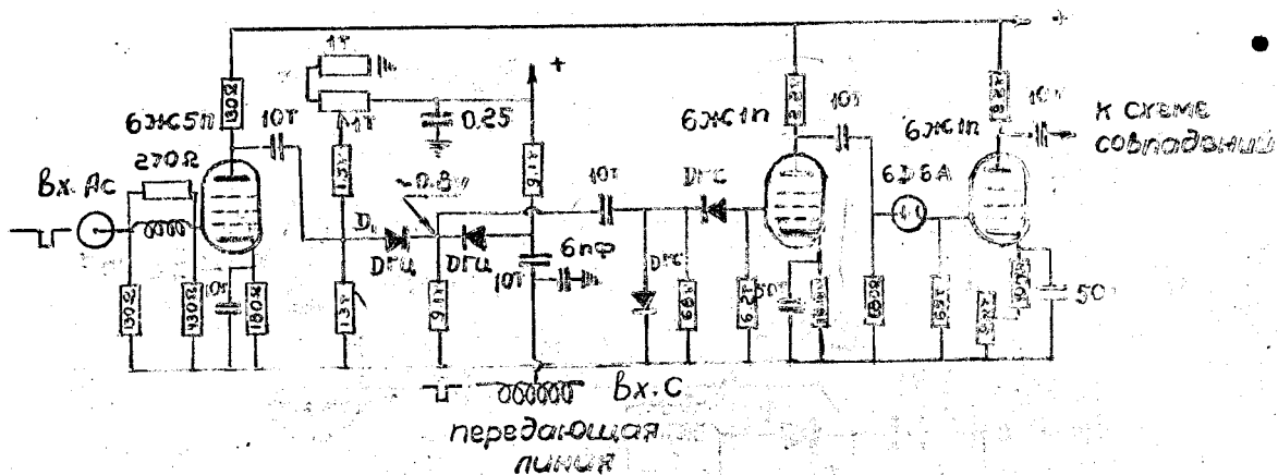
Рис. 8 Схема антисовпадений.
