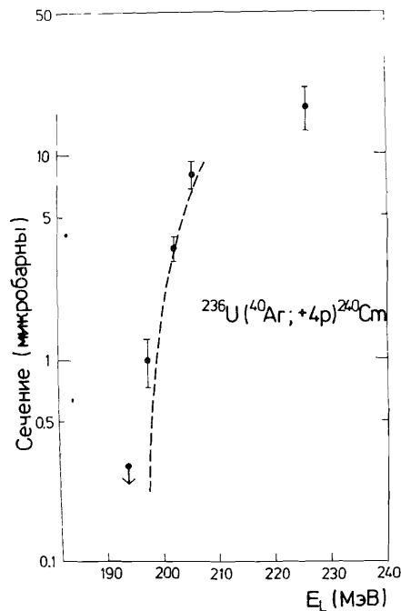
Рис.7. Зависимость сечения образования ядер ^{240}\text{Cm} от энергии ионов в реакции ^{236}\text{U} + ^{40}\text{Ar} . Пунктирная кривая проведена через экспериментальные точки с поправкой на толщину мишенного слоя.
