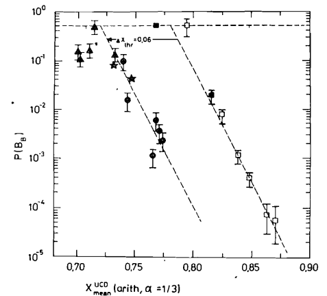
Рис. 3. Зависимость вероятности полного слияния ядер от параметра \chi_{mean}^{UCD} (\alpha=1/3) / 10 . Квадраты - данные опытов по "холодному" слиянию; треугольники, точки, звездочки - другие реакции, протекающие с образованием "горячего" компаунд-ядра.
