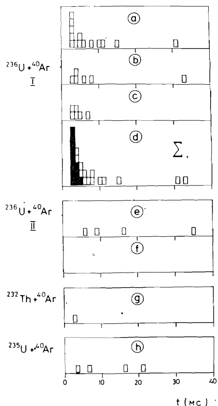
Рис. 11. Временные распределения событий спонтанного деления в интервале от 2 до 38 мс.
