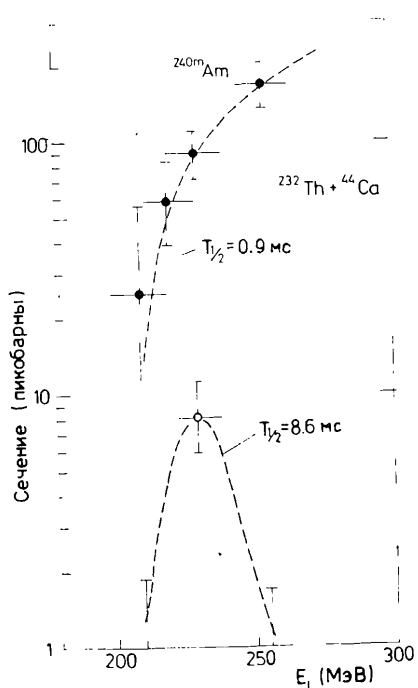
Рис. 4. Сечение образования ^{240m}\text{Am} ( T_{1/2} = 0,9 мс) и активности спонтанного деления с T_{1/2} \sim 8,6 мс в реакции ^{232}\text{Th} + ^{44}\text{Ca} в зависимости от энергии ионов ^{44}\text{Ca} . Пунктирные кривые проведены через экспериментальные точки для наглядности.
