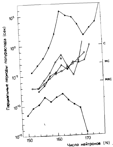
Рис. 14. Расчетные парциальные периоды \alpha -распада (открытые символы) и спонтанного деления (черные символы) изотопов 110 элемента. Точки - данные работы Г.А.Леандера и др. /13/, треугольники - К.Бёнига и др. /24/, открытые квадраты - расчеты Н.Н.Колесникова и А.Г.Демина. Крестиком показано значение периода полураспада для N=162 , полученное в настоящей работе.
