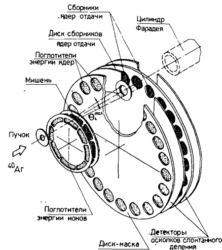
Рис. 5. Схема установки.
