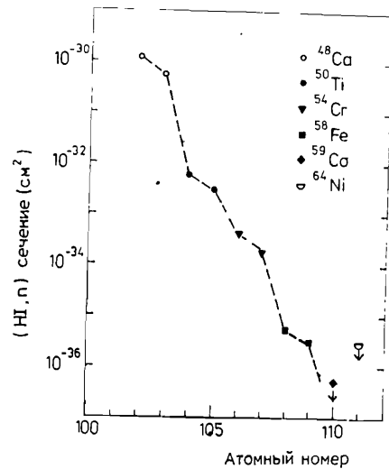
Рис. 2. Зависимость сечения реакции (HI, n) от атомного номера компаунд-ядра при облучении мишеней 208 Pb и 209 Bi различными ионами (указаны на рисунке).
