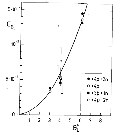
Рис.8. Зависимость эффективности сбора ядер ^{242}\text{Am} , ^{240,242}\text{Cm} от \theta_L в реакциях: ^{236}\text{U} + ^{40}\text{Ar} (206 МэВ) - точки; ^{238}\text{U} + ^{40}\text{Ar} (206 МэВ) - квадраты; кривая - \epsilon(\theta_L) \sim \theta_L^2 .
