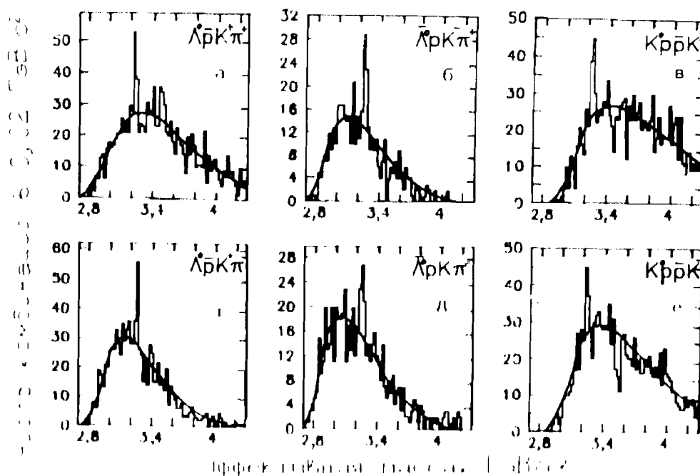
Рис. 2. Спектры инвариантных масс систем: а - \Lambda\bar{p}K^+\pi^+ , б - \bar{\Lambda}pK^-\pi^- , в - K_s^0 p\bar{p}K^+ , г - \Lambda\bar{p}K^+\pi^- , д - \bar{\Lambda}pK^-\pi^+ , е - K_s^0 p\bar{p}K^- .
