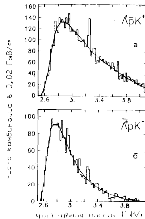
Рис. 2. Спектры инвариантных масс систем: а - \Lambda\bar{p}K^+\pi^+ , б - \bar{\Lambda}pK^-\pi^- , в - K_s^0 p\bar{p}K^+ , г - \Lambda\bar{p}K^+\pi^- , д - \bar{\Lambda}pK^-\pi^+ , е - K_s^0 p\bar{p}K^- .
