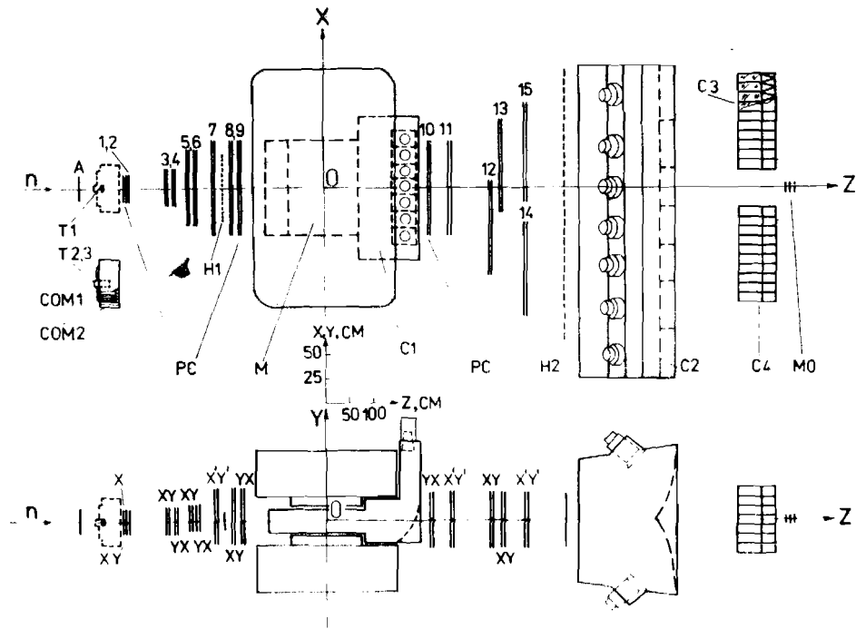
Рис. 1. Схема расположения основных элементов спектрометра БИС-2: Т1/Т2,3 - мишени; СОМ1/2 - счетчики окружения мишени; РС 1-15 - двухкоординатные пропорциональные камеры; С1/2 - многоканальные пороговые газовые черенковские счетчики (МПЧС1/2); С3/4 - черенковские счетчики полного поглощения; МО - нейтронный монитор; М - спектрометрический магнит.
