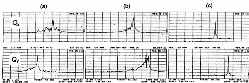
Рис. 2. Пример измерения спектров горизонтальных ( Q_x ) и вертикальных ( Q_y ) бетатронных колебаний. (а) начальная настройка при выключенных соленоидах секции охлаждения, (б) соленоиды секции охлаждения включены и орбита протонного пучка настроена для охлаждения. Спектр охлажденного пучка (с) существенно уже из-за меньшего разброса по импульсу. Полный размах графика по оси частот от 3.500 до 3.700, бетатронные частоты охлажденного пучка Q_x = 3.615 и Q_y = 3.648 .
