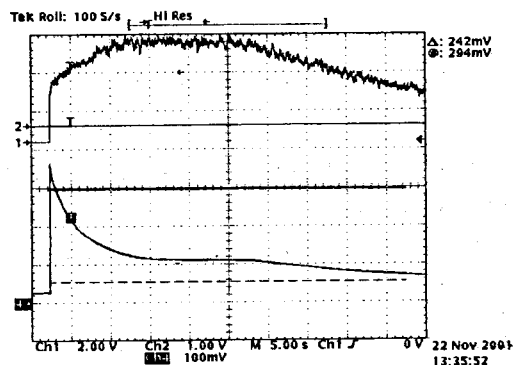
Рис. 1. Изменение во времени тока протонного пучка (нижняя кривая) и скорости счёта нейтральных атомов (верхняя кривая) при однократной инжекции. Масштаб по оси времени – 5 с/деление, ток протонов 100 мВ/деление \approx 1.25 \cdot 10^{10} протонов, темп счёта N^0 1 В/деление = 3000 Гц..
